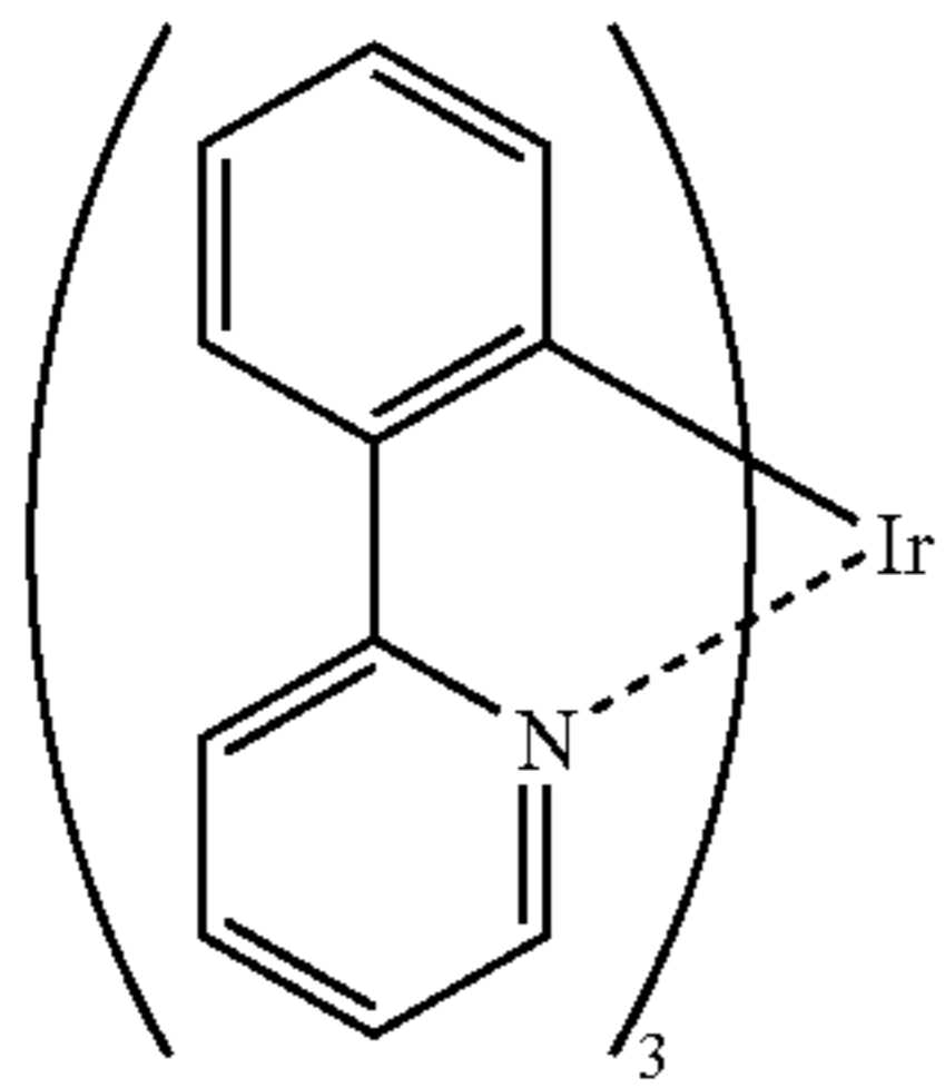
Ir(ppy) 3
