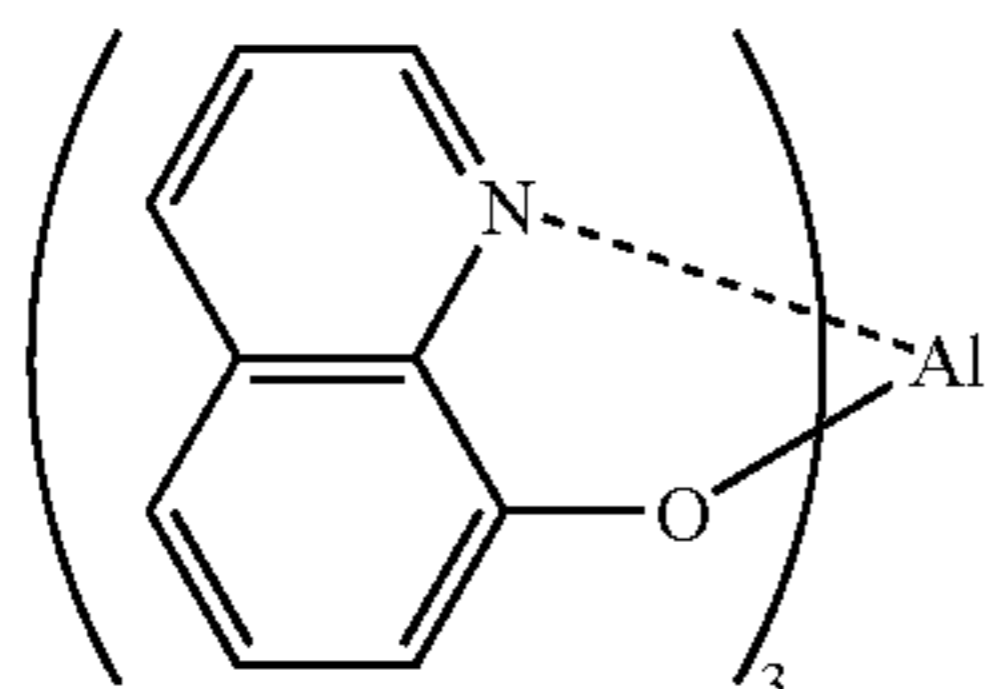
Alq
