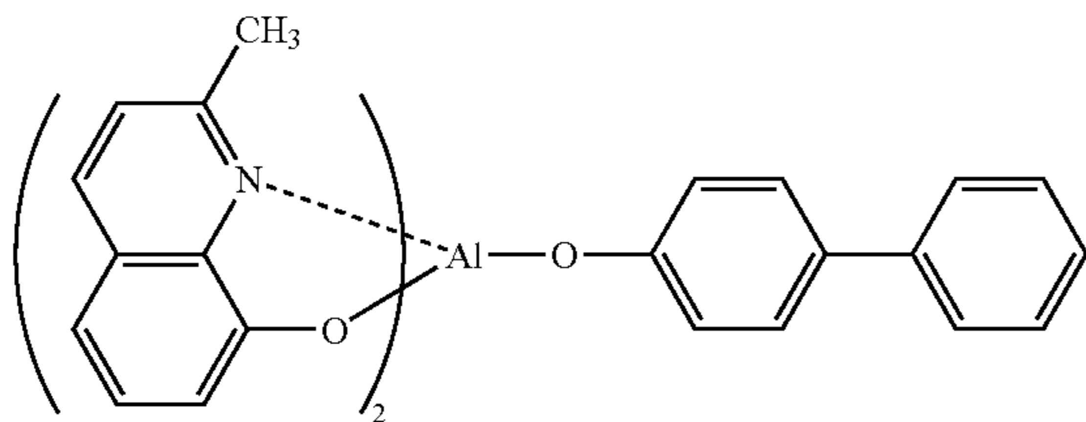
Balq
