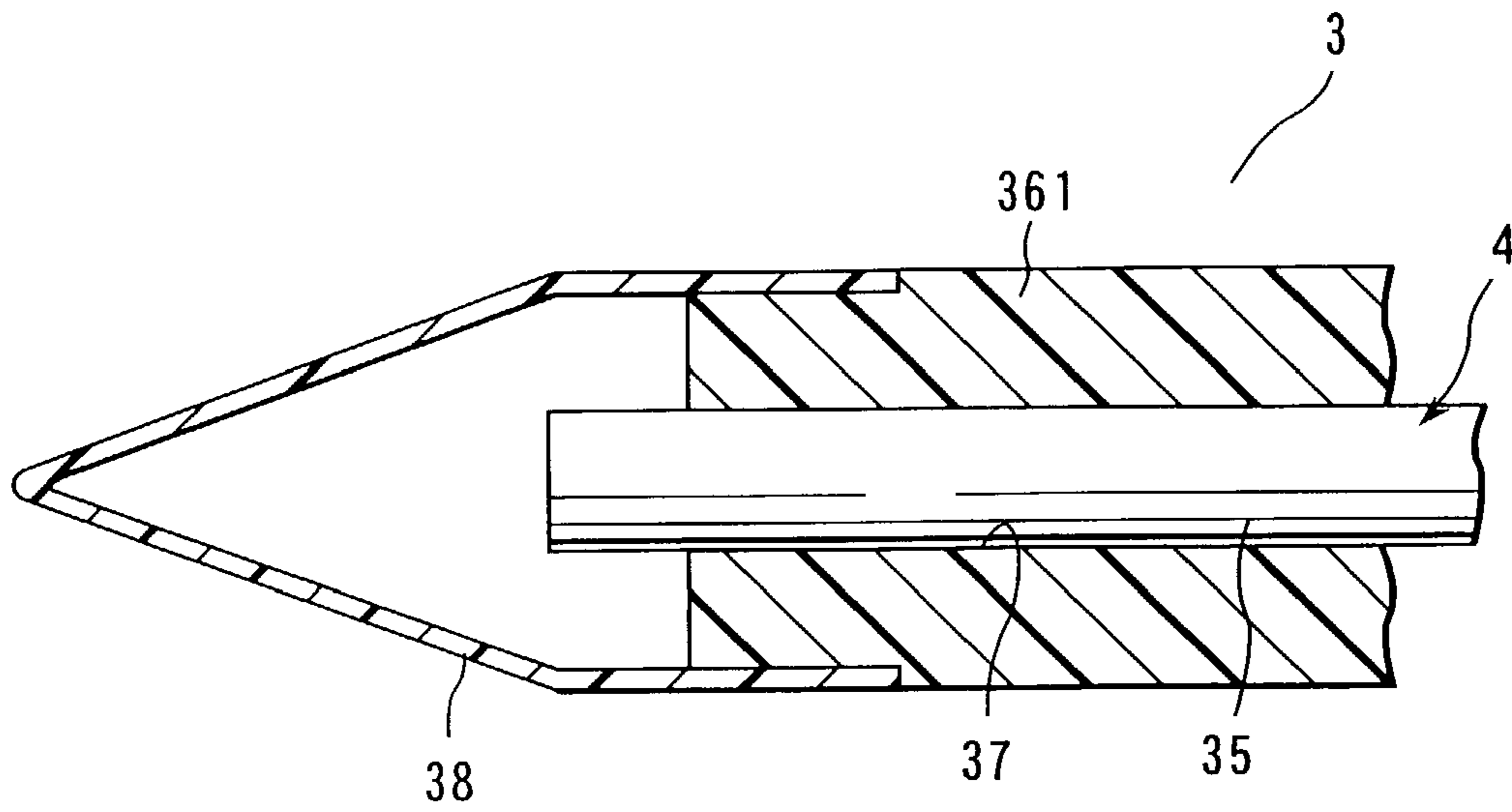
FIG. 4E
