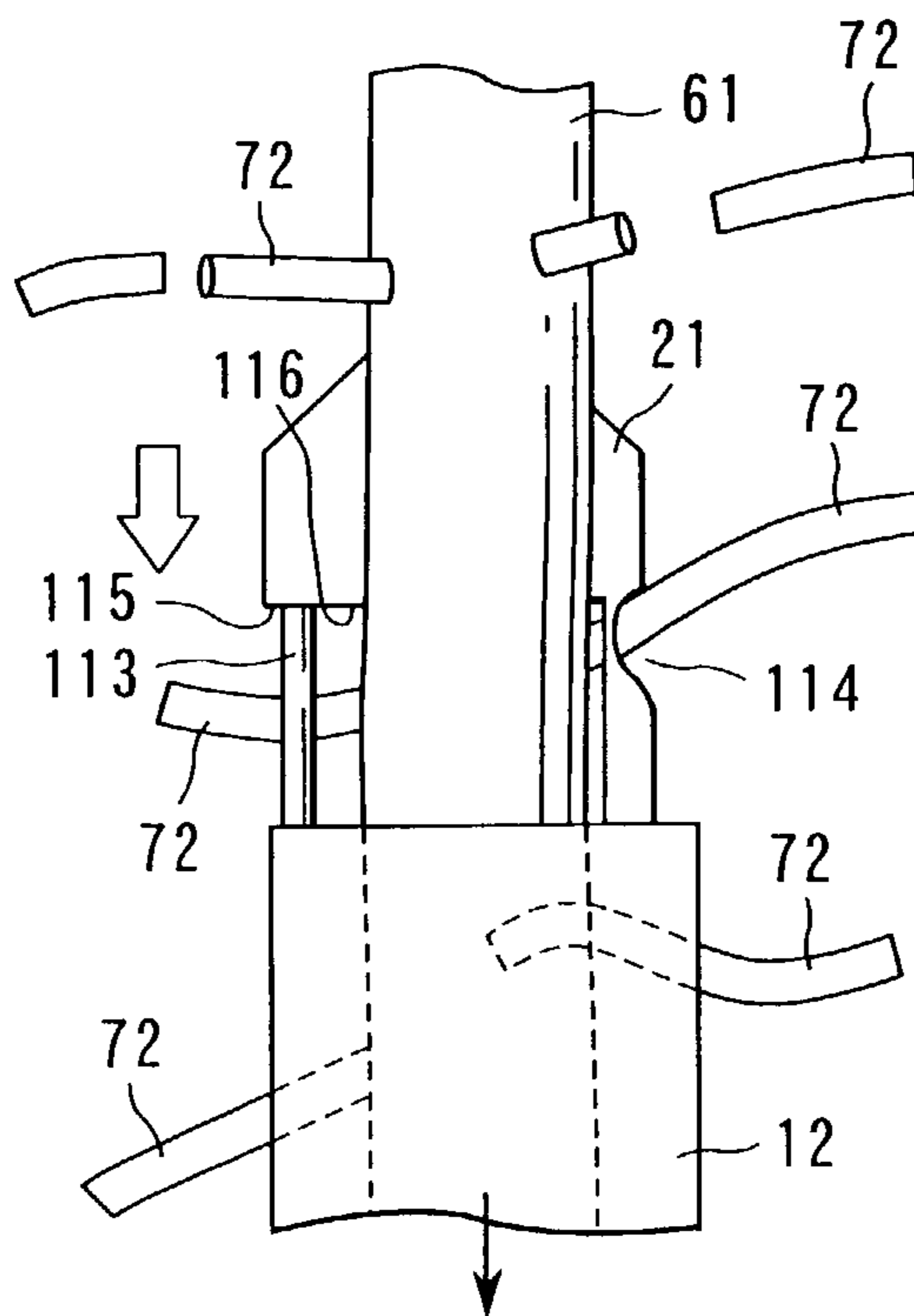
FIG. 34
