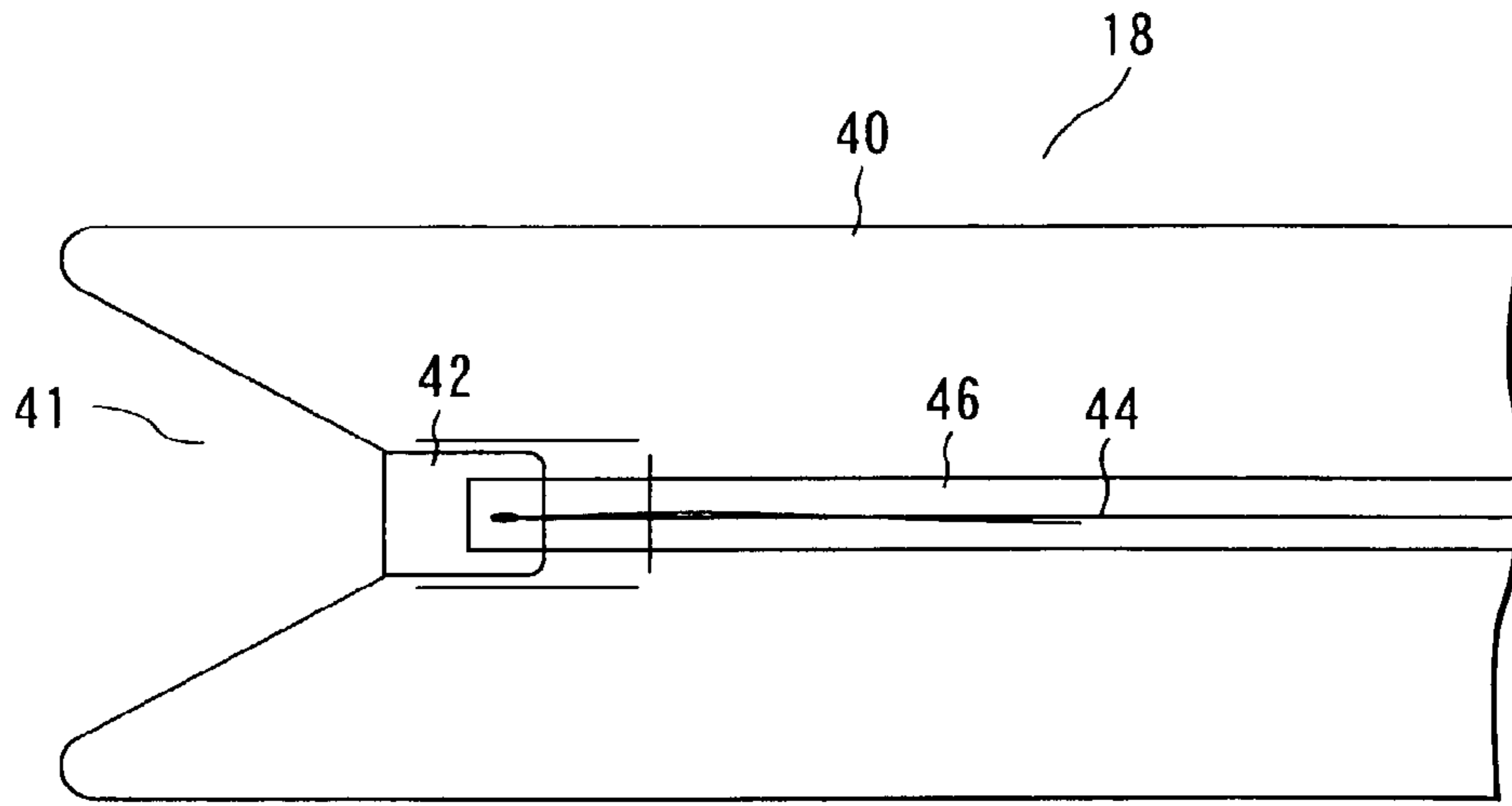
FIG. 5A
