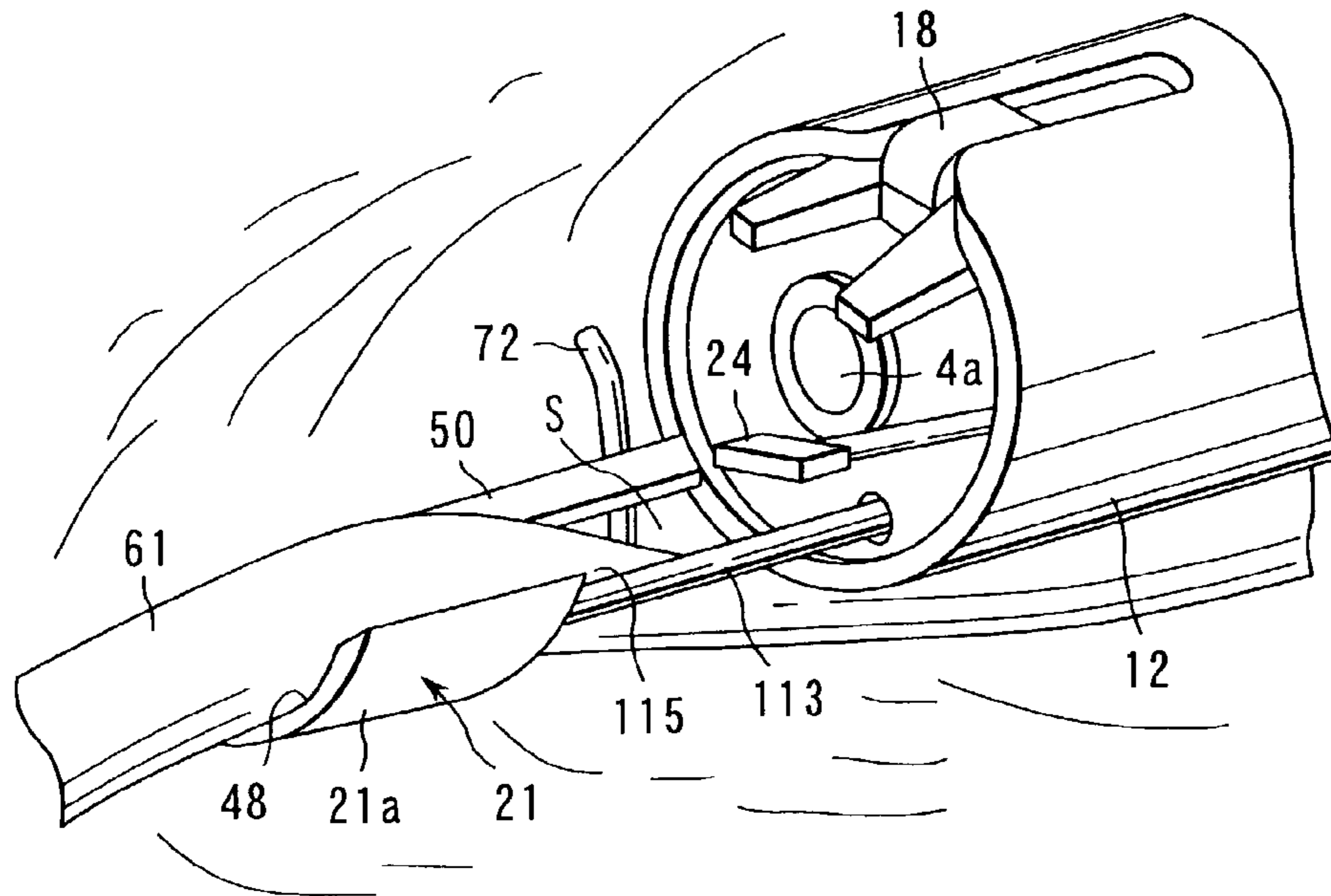
FIG. 29
