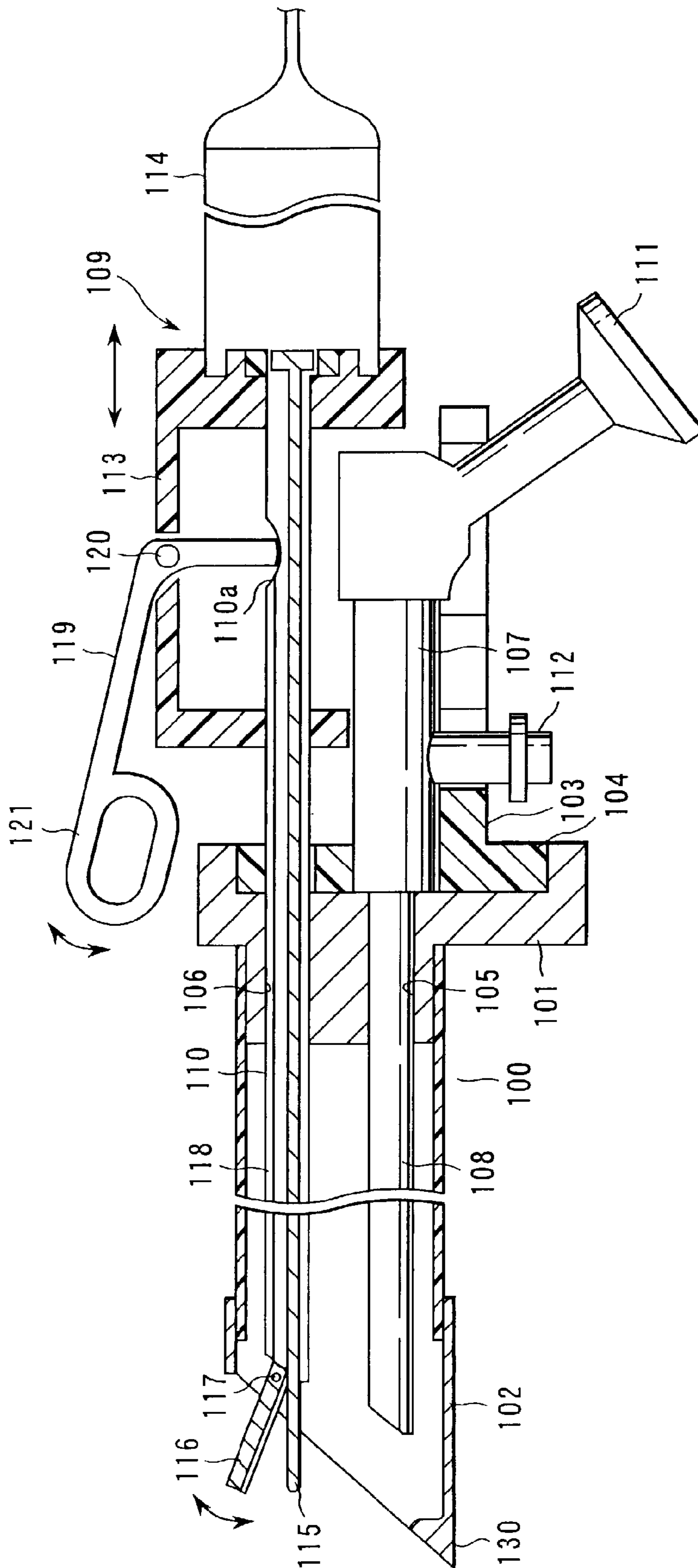
FIG. 36
