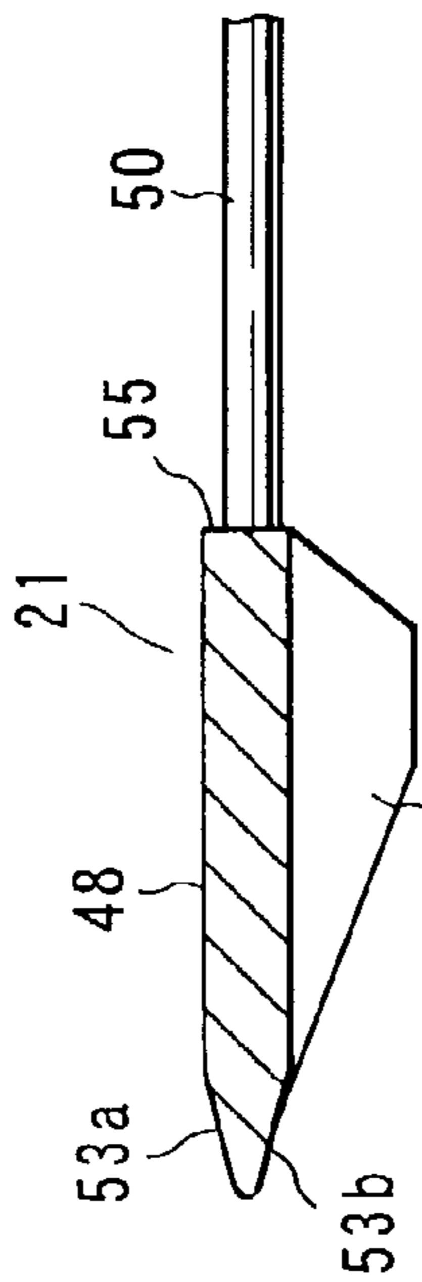
FIG. 6B
