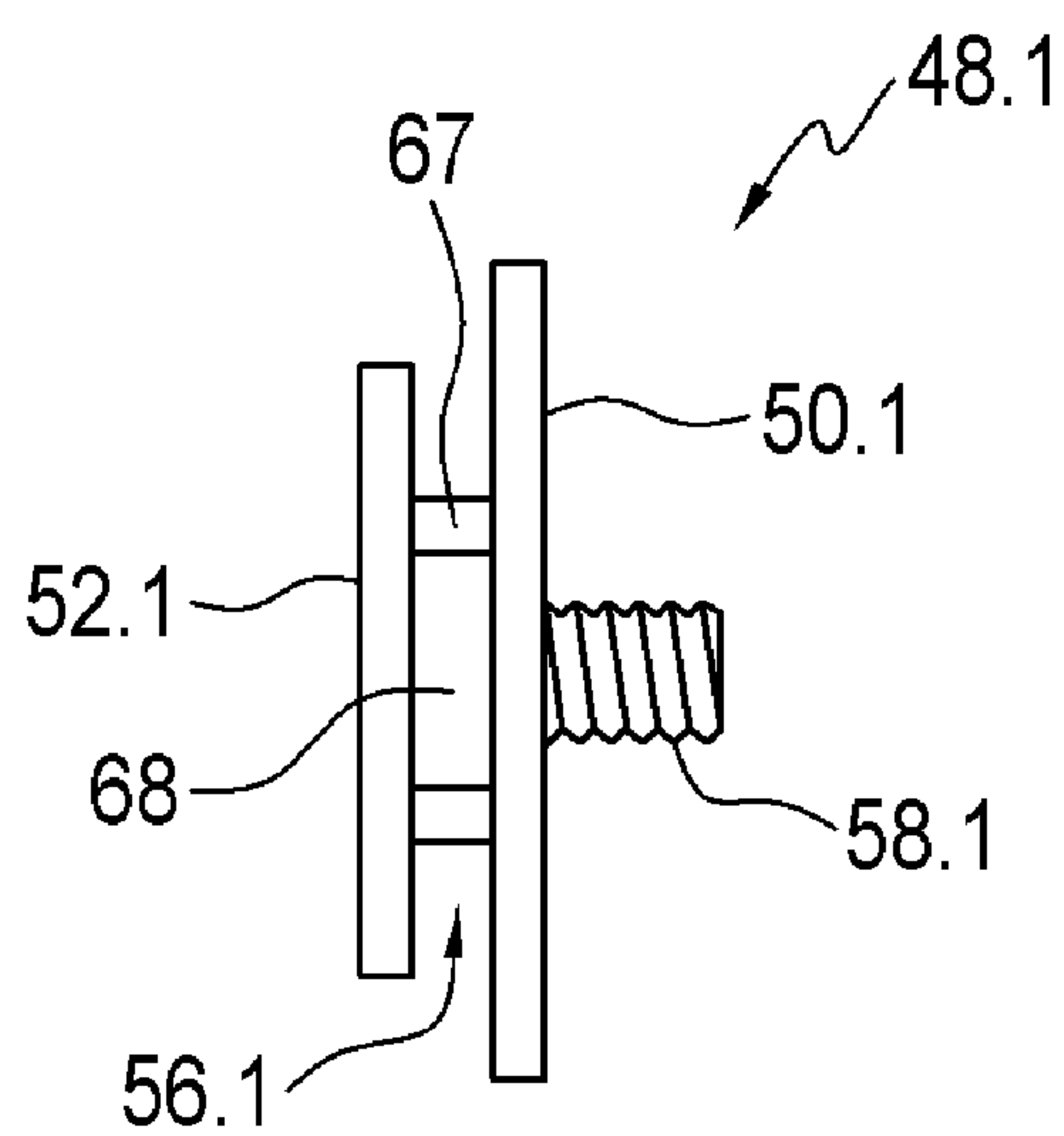
FIG. 16
