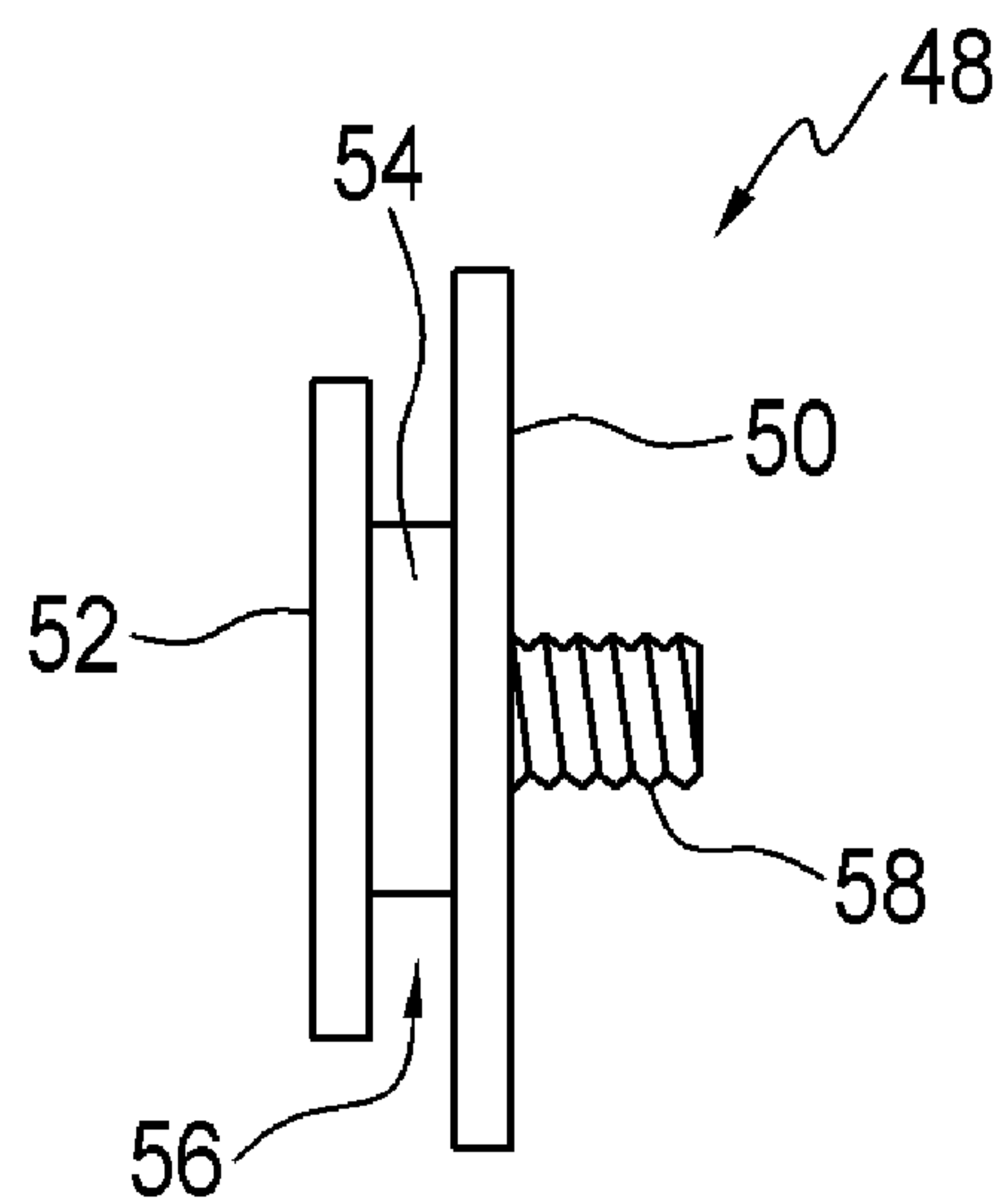
FIG. 10
