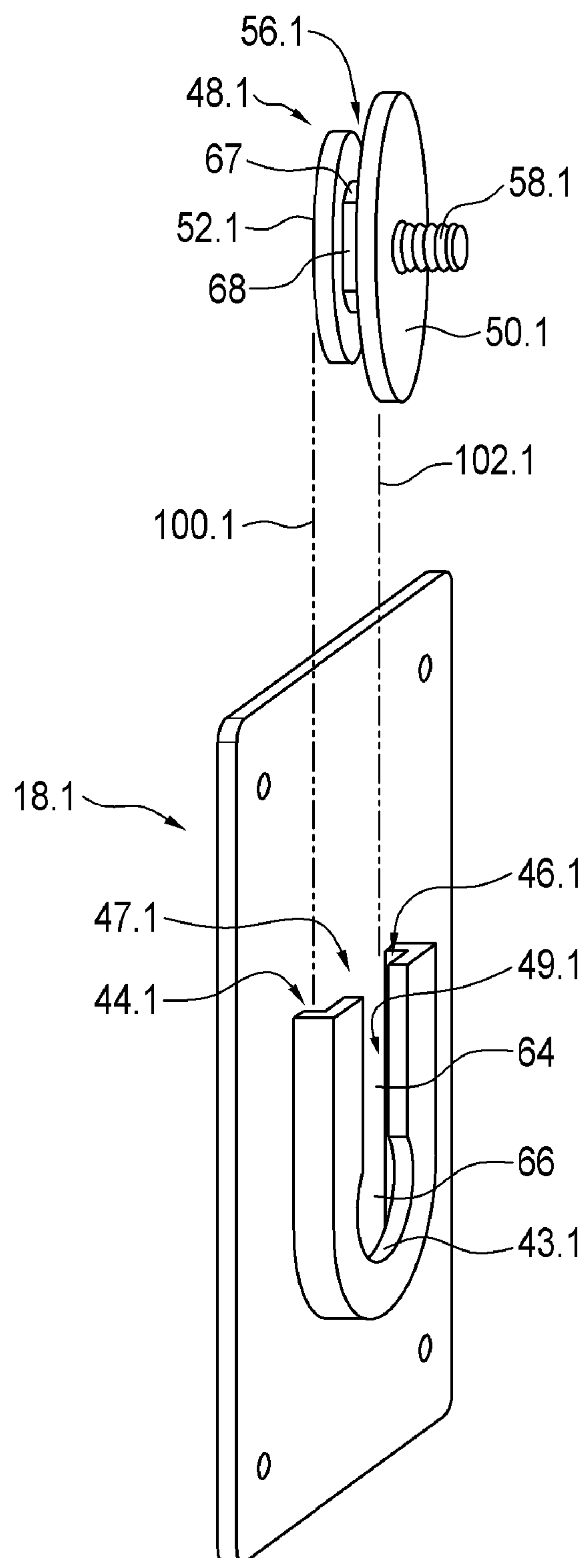
FIG. 17
