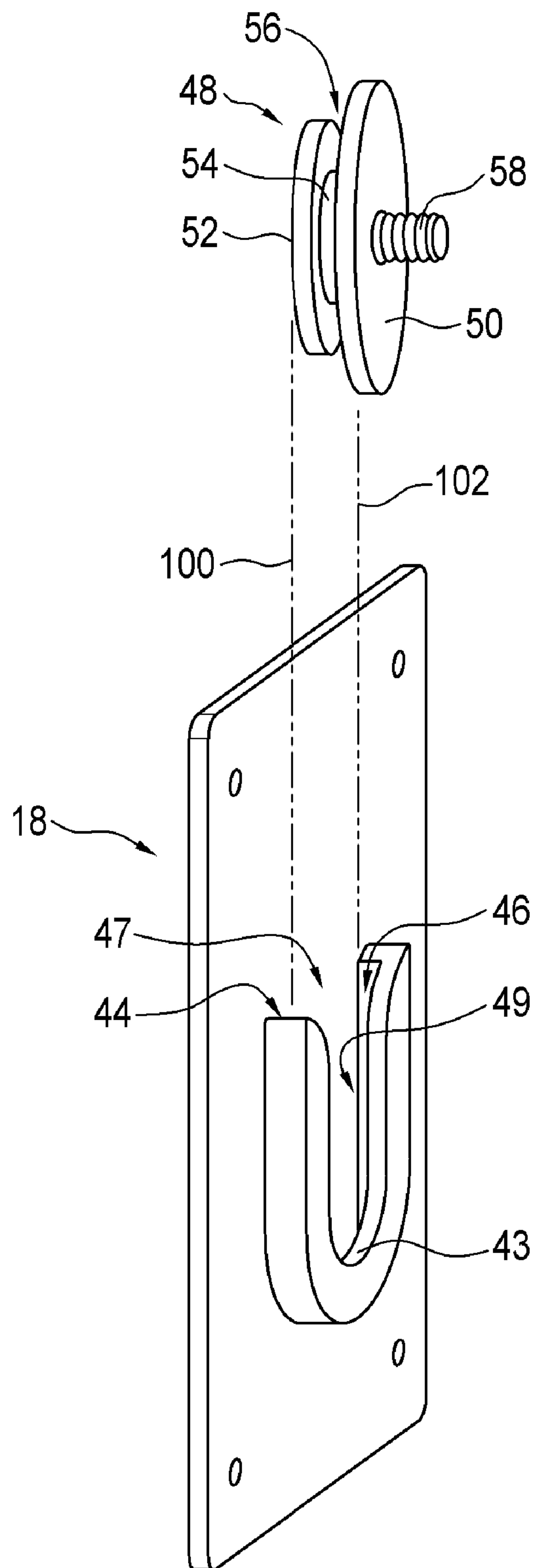
FIG. 11
