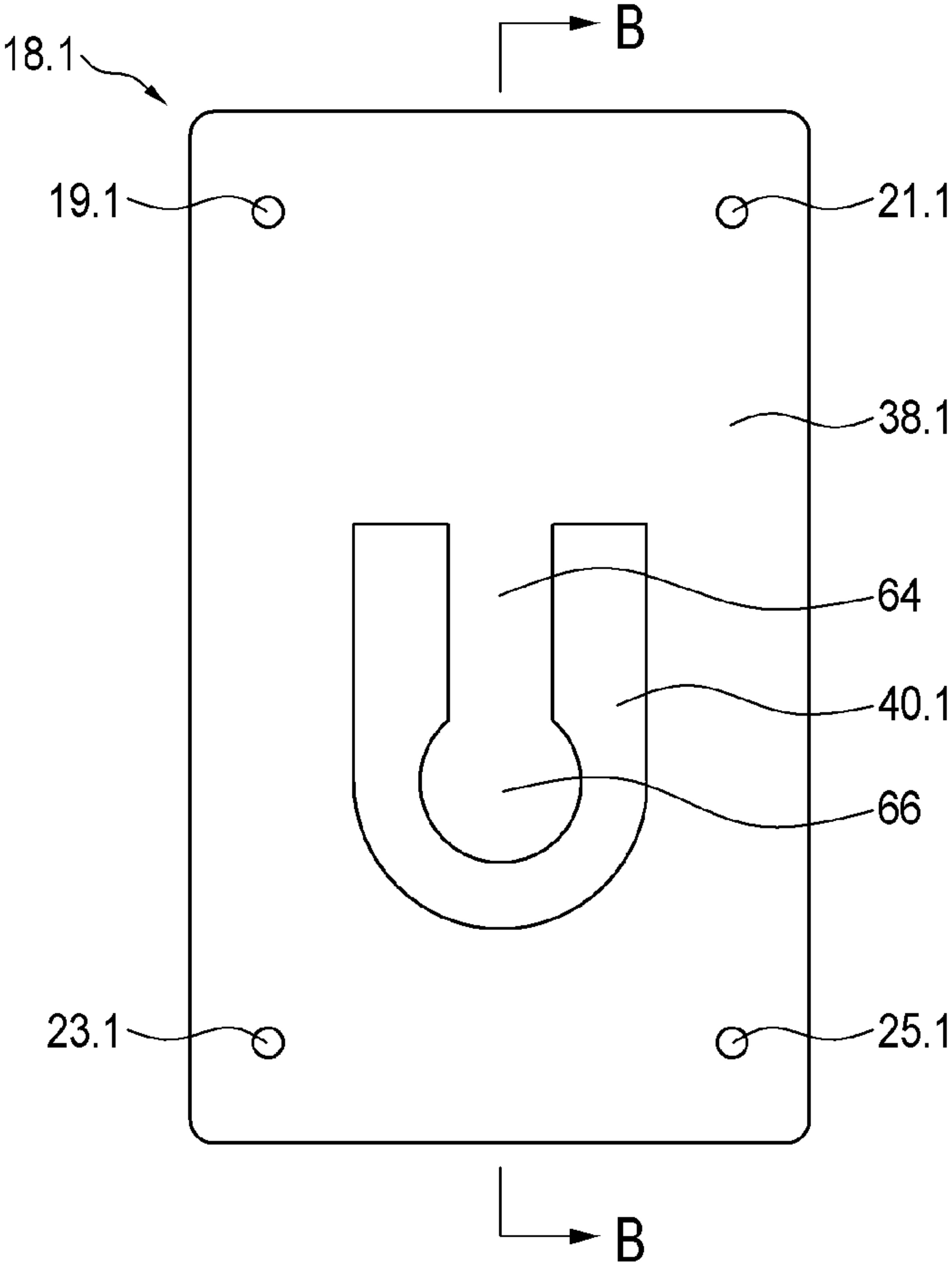
FIG. 13
