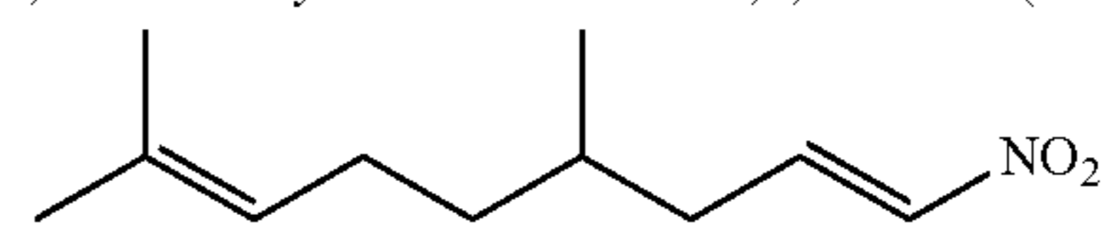
4,8-Dimethyl-1-nitronona-1,7-diene (RG-7)
