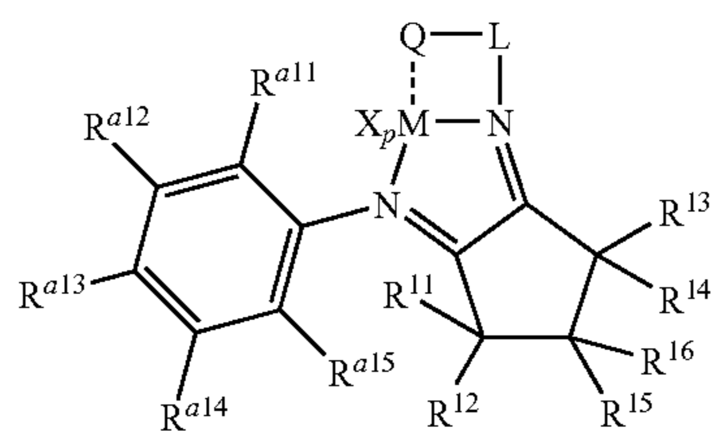
Structure 30e
