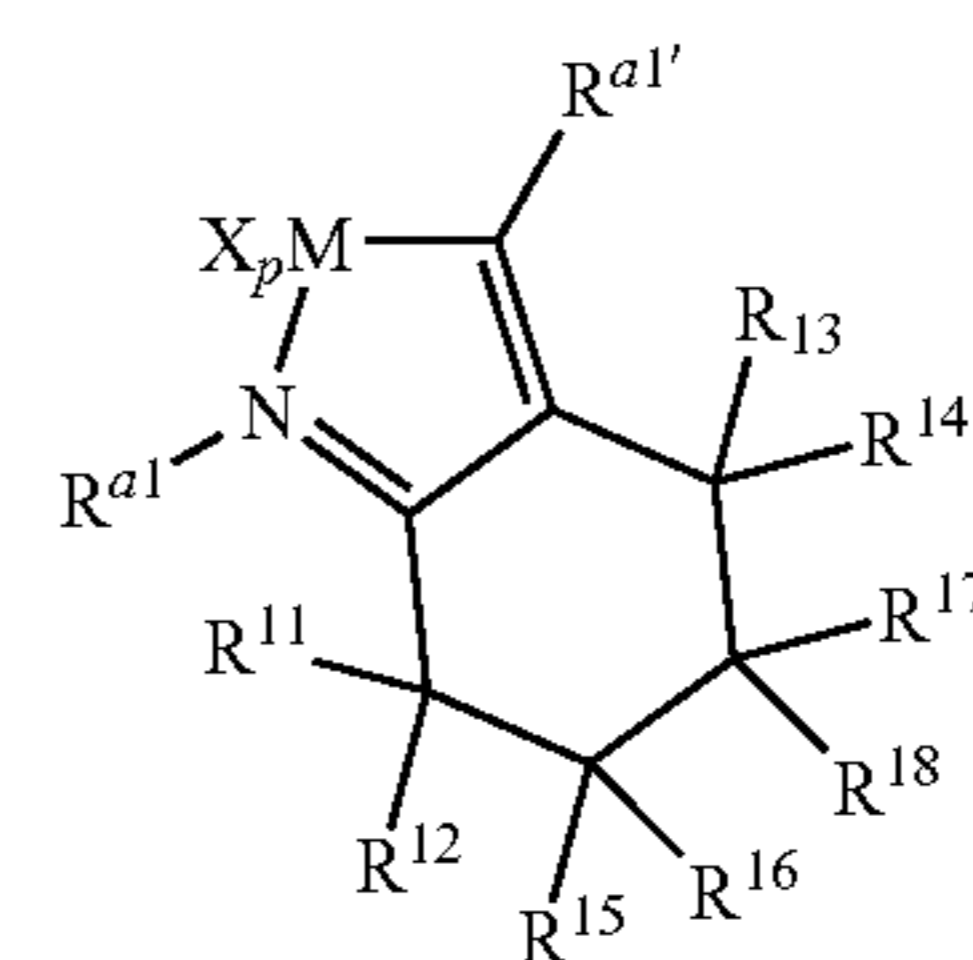
Structure 5e
