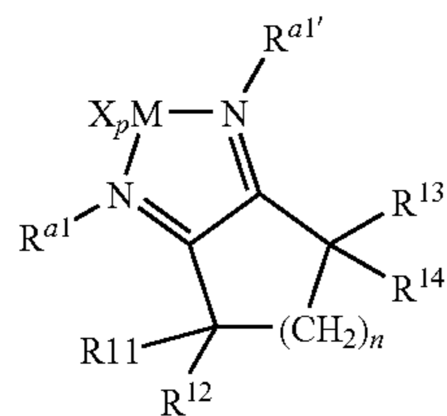
Structure 2e
