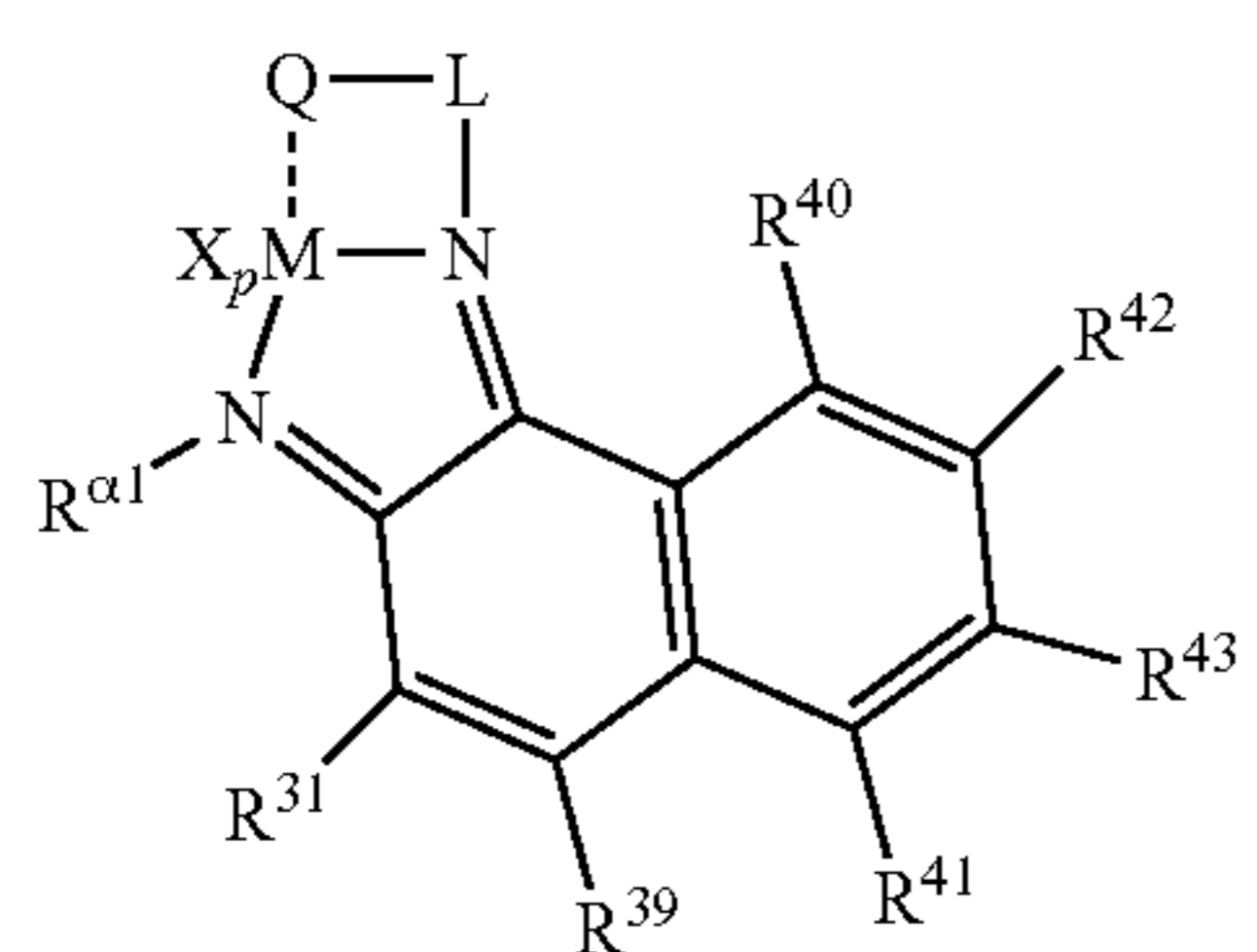
Structure 22e
