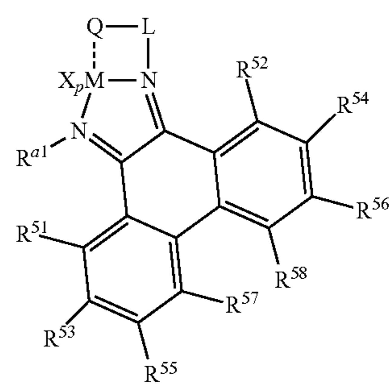
Structure 25e
