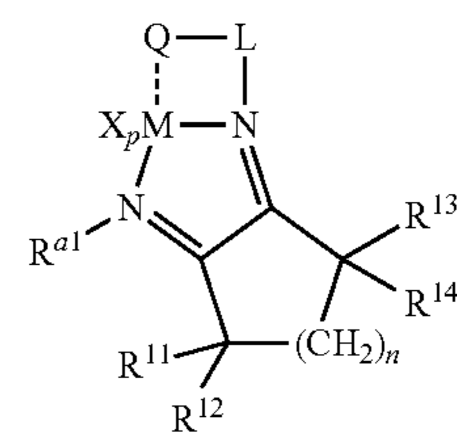
Structure 15e
