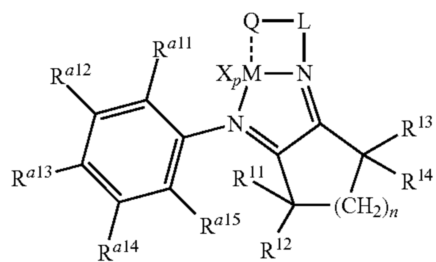
Structure 28e
