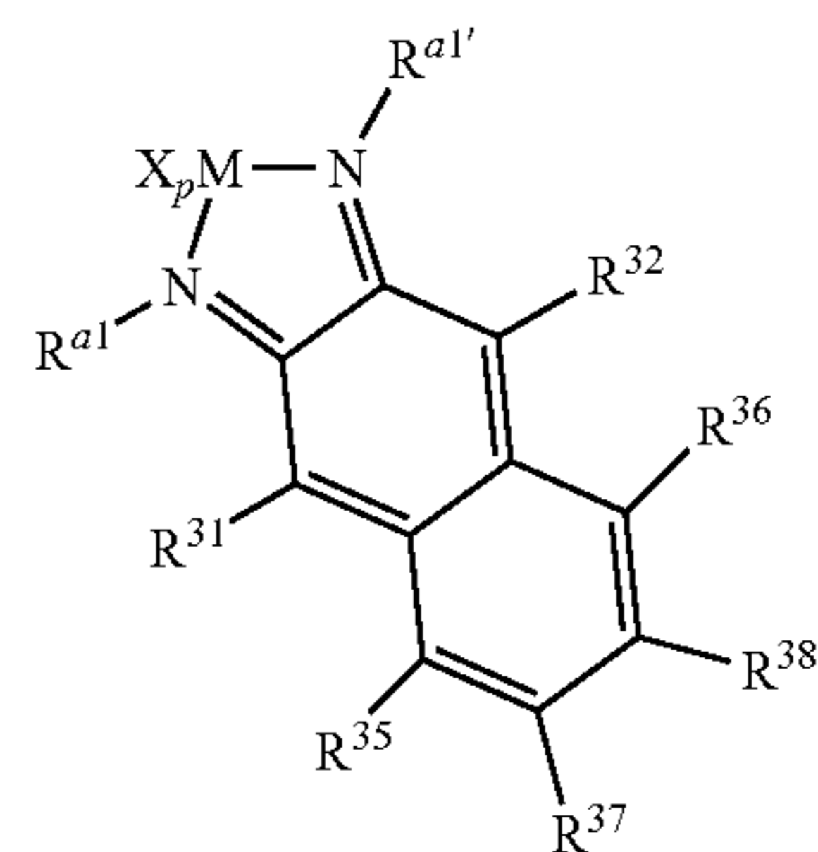
Structure 8e
