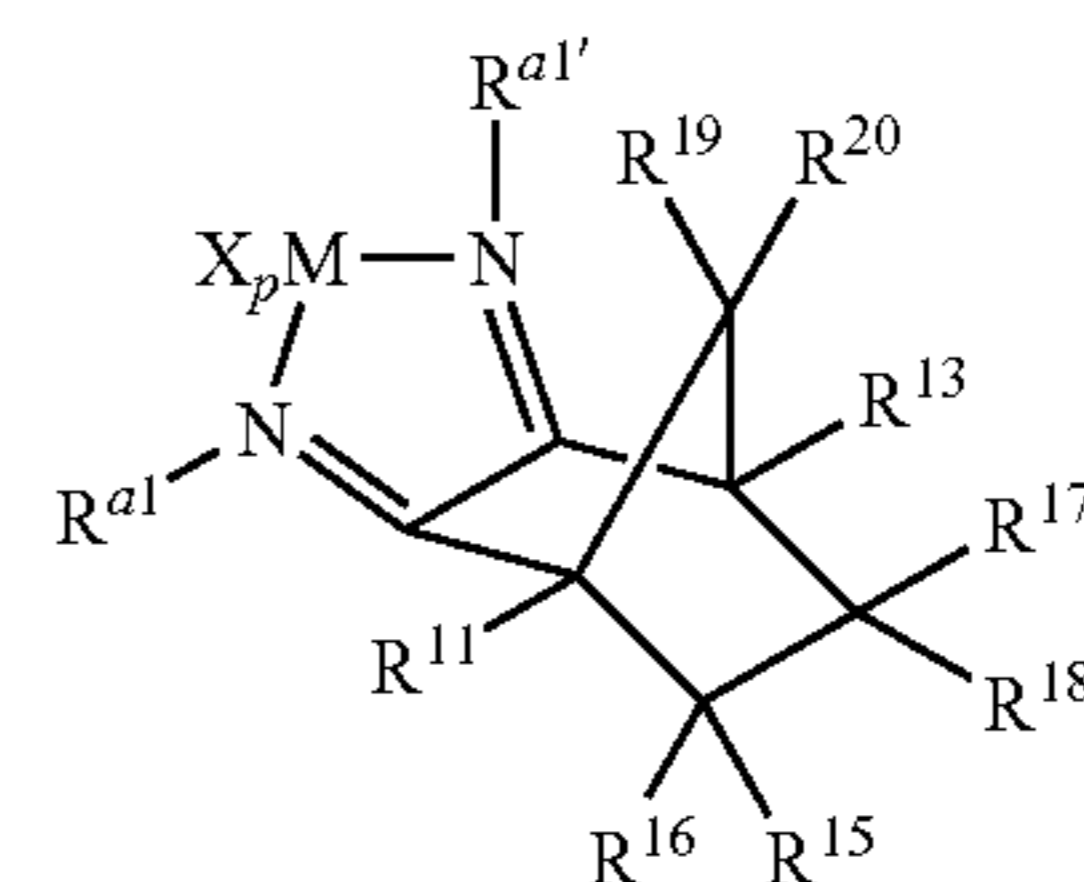
Structure 6e
