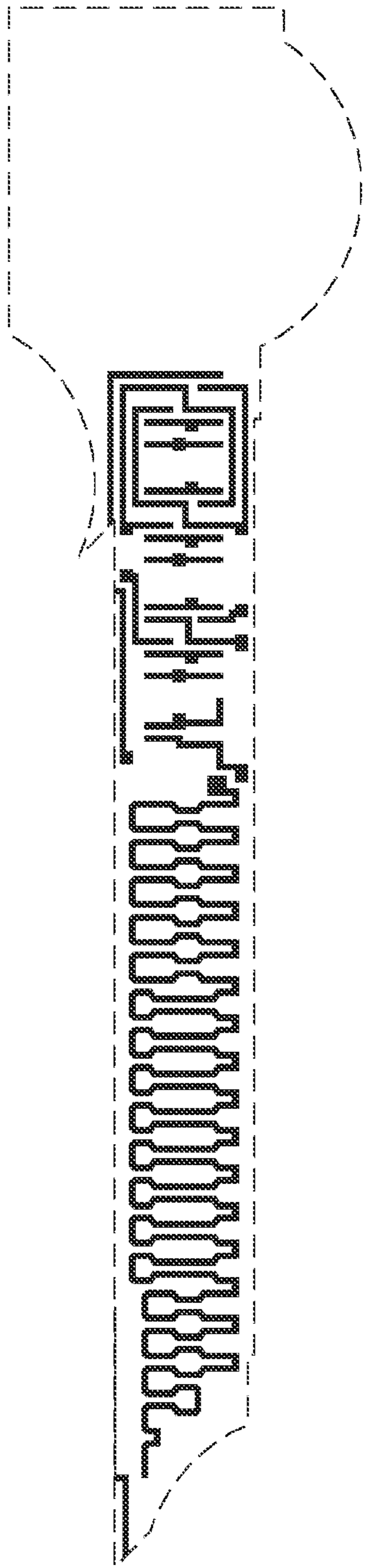
Poly mask
