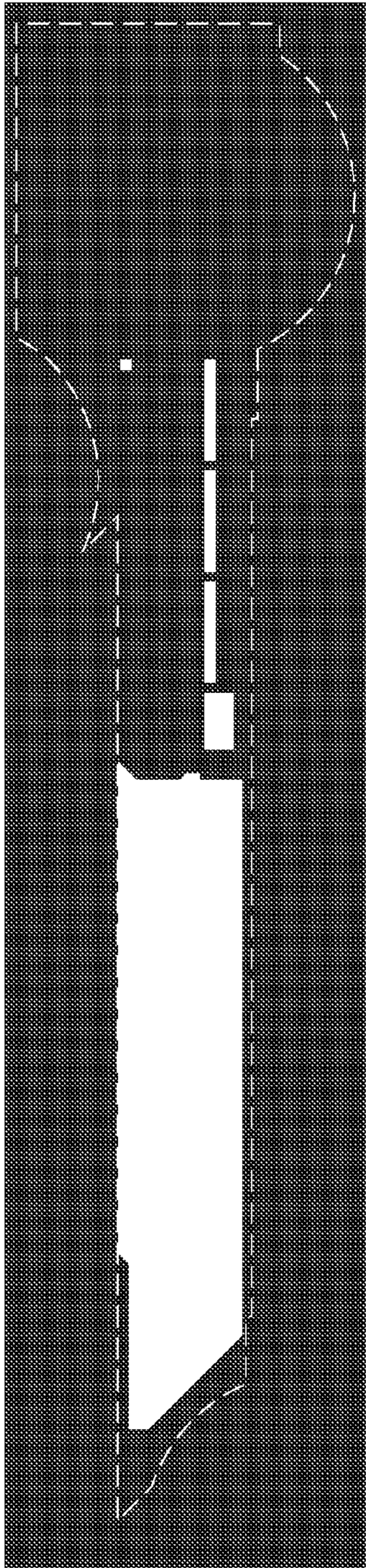
p+ mask
