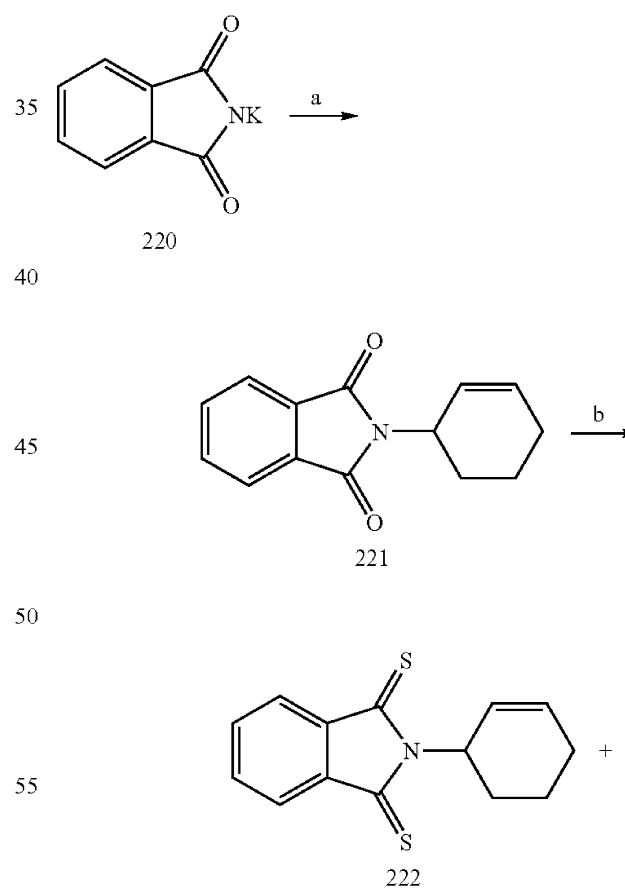
Scheme 16.
