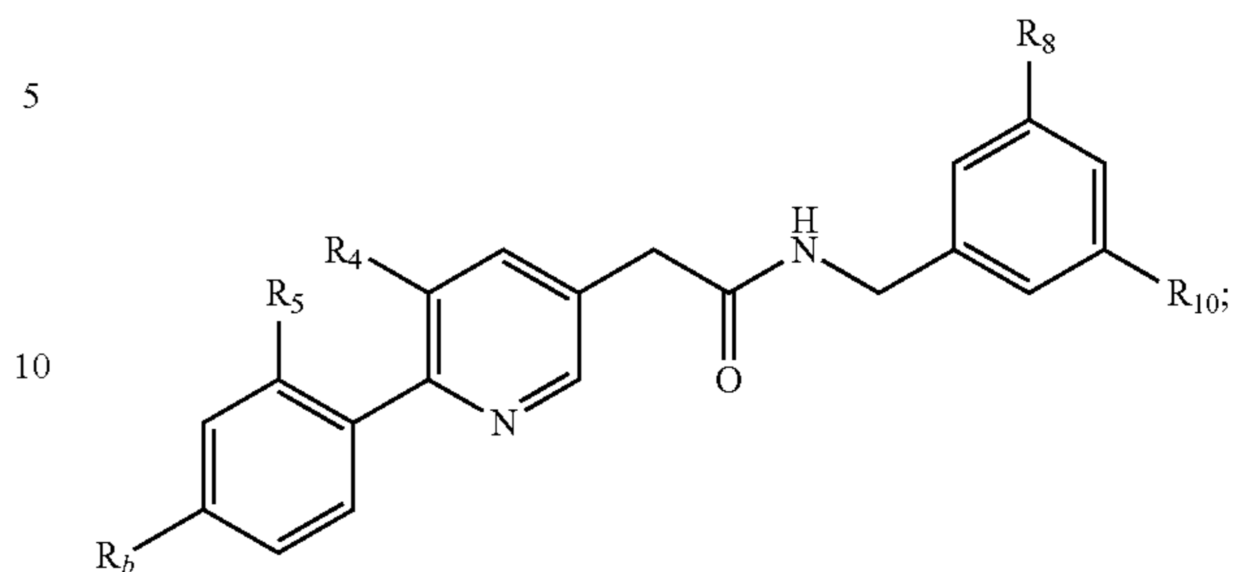
Formula VIII:
