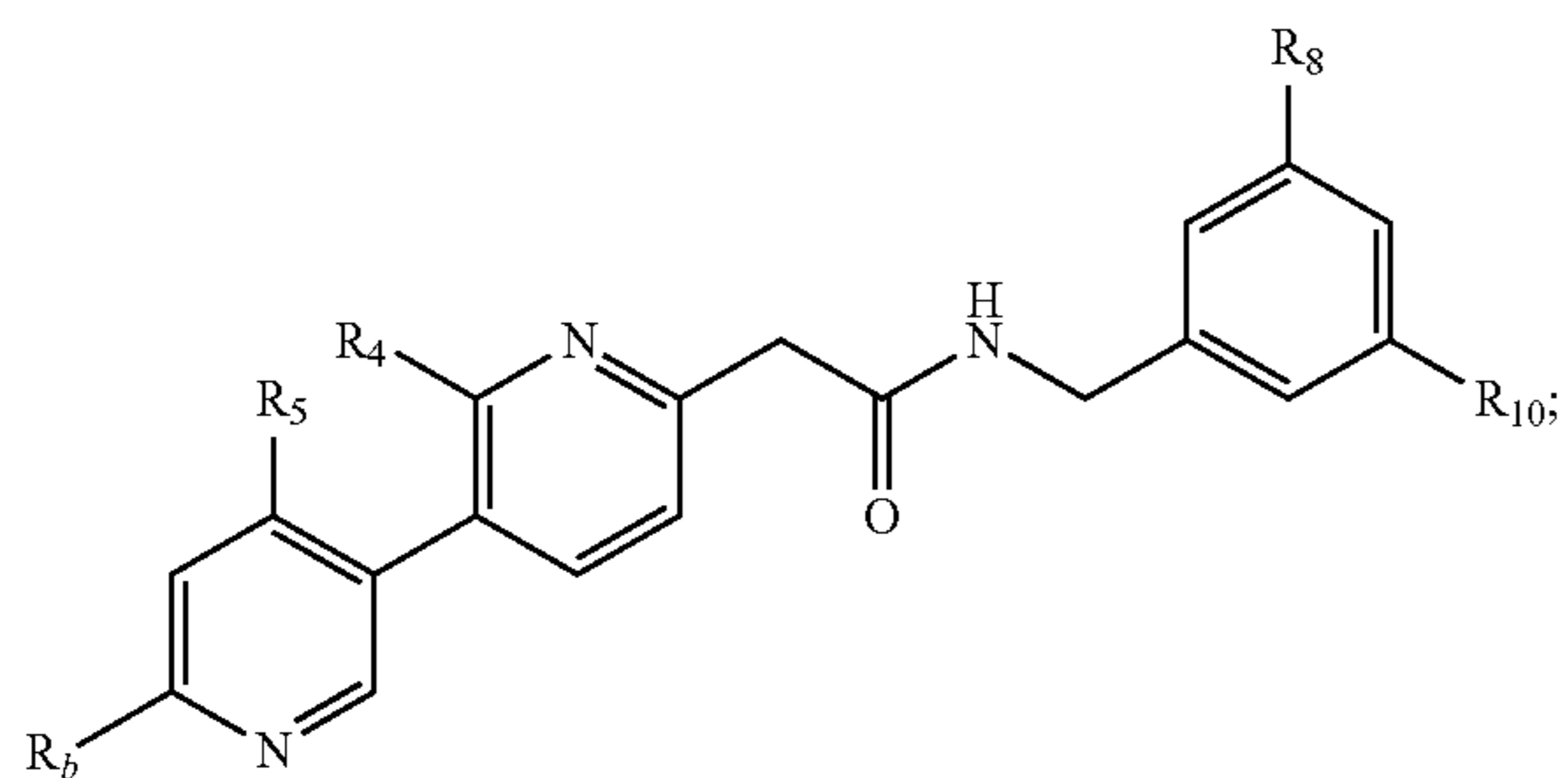
Formula VI:
