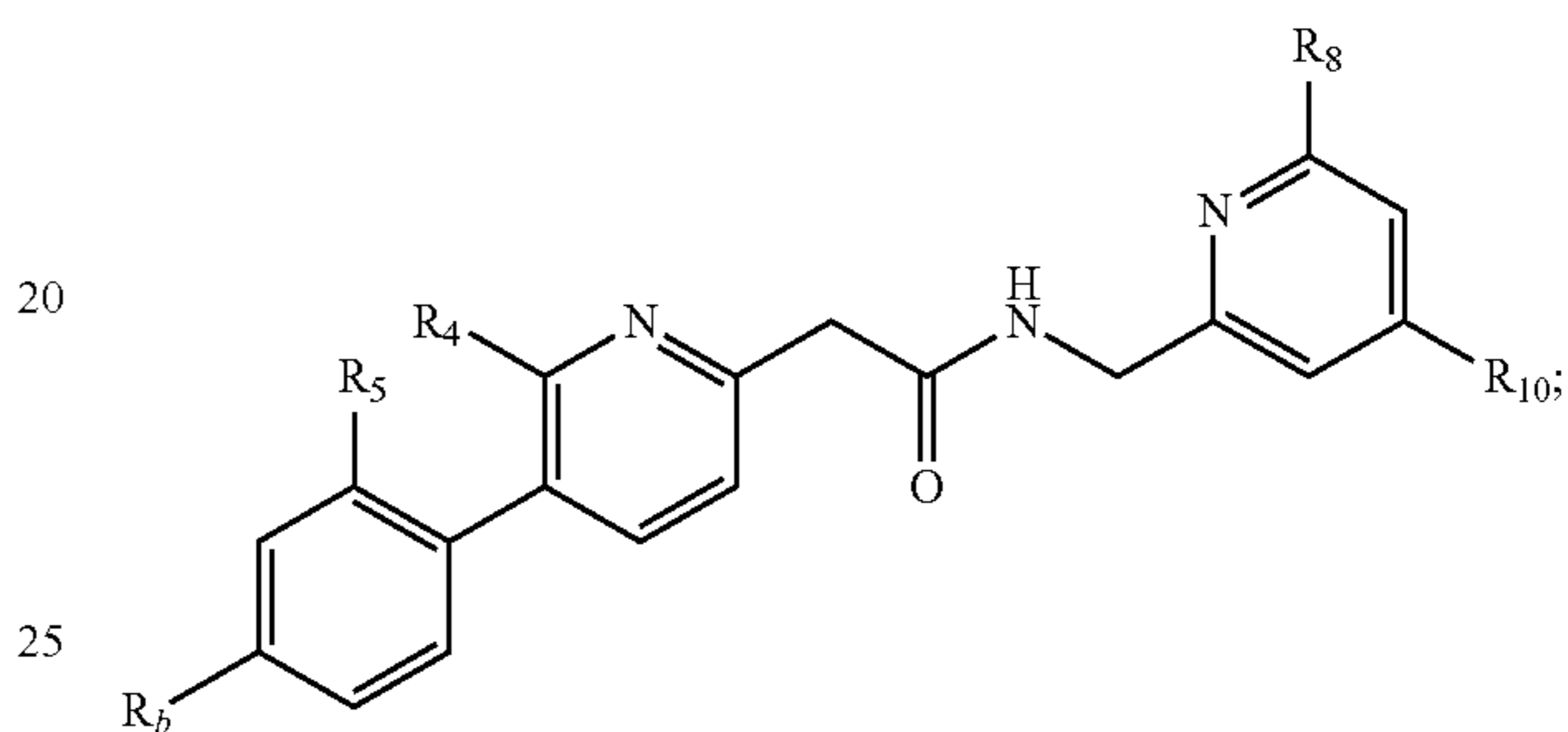
Formula VIII:
