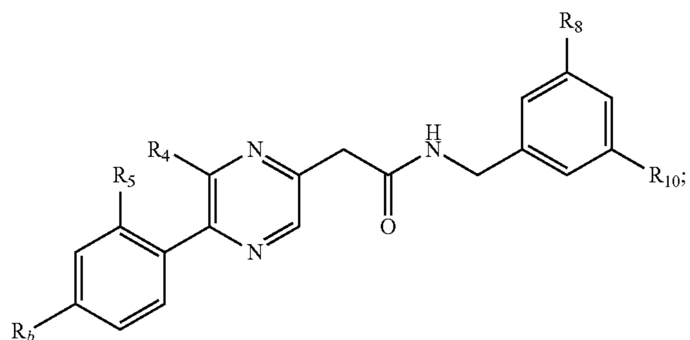
Formula VI:
