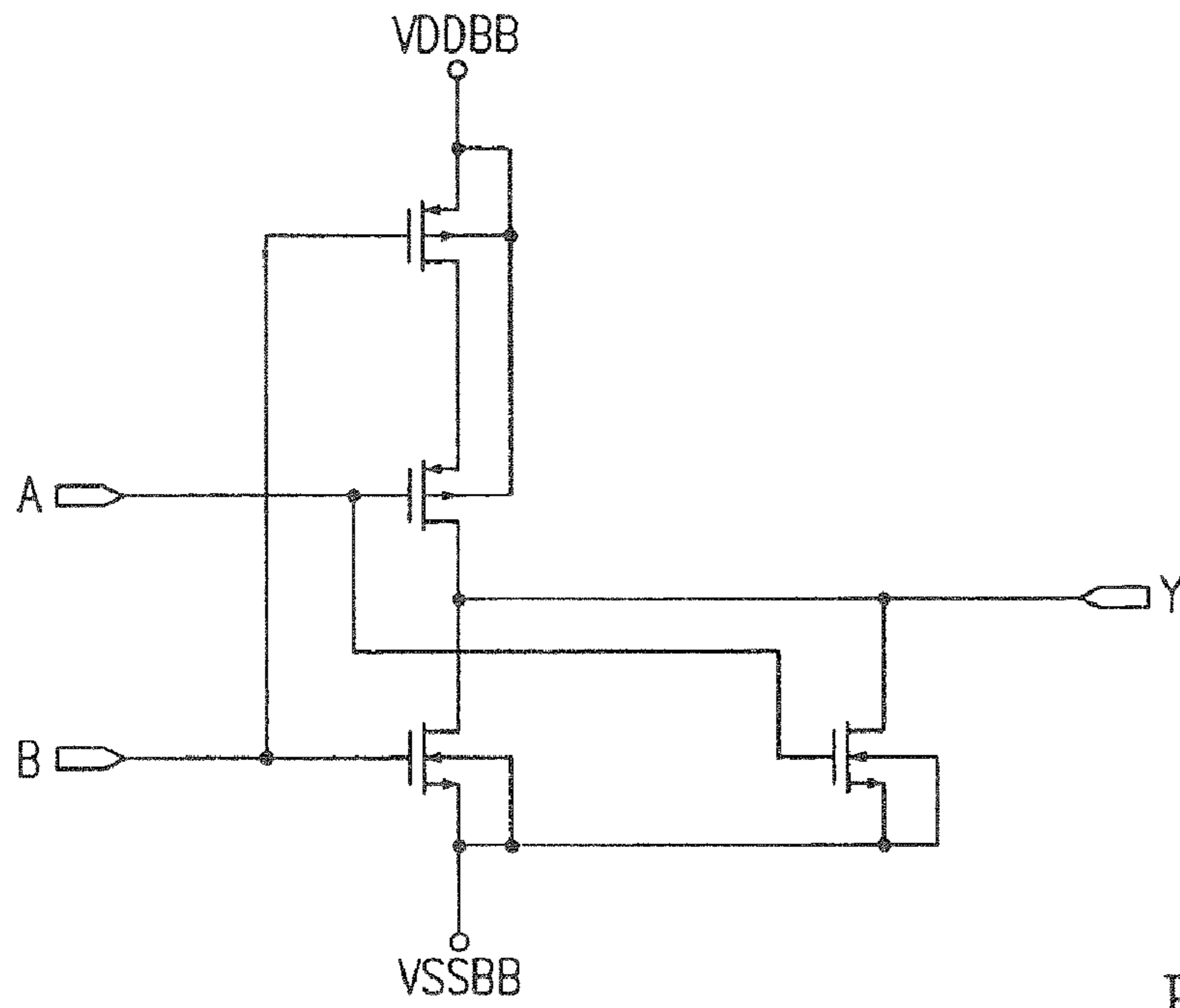
NOR2
