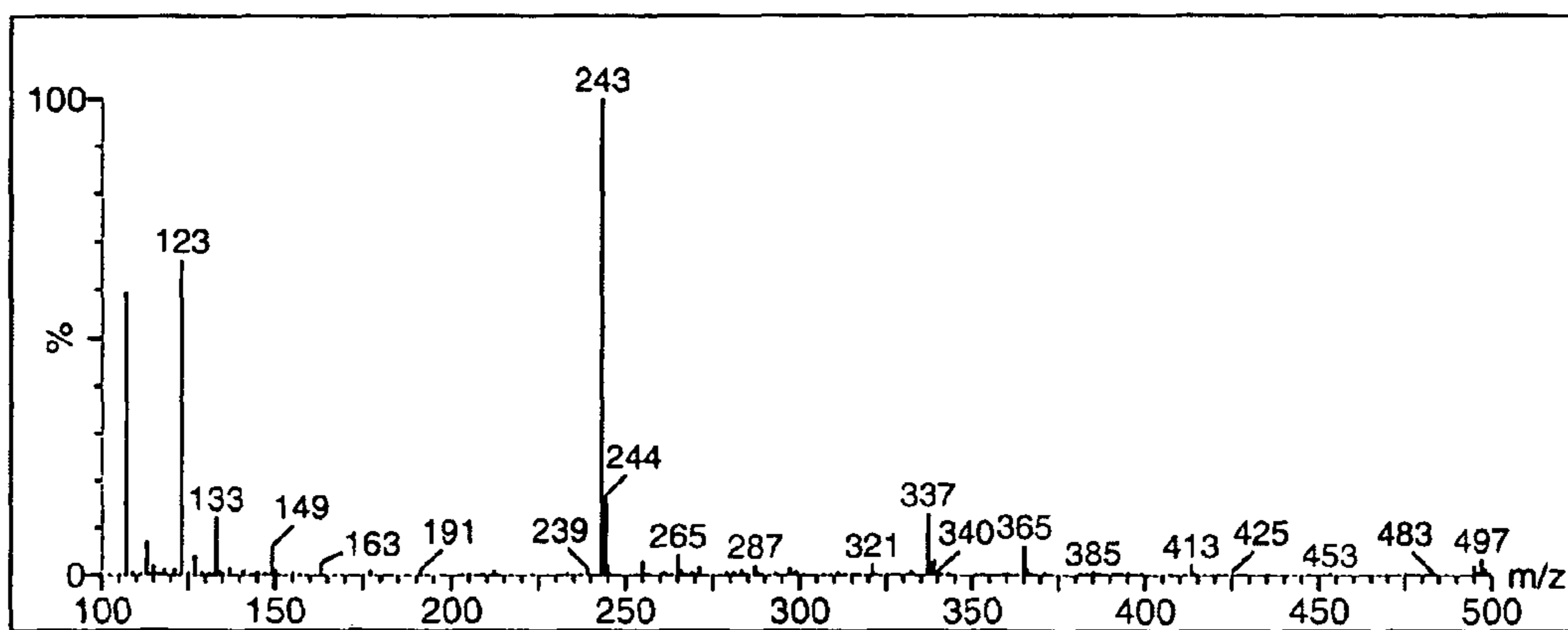
Spectrum - S-Equol
