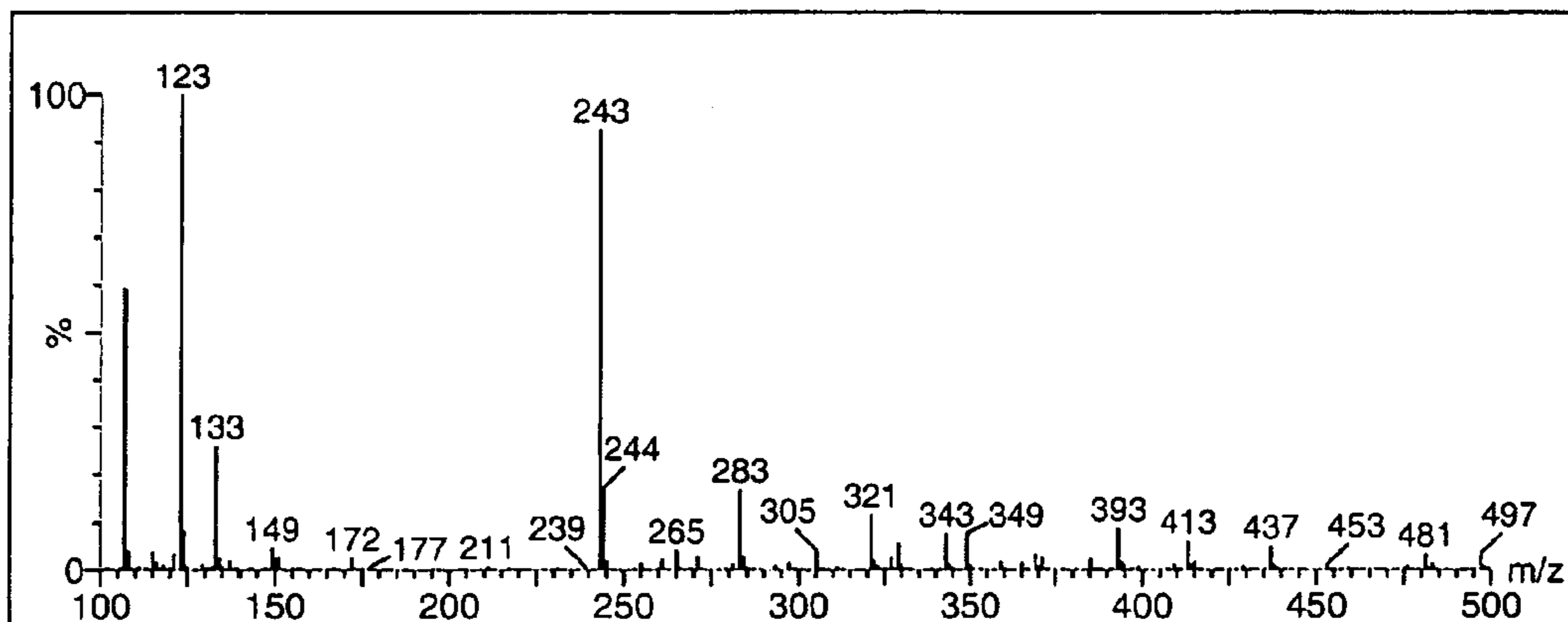
Spectrum - R-Equol
