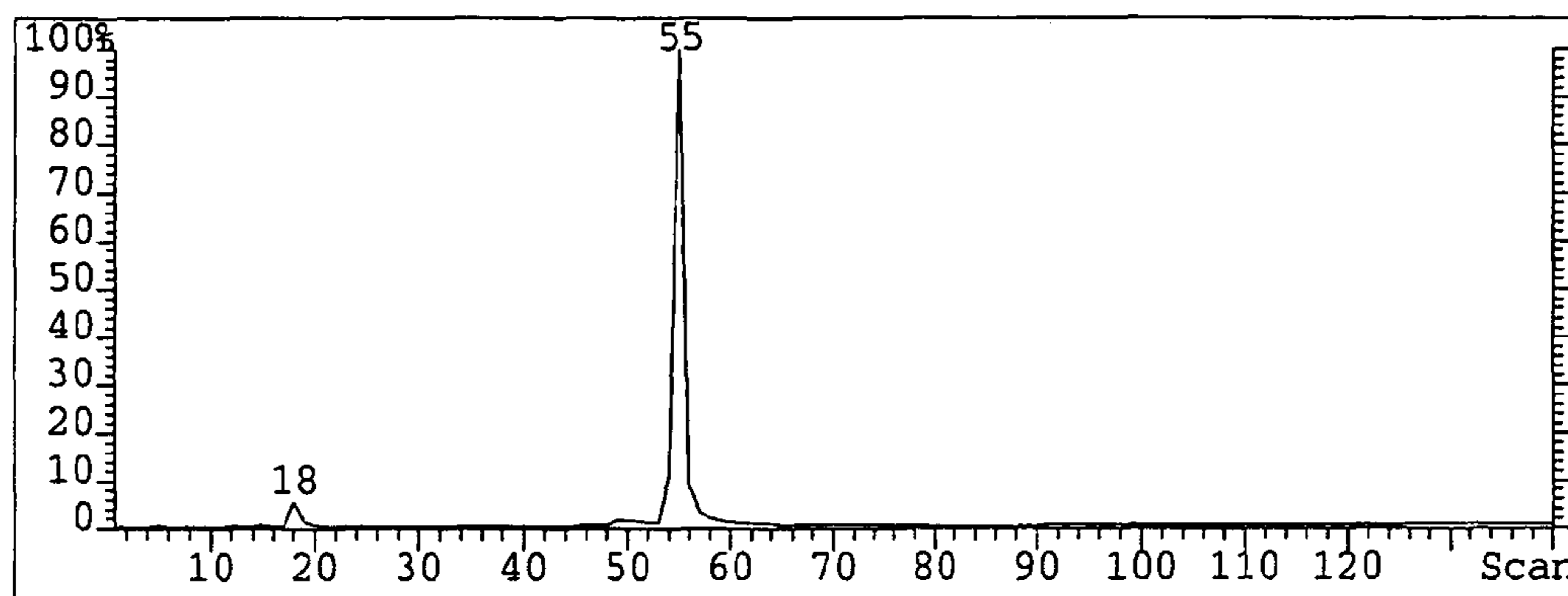
GC Trace - bis-MOM-dehydroequisol
