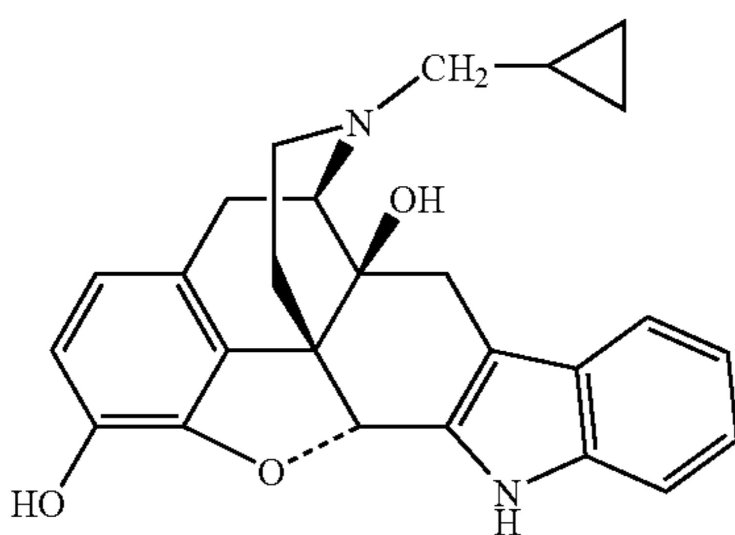
Naltrindole
