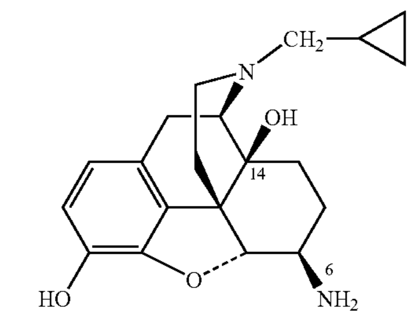
\beta -Naltrexamine
