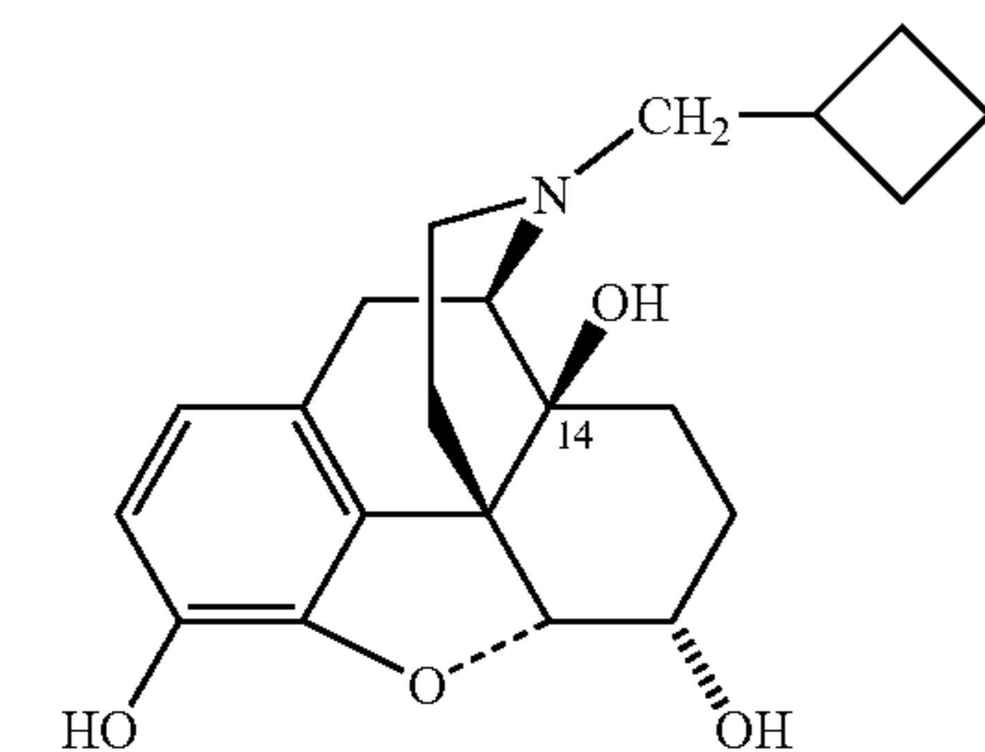
Naltrindole
