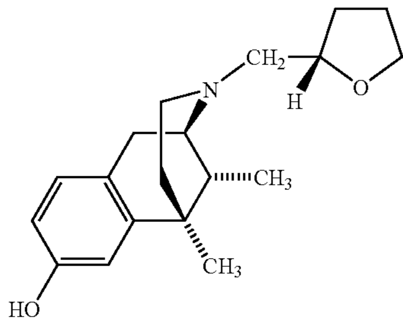
Ethylketocyclazocine (EKC)
