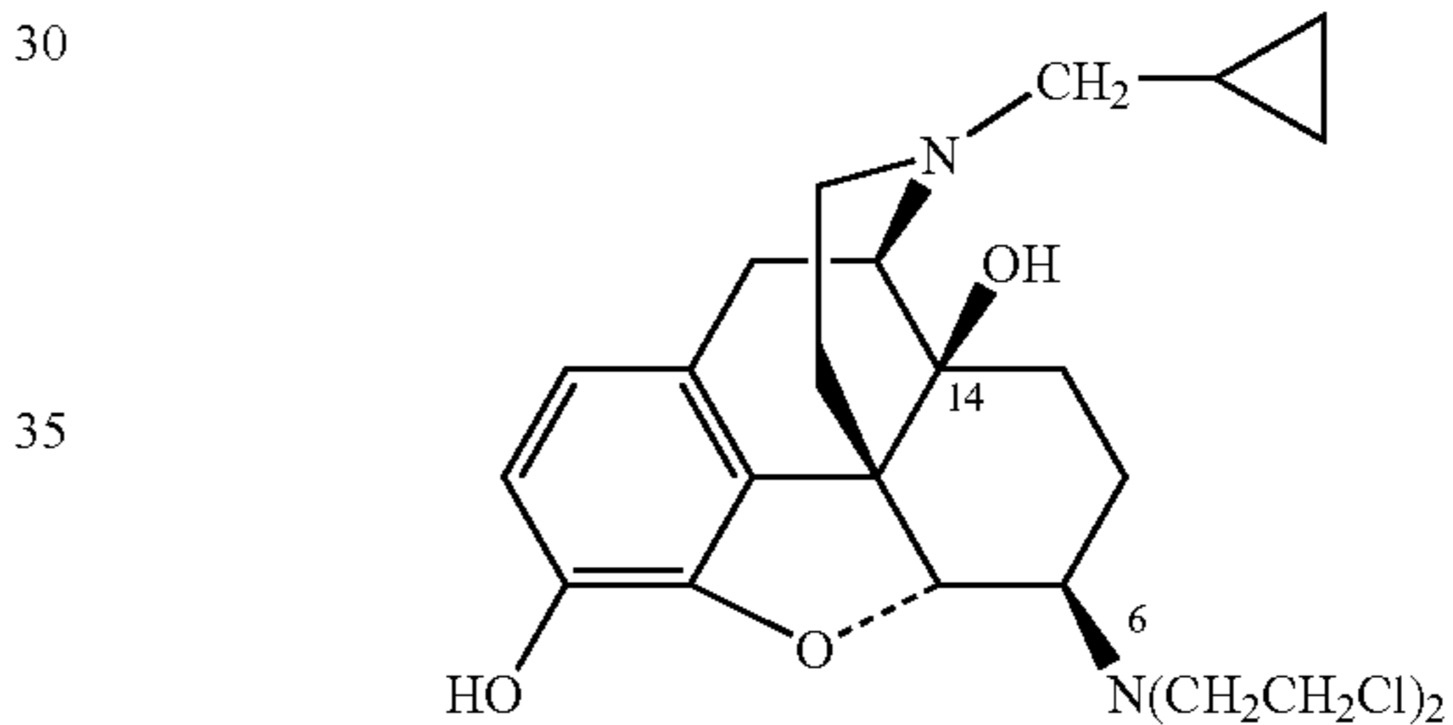
\beta -FNA
