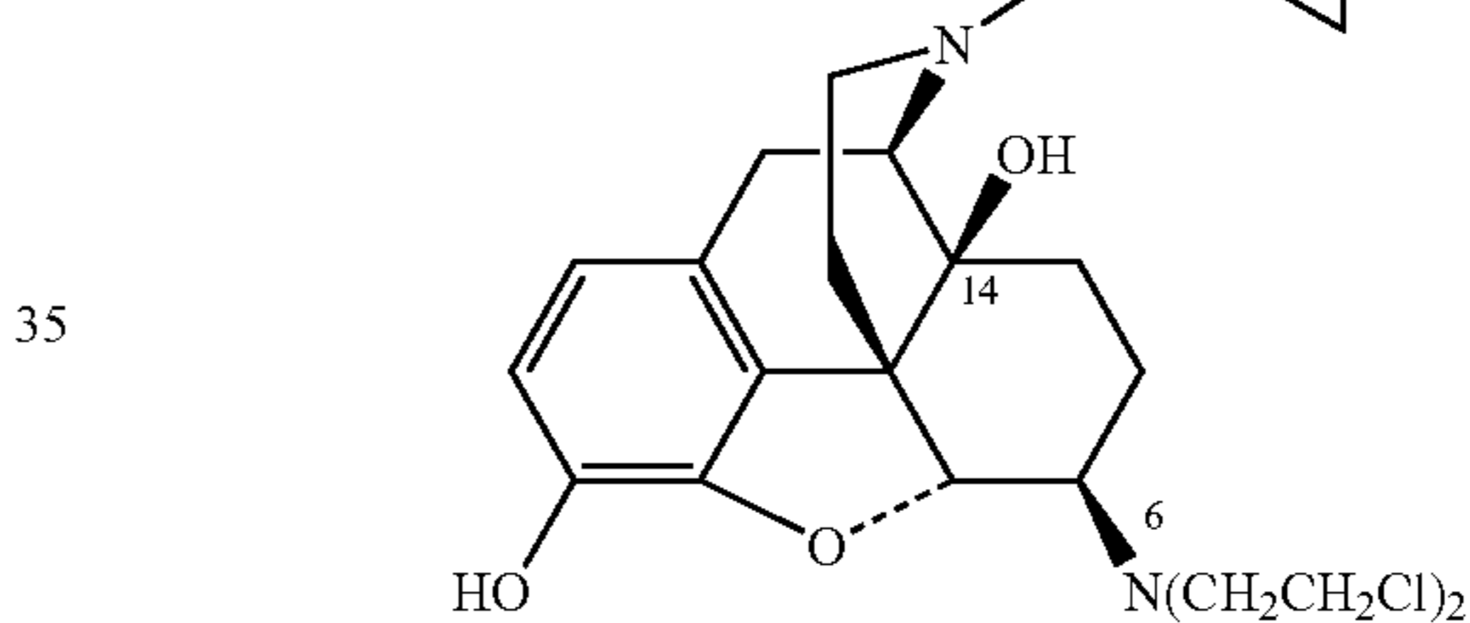
\beta -CNA
