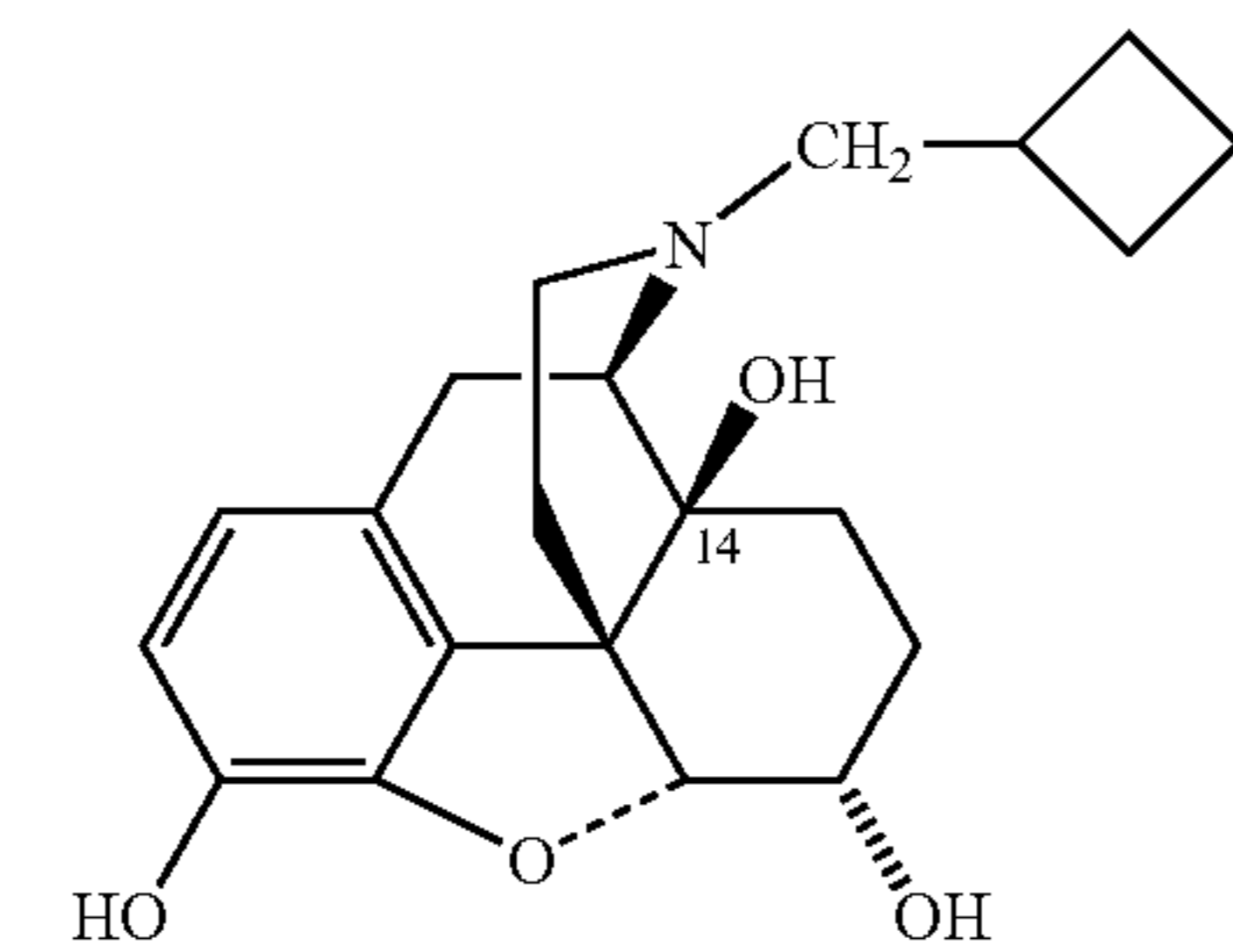
Naltrindole
