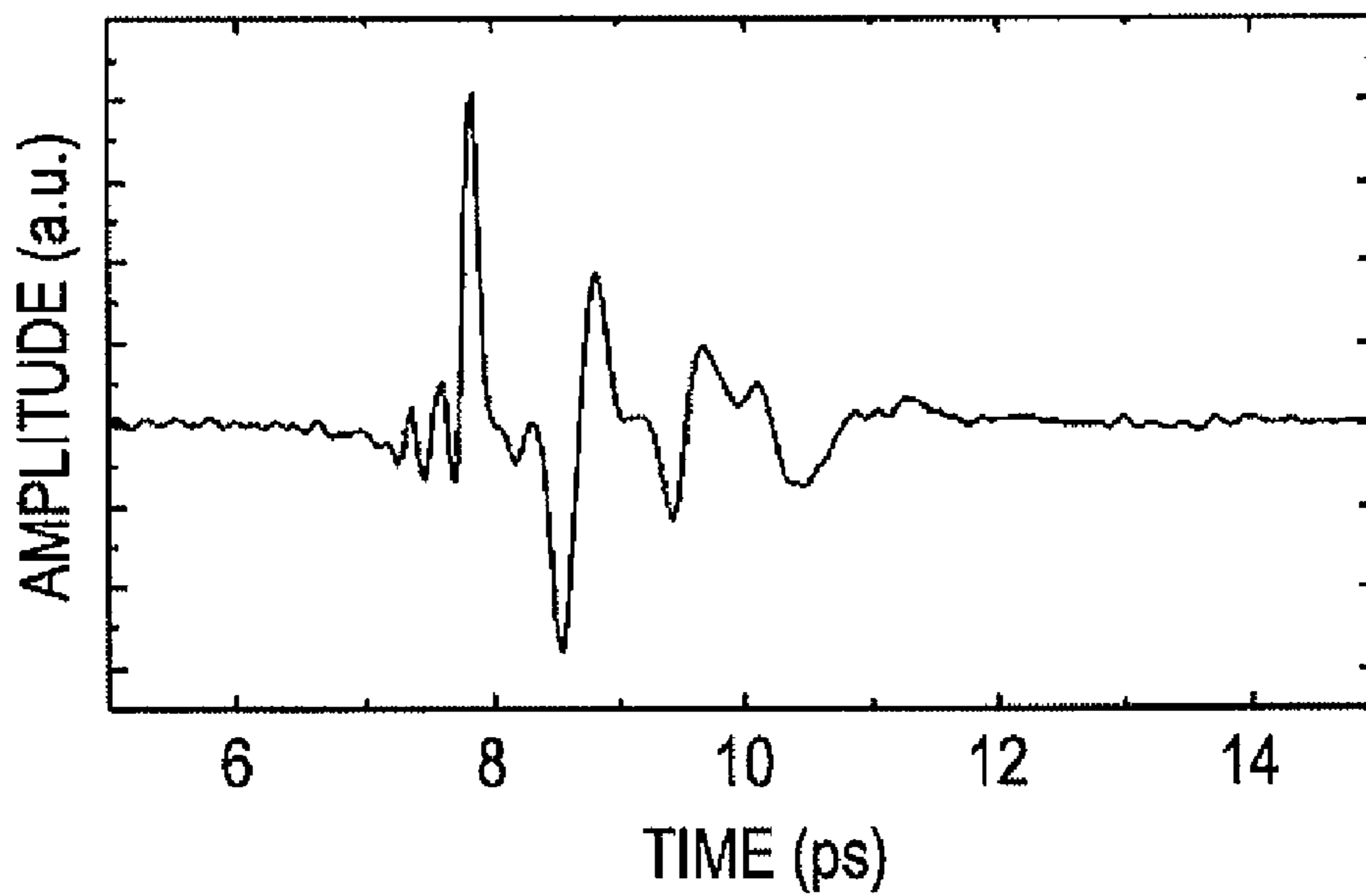
FIG. 17B
