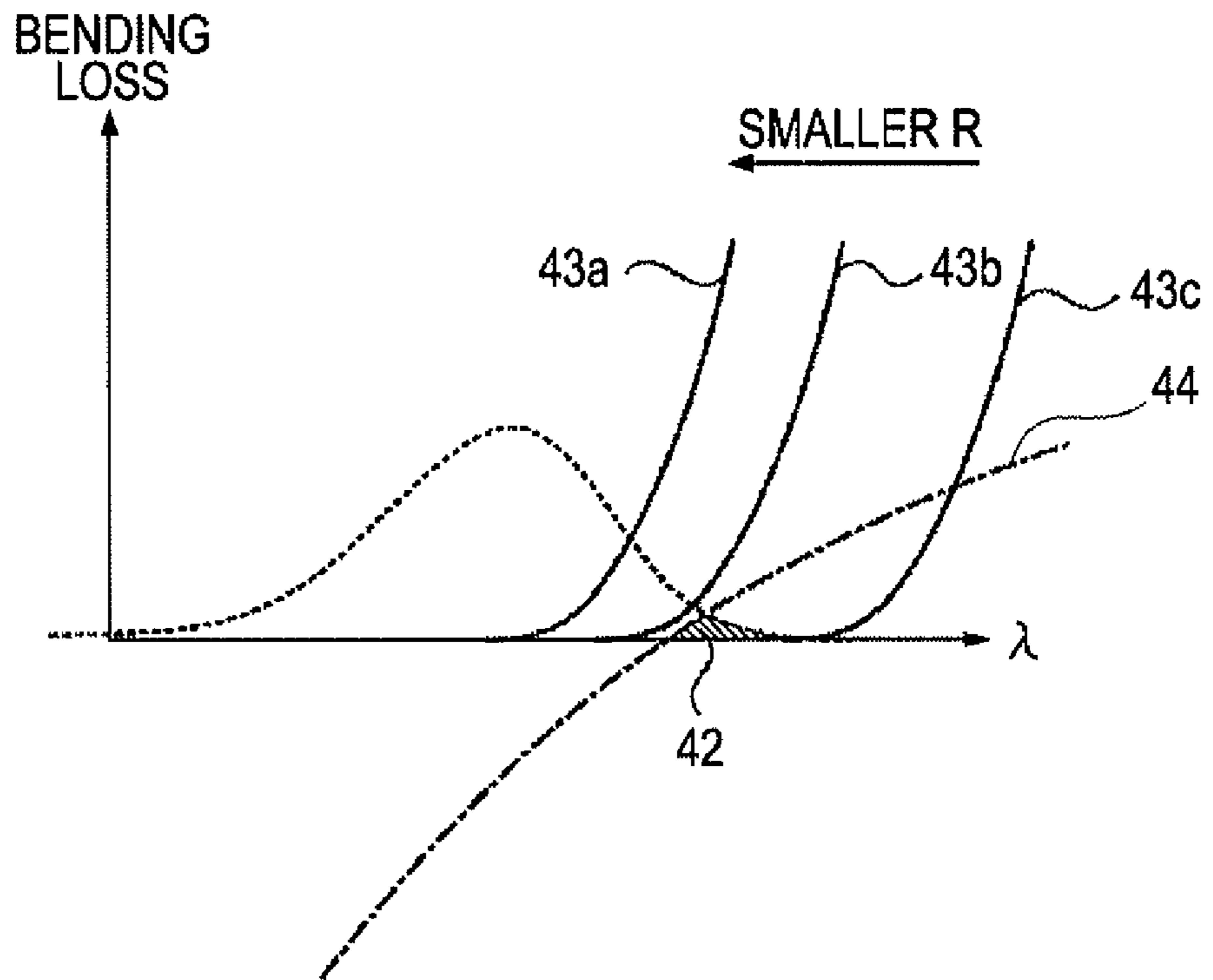
FIG. 4A
