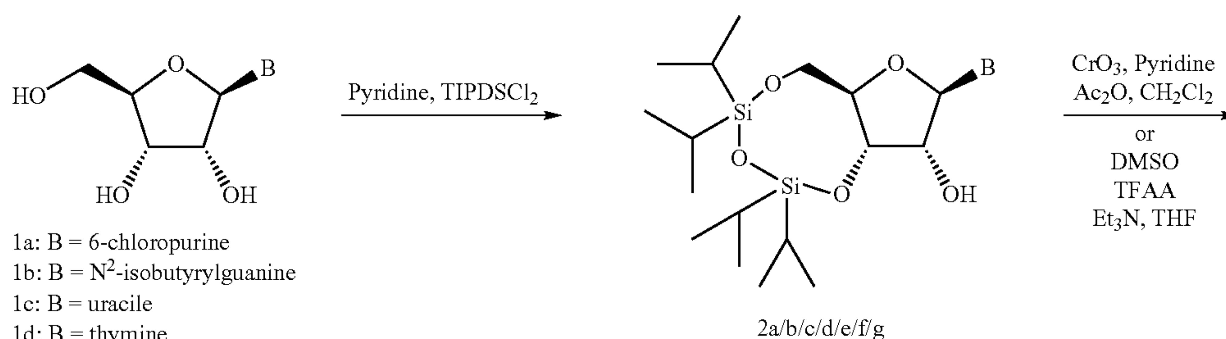
-Scheme 1-
