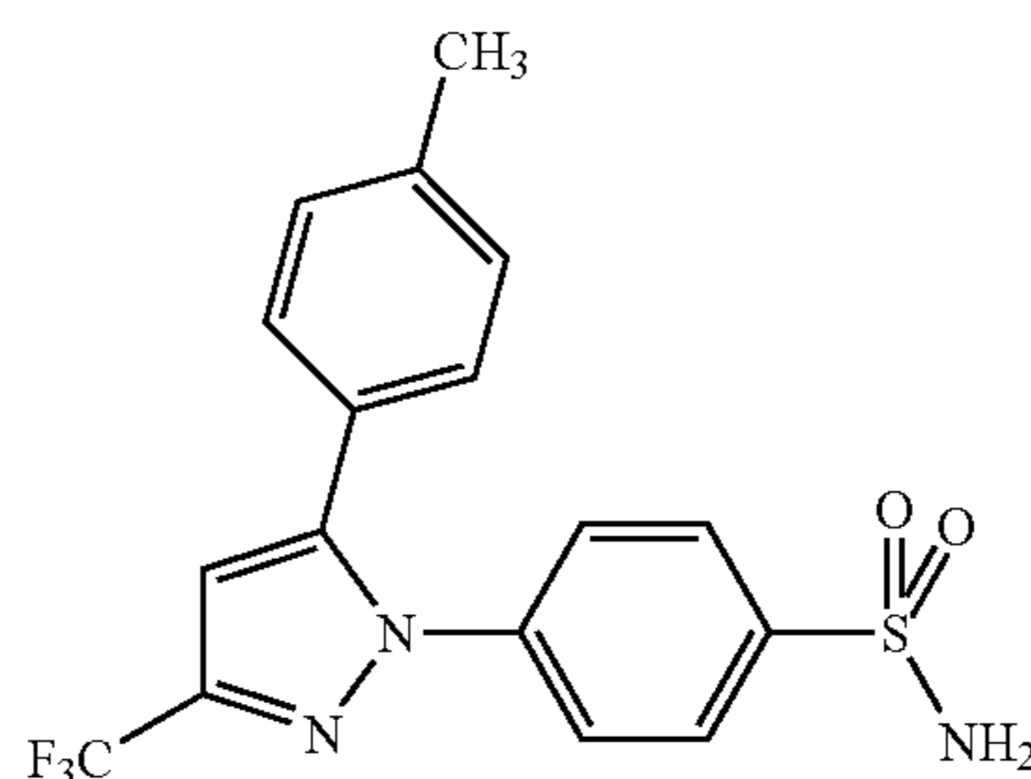
Celecoxib
