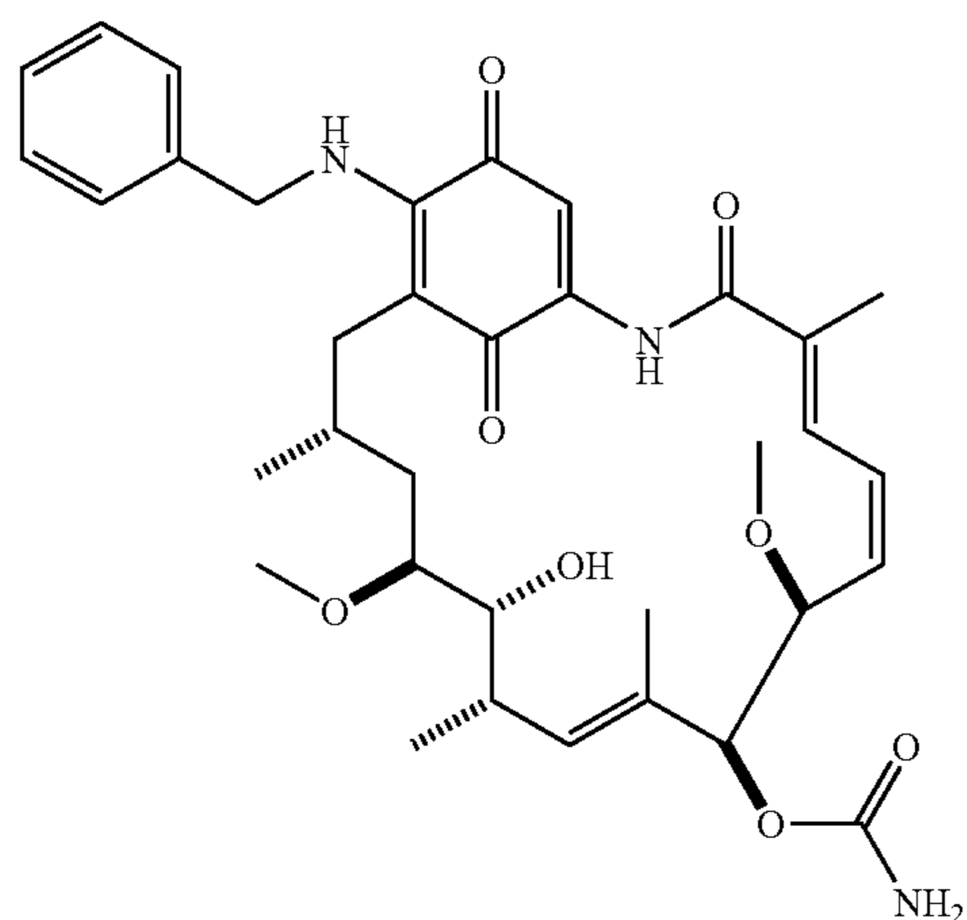
17-benzylaminogeldanamycin
