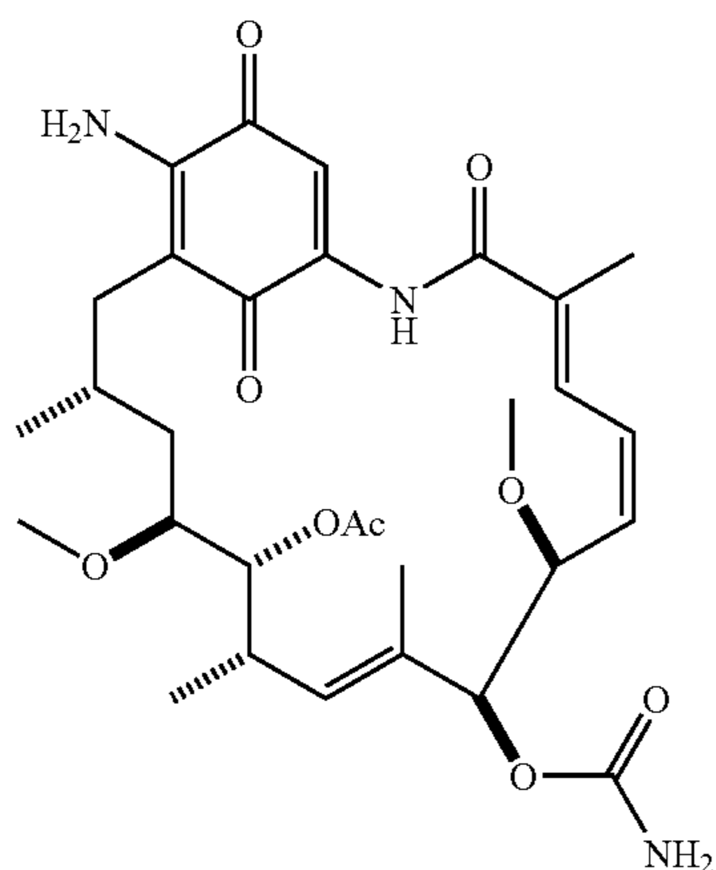
11-acetyl-17-aminogeldanamycin
