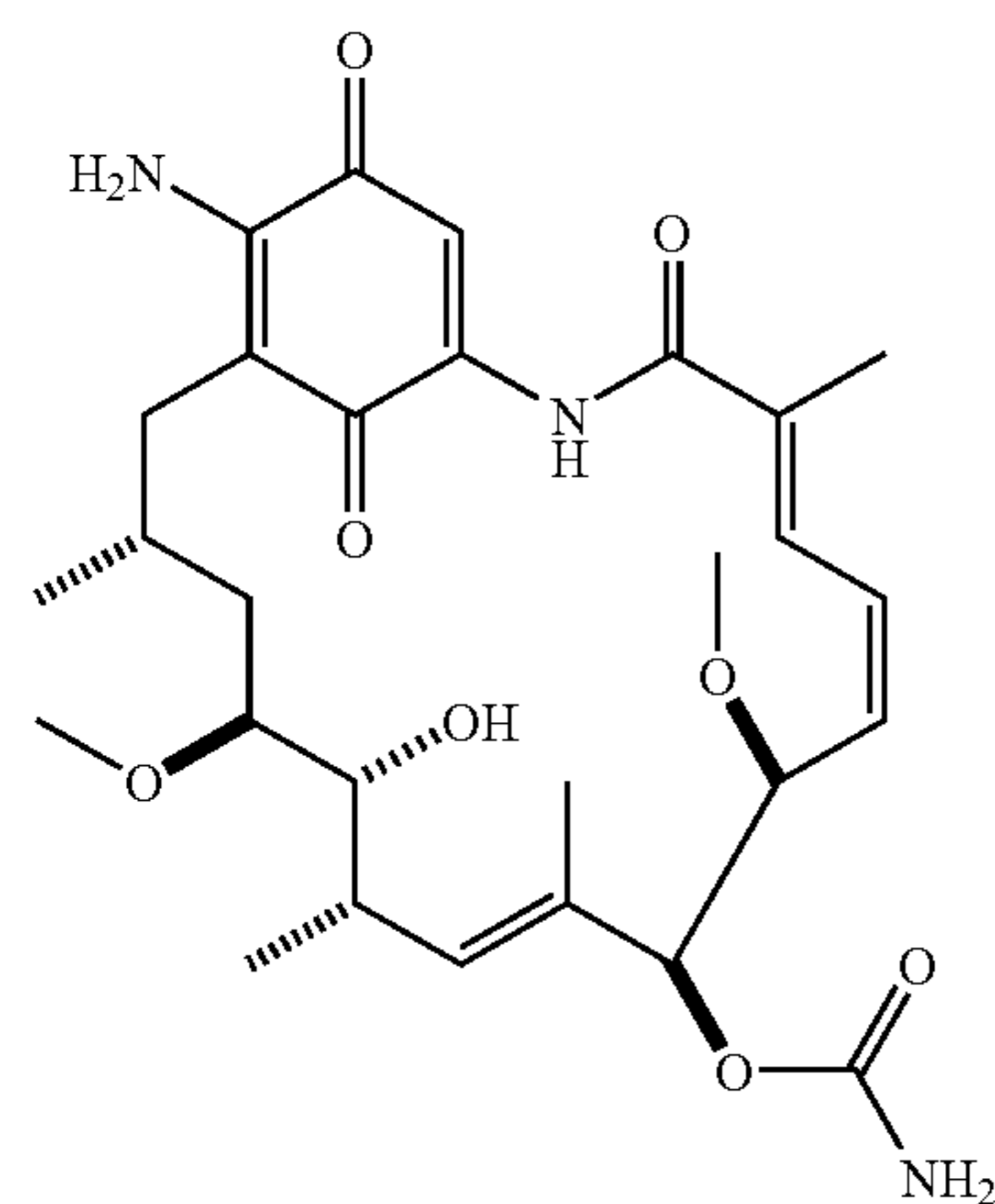
17-aminogeldanamycin
