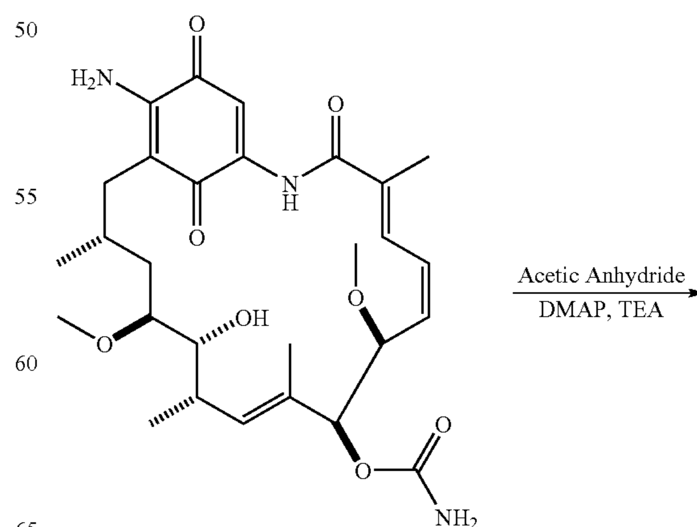
17-aminogeldanamycin
