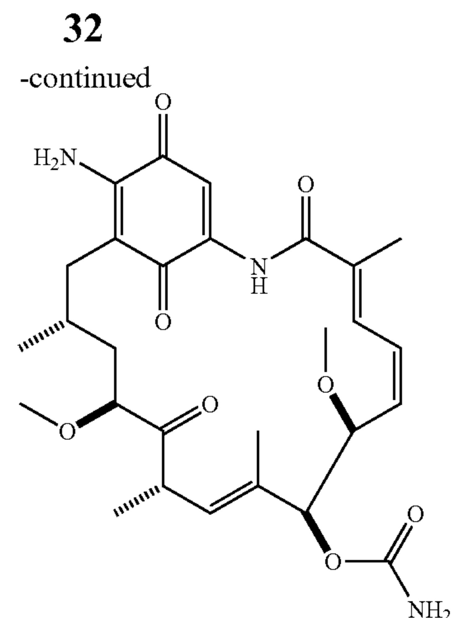
11-oxo-17-aminogeldanamycin
