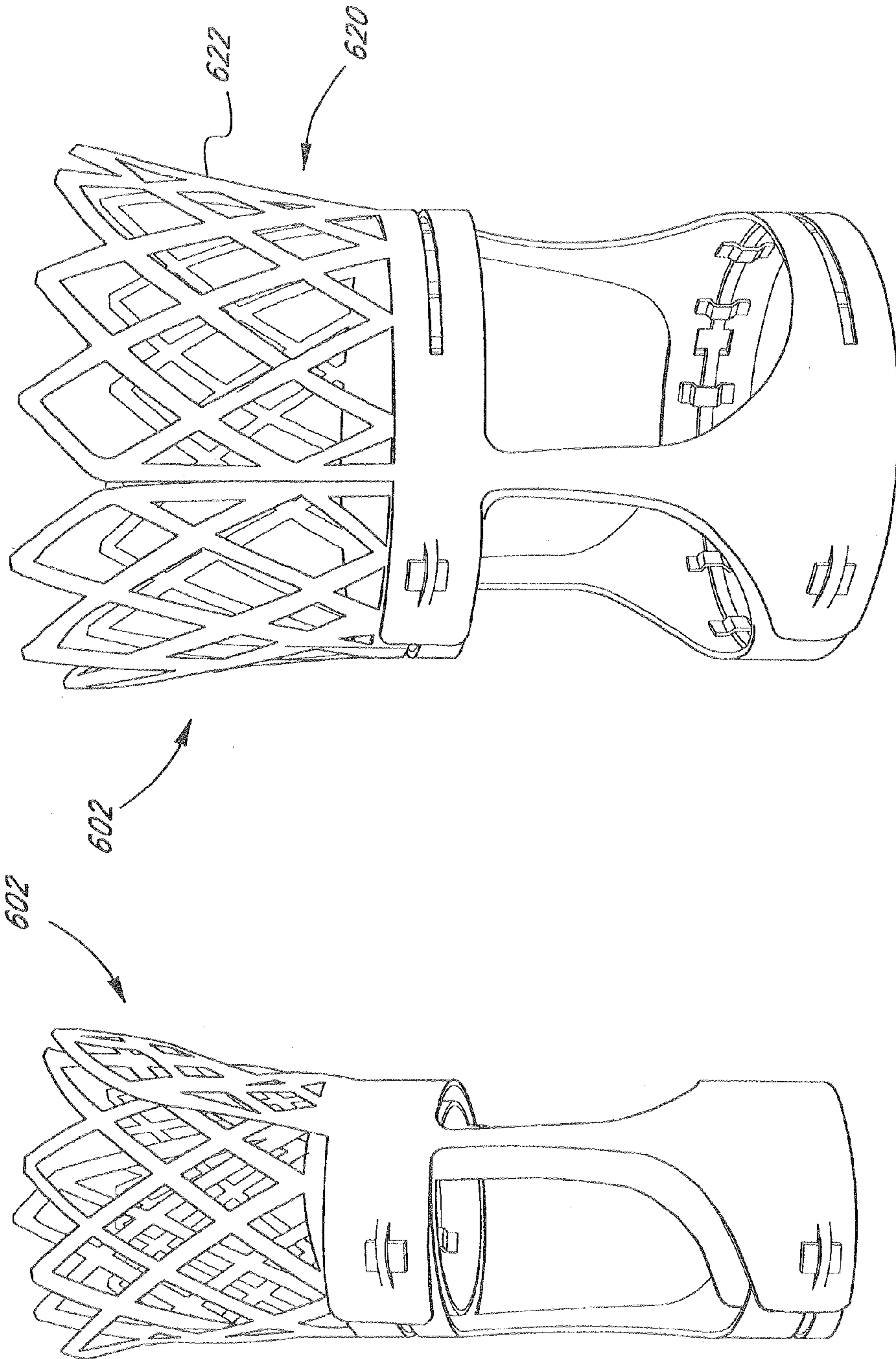
FIG. 21B
