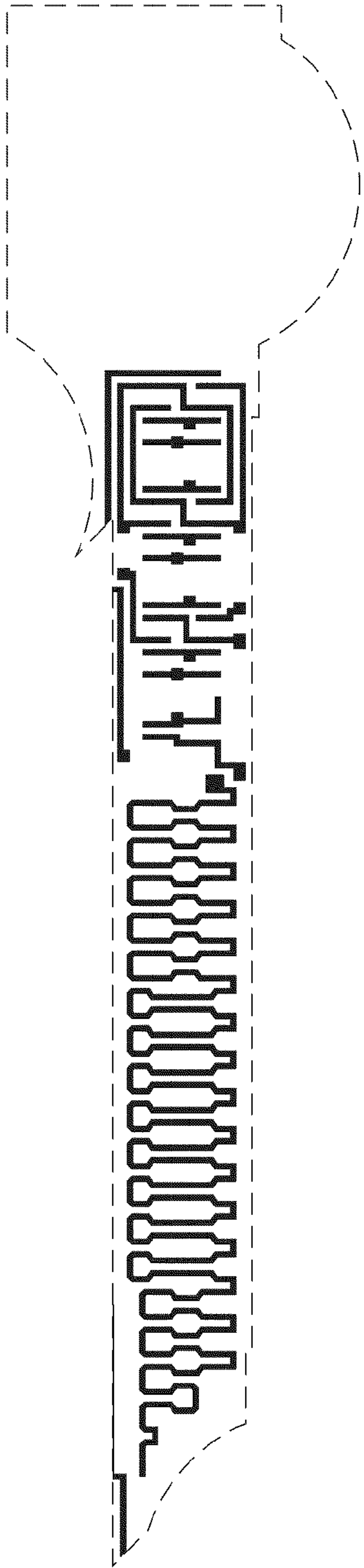
Poly mask
