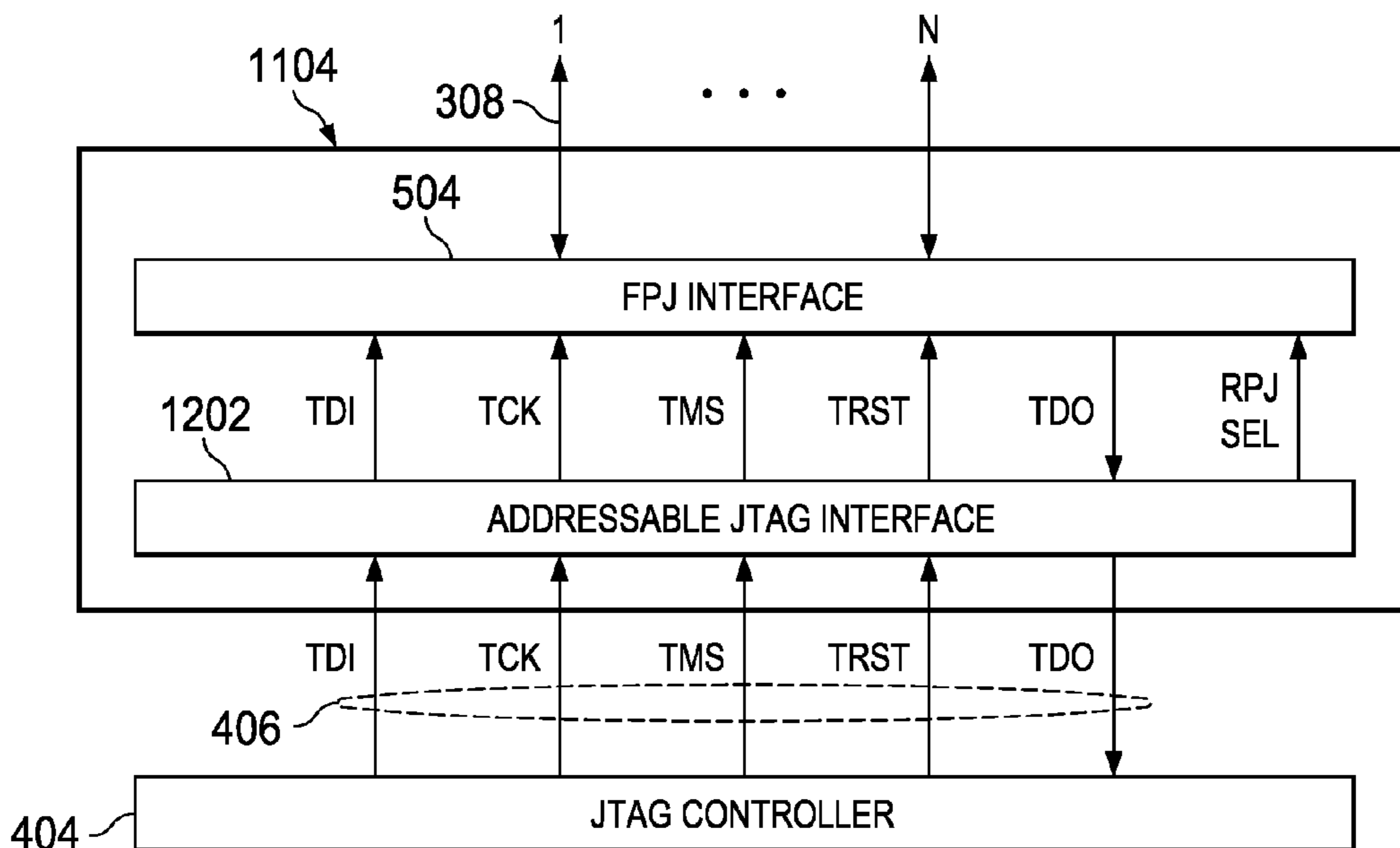
FIG. 12
