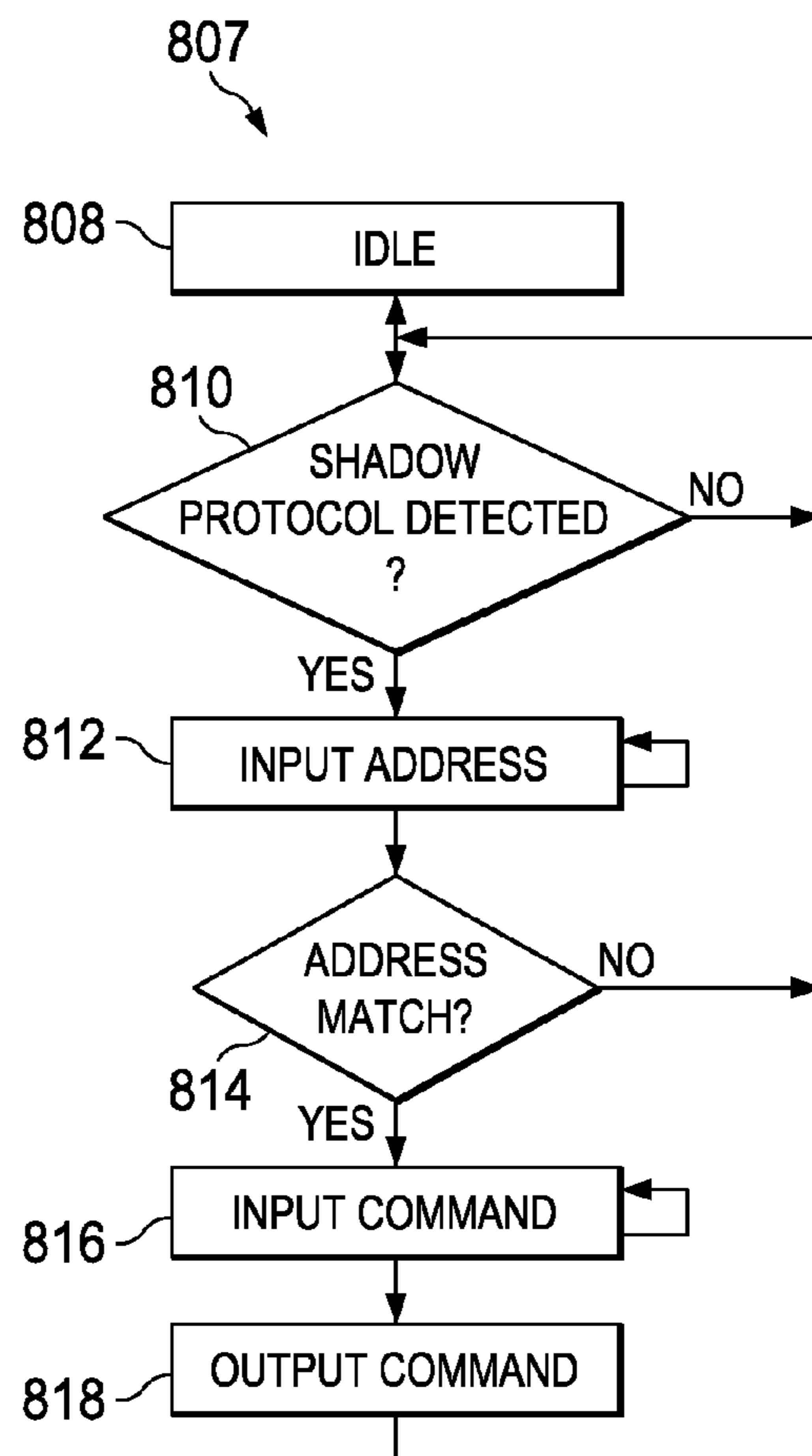
FIG. 8B
