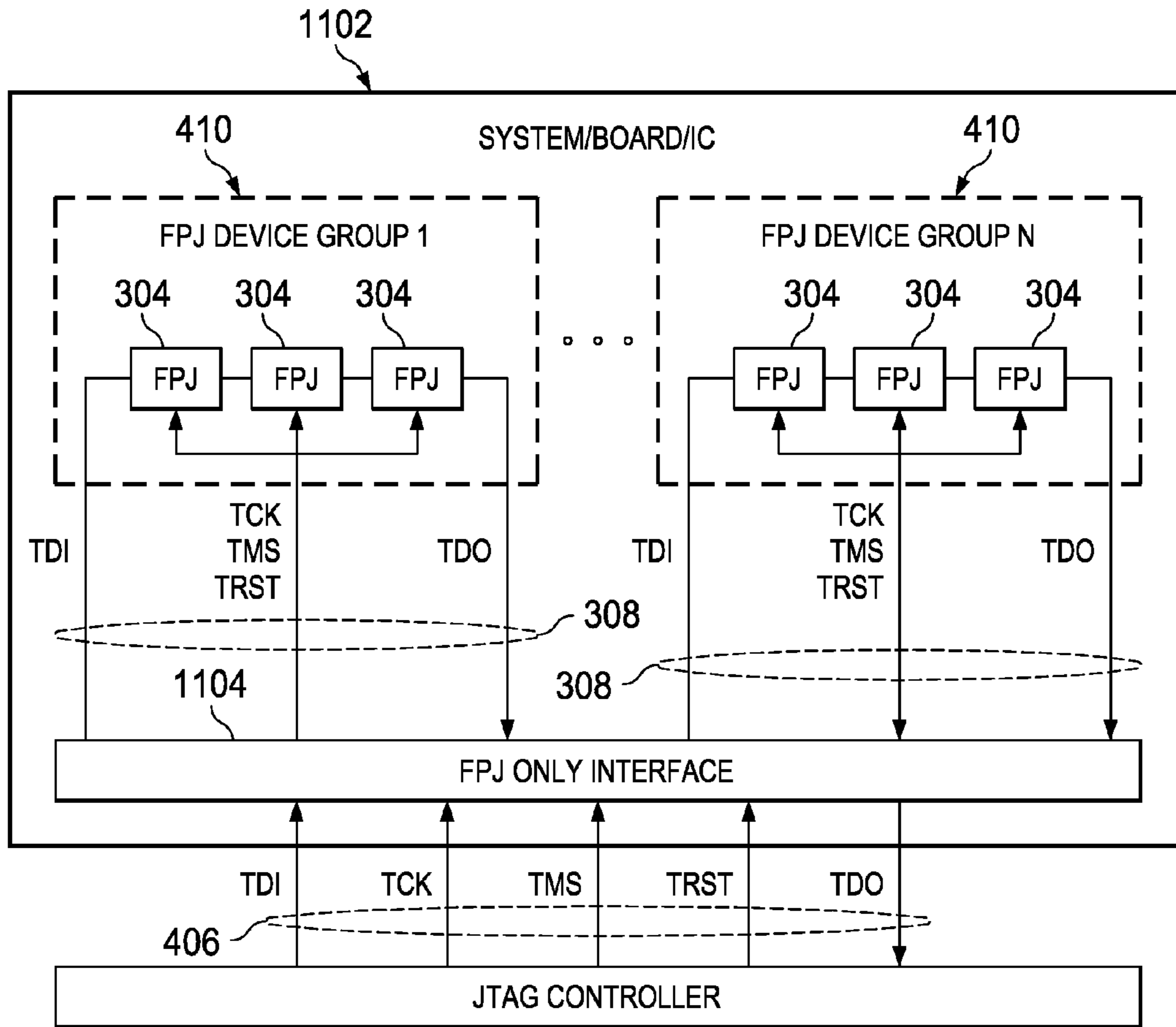
404 FIG. 11
