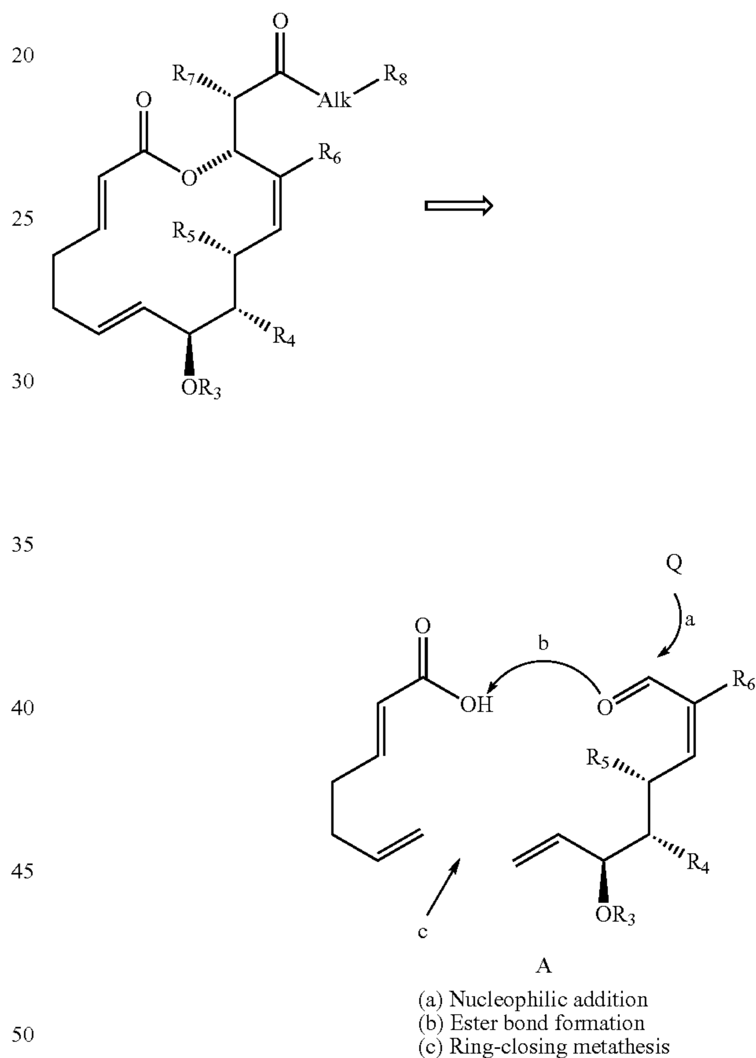
Scheme 1A
