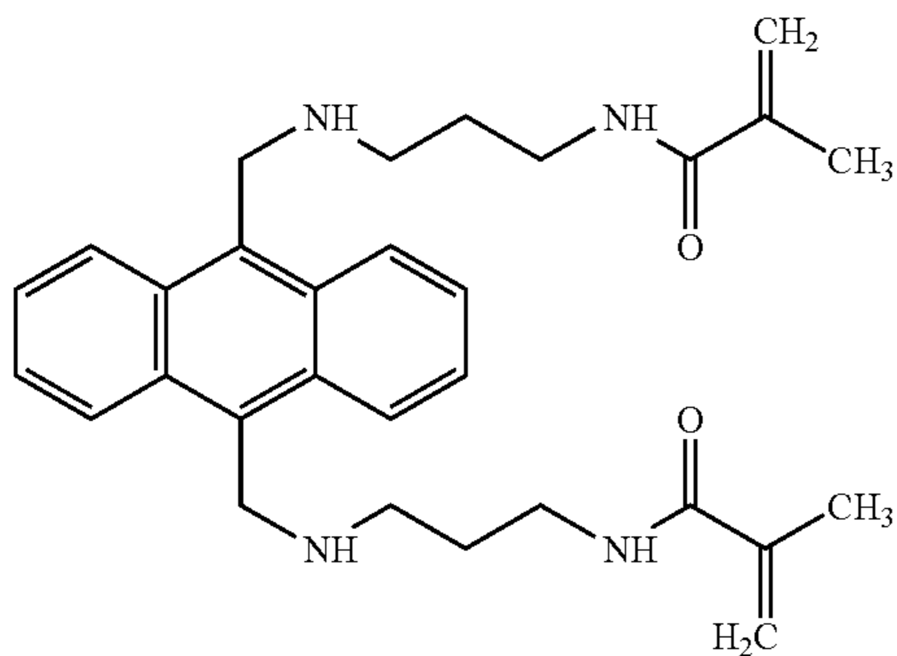
A. 9,10-bis[3-(methacrylamido)propylamino]methyl-anthracene
