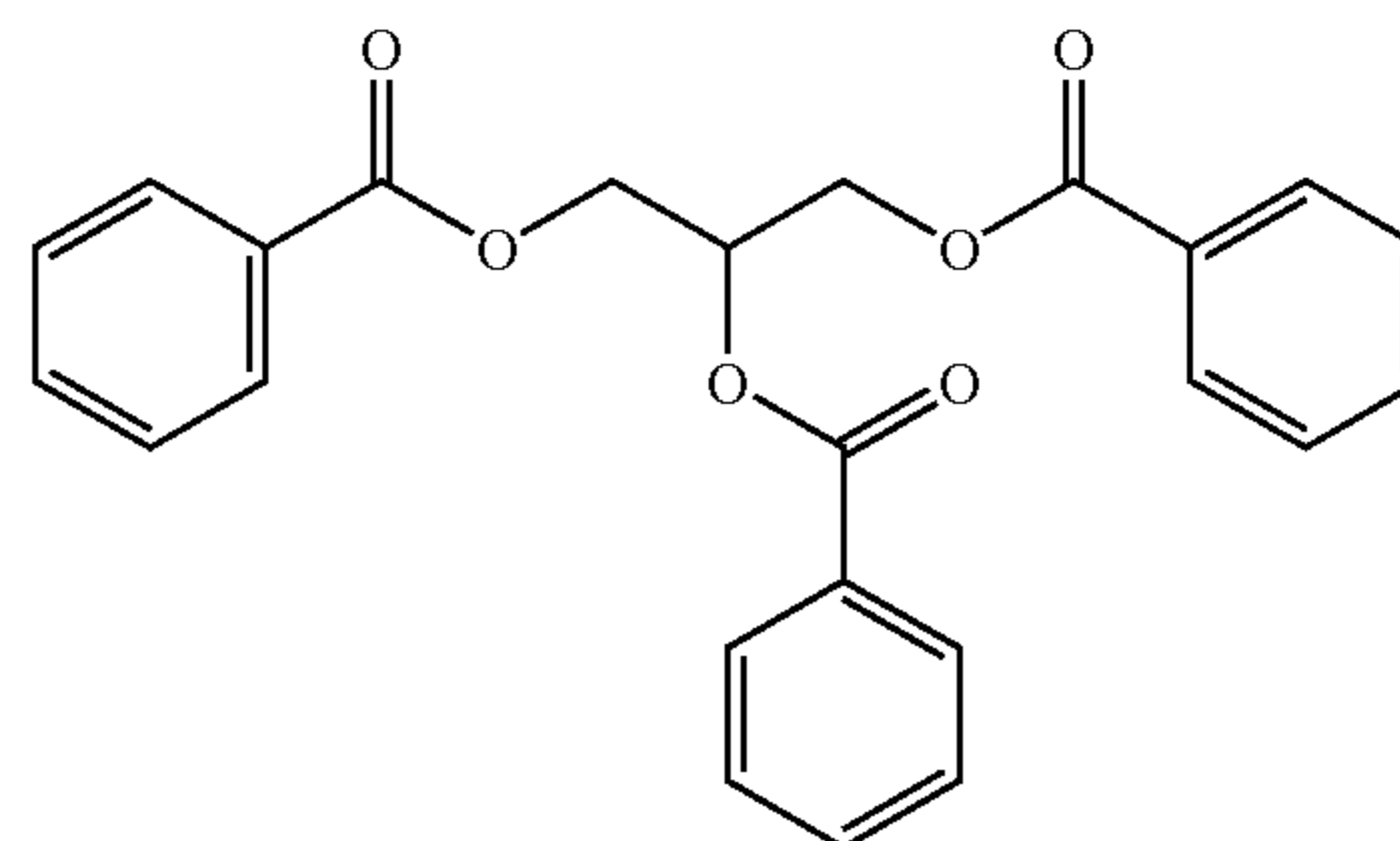
Glycerol Tri-Benzoate
