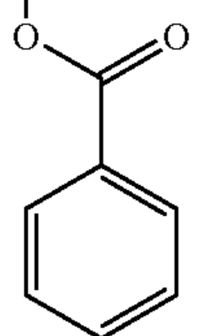
Glycerol Di-Benzoate
