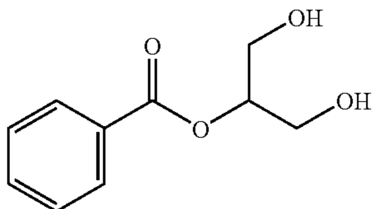
Glycerol Mono-Benzoate
