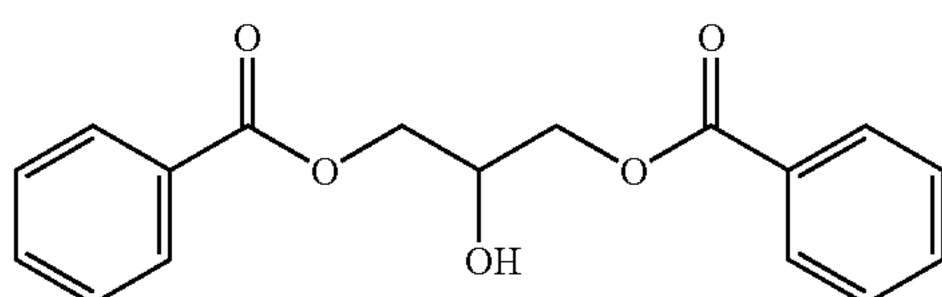
Glycerol Di-Benzoate
