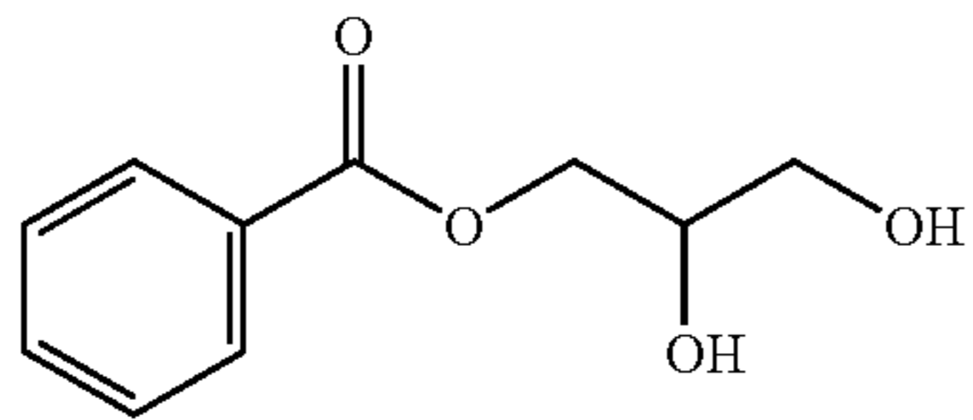
Glycerol Mono-Benzoate
