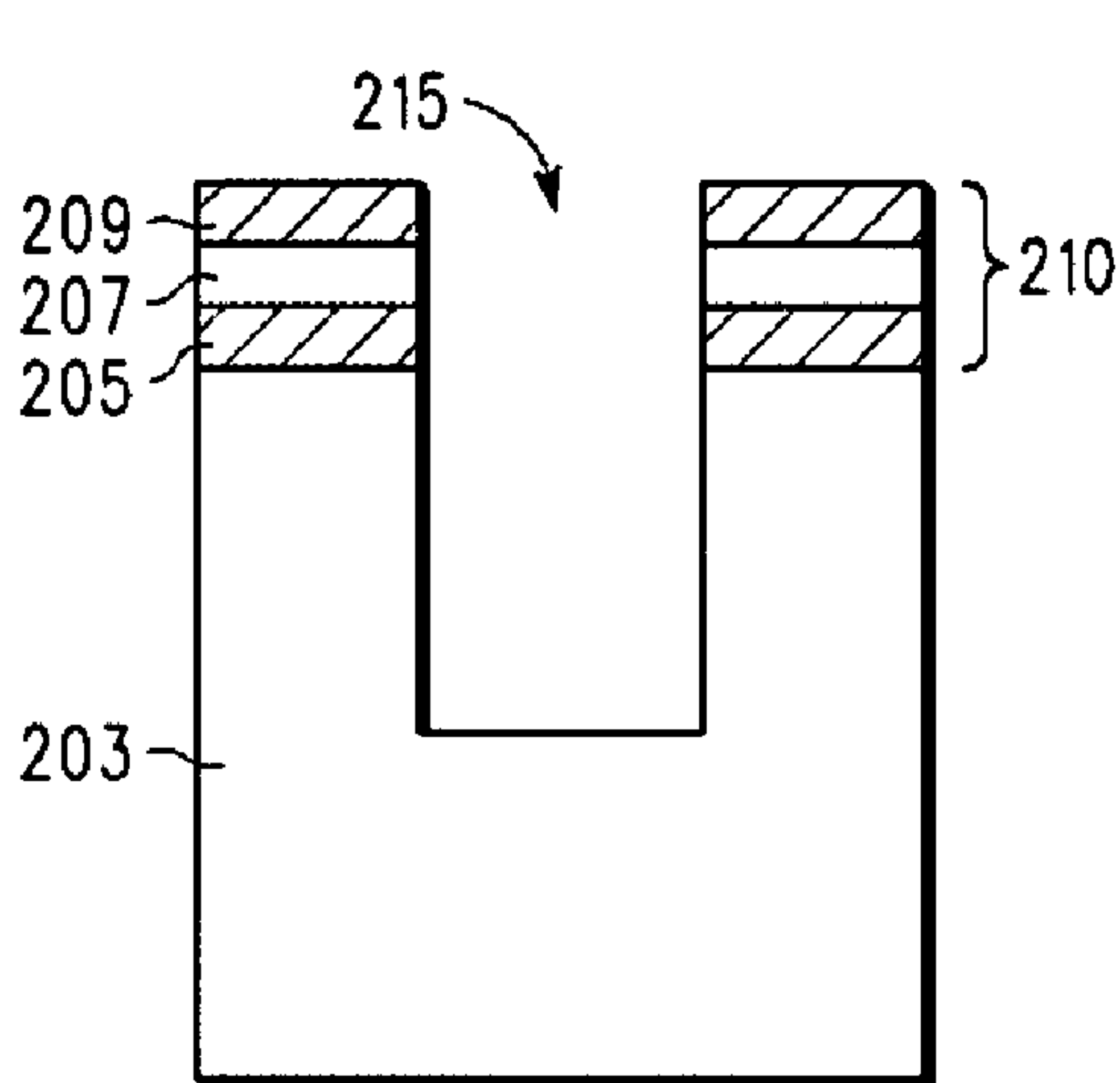
FIG. 8
