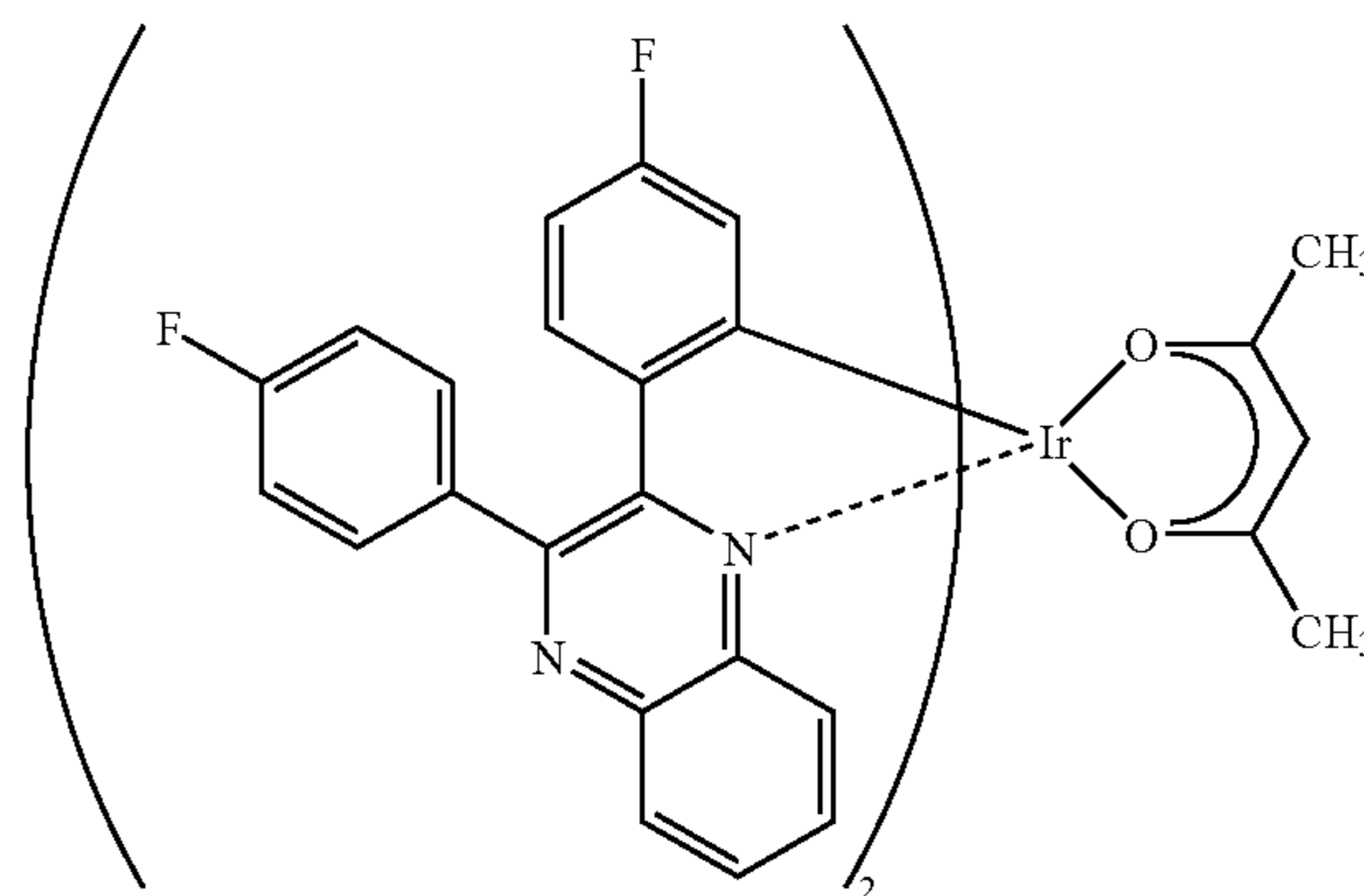
Ir(Fdpq) 2 (acac)
