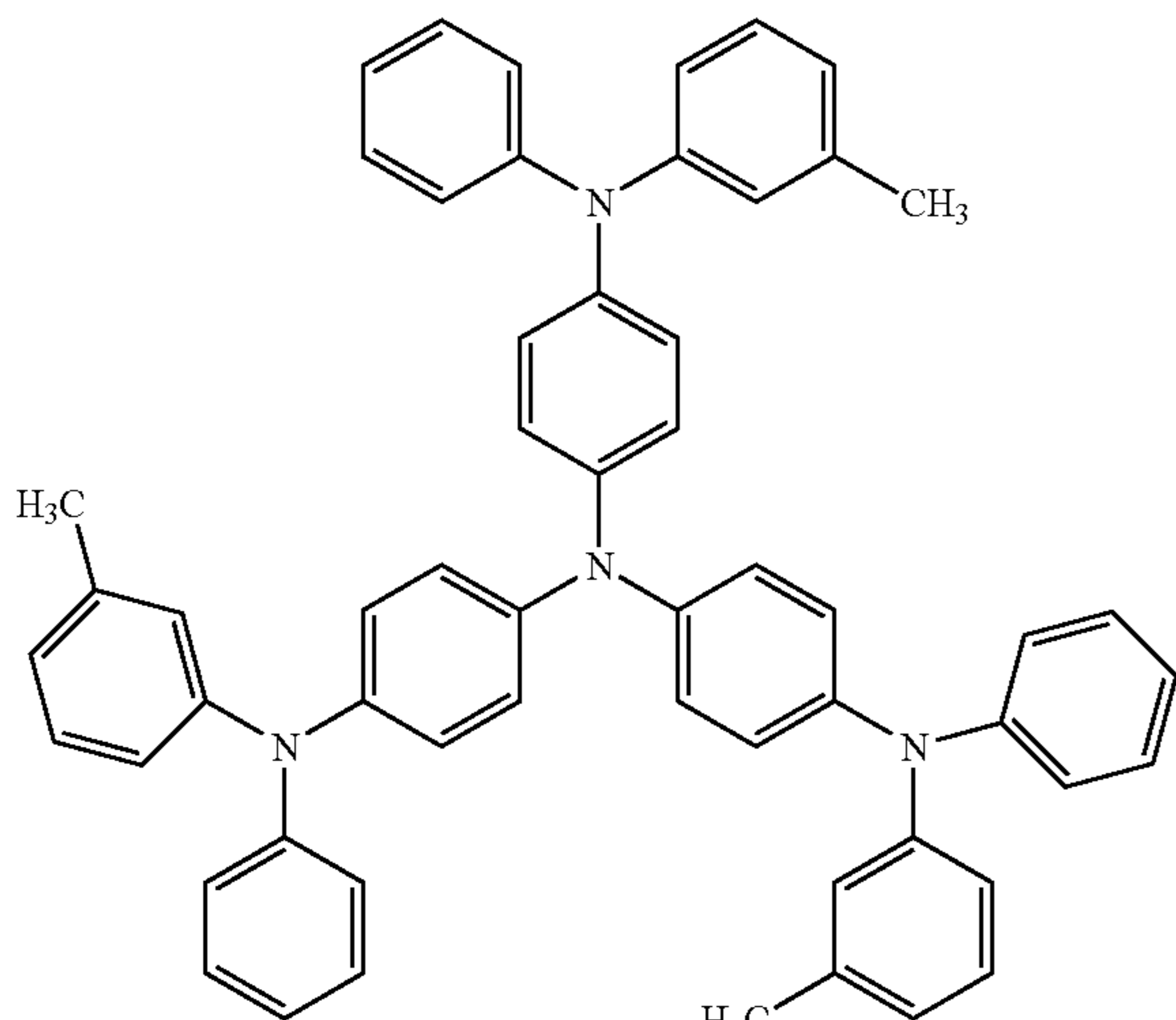
m-MTDATA
