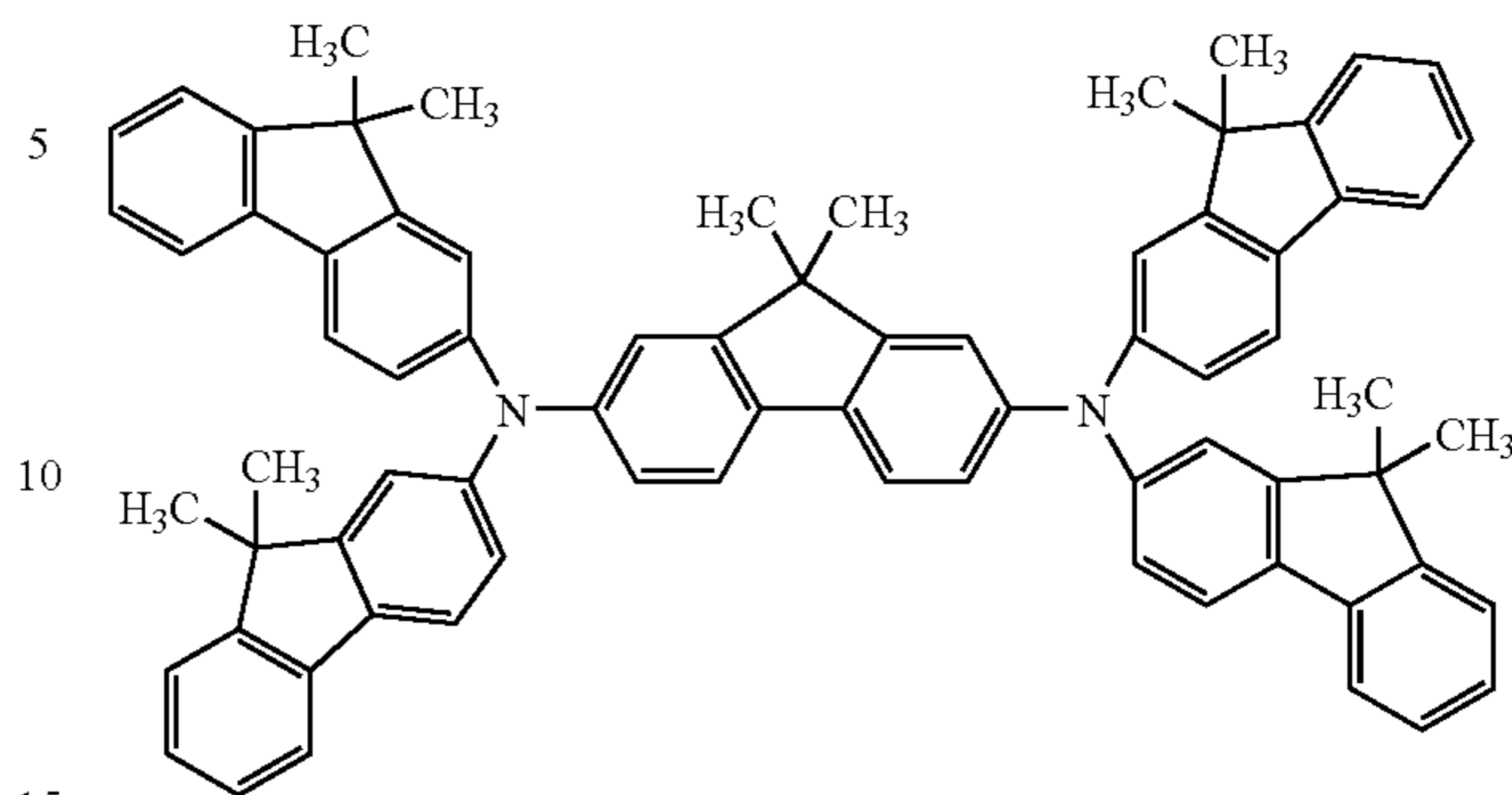
TFLFL
