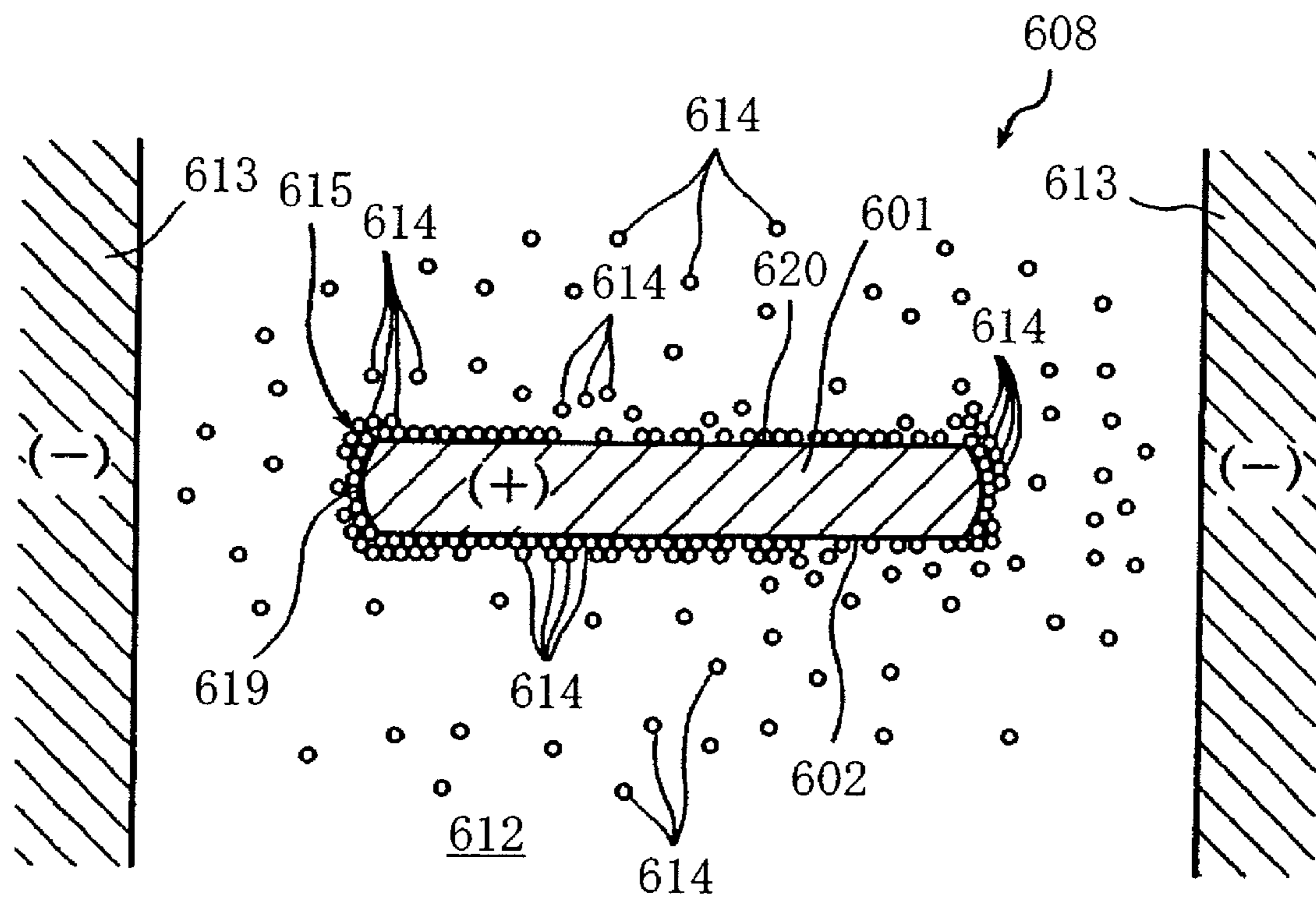
FIG. 86
