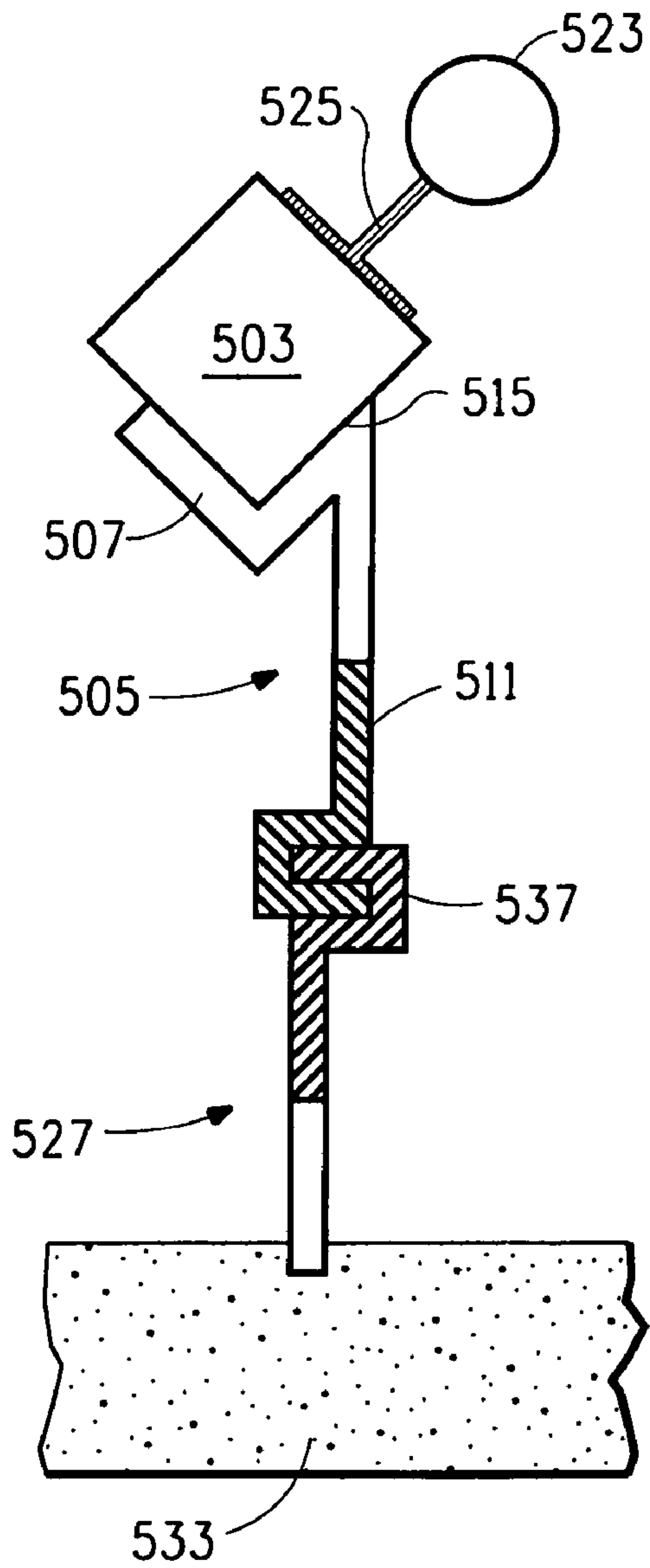
FIG. 6C
