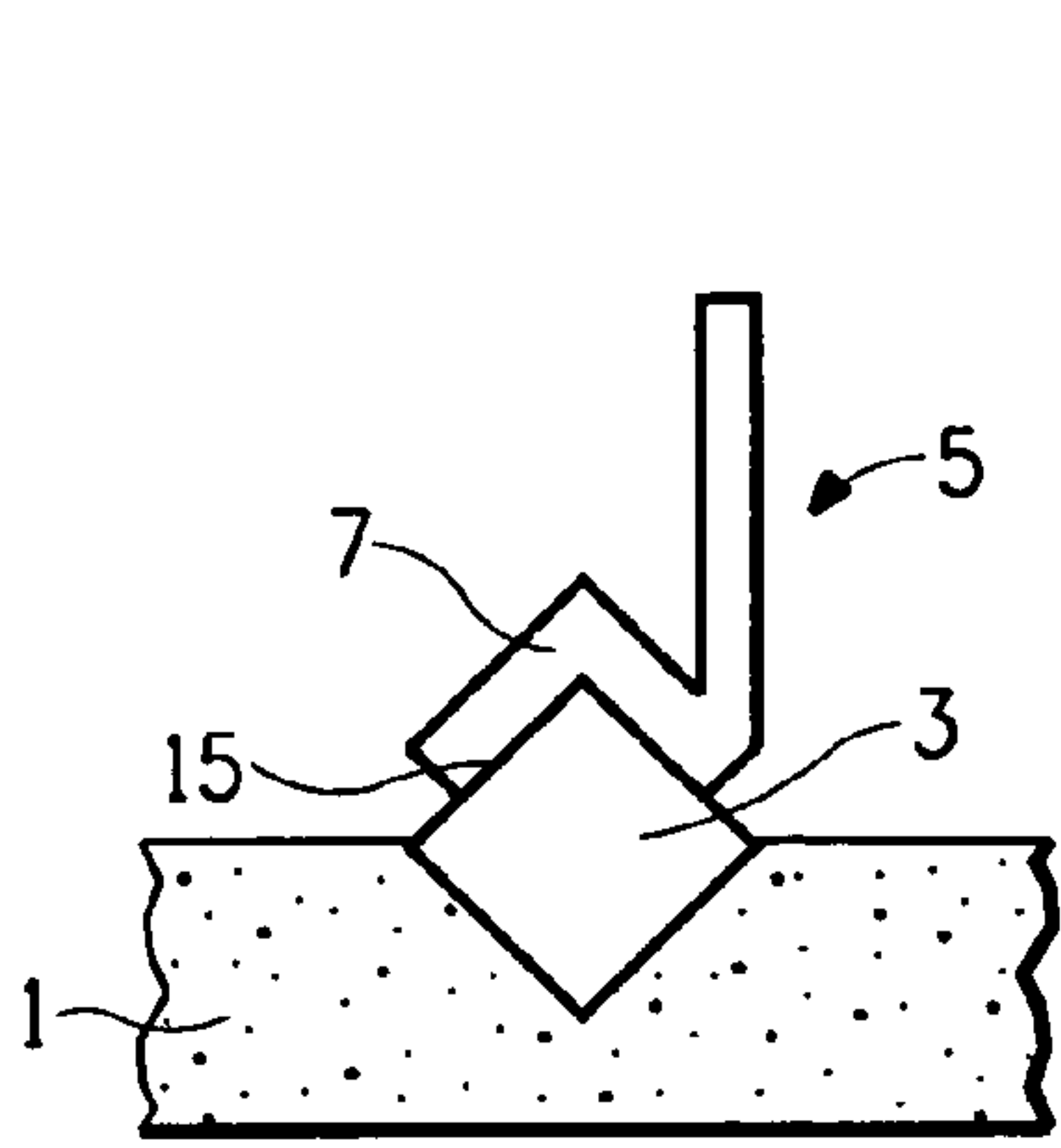
FIG. 1A
