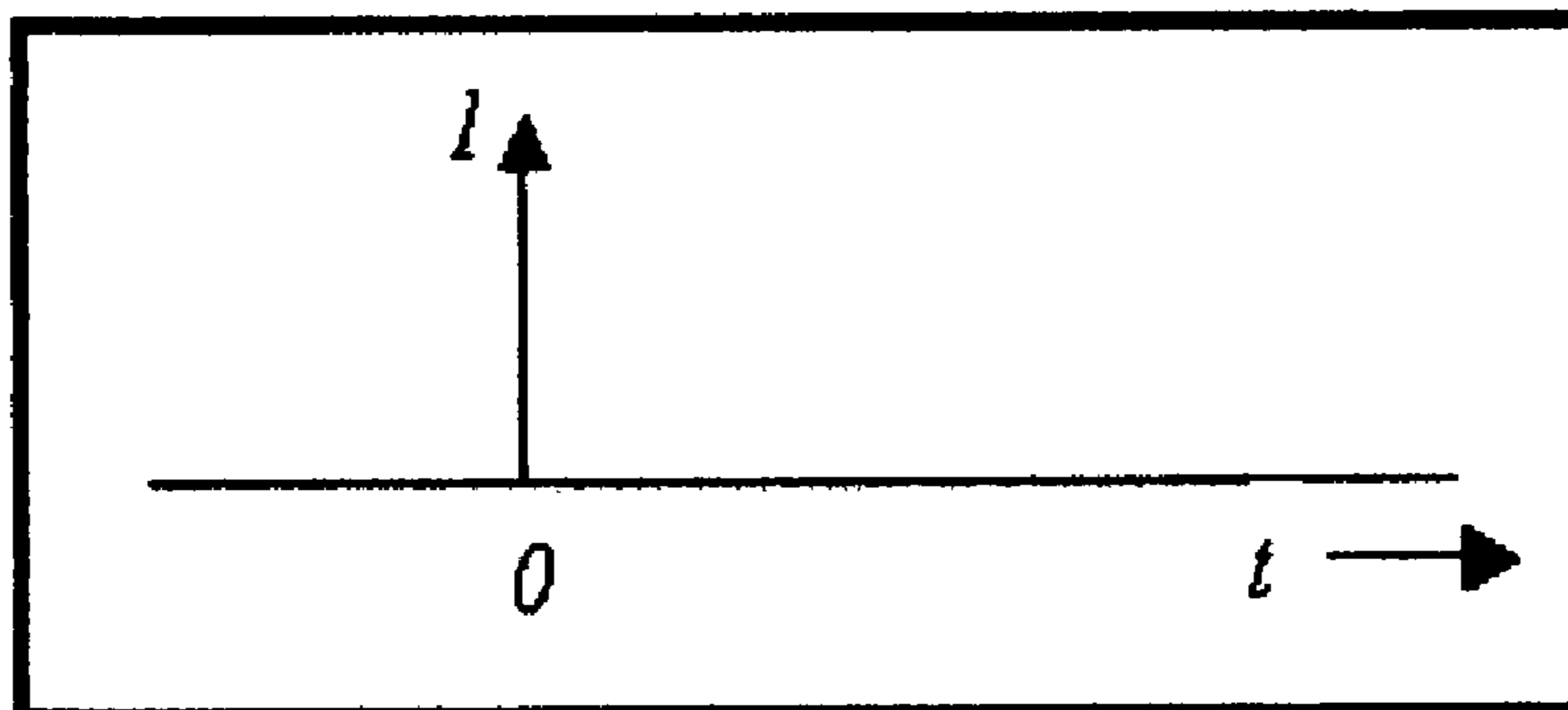
: Dirac Delta Function
