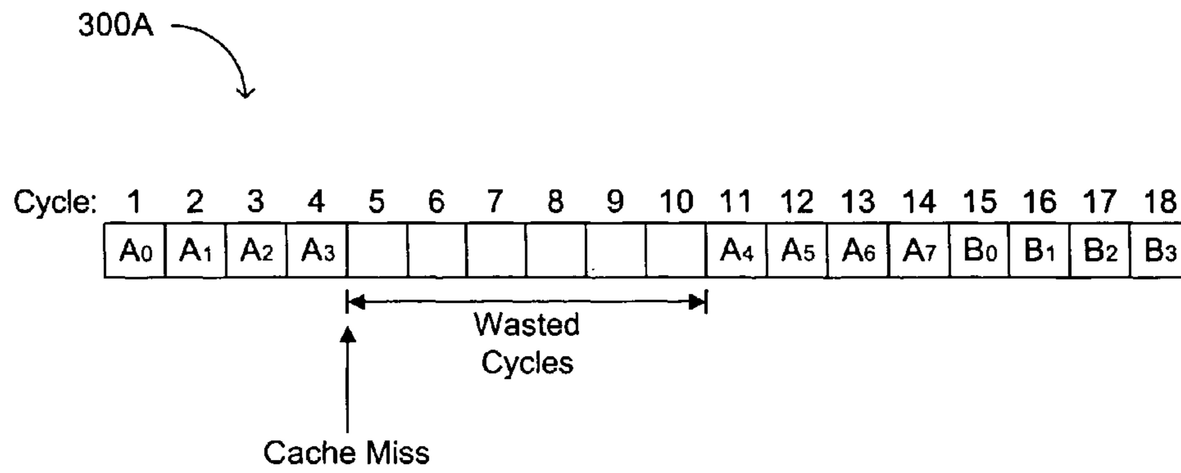
FIG. 3A (conventional)
