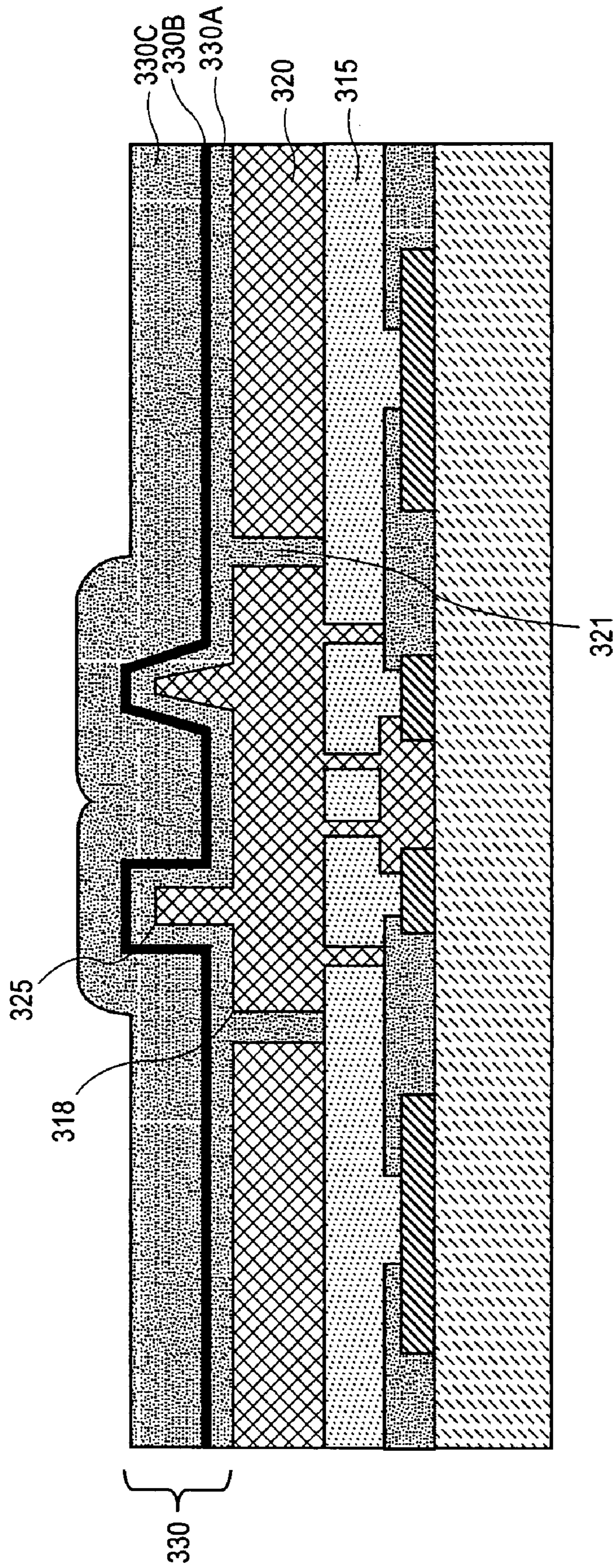
FIG. 3F
