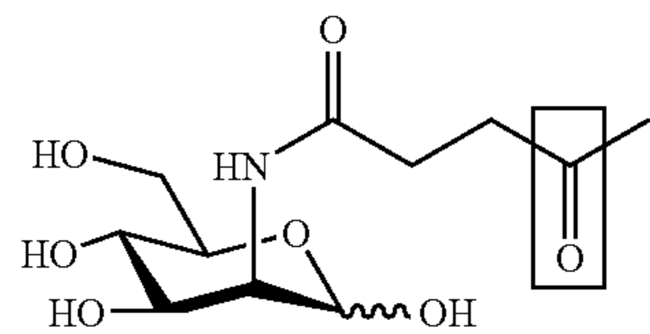
ManLev 3
