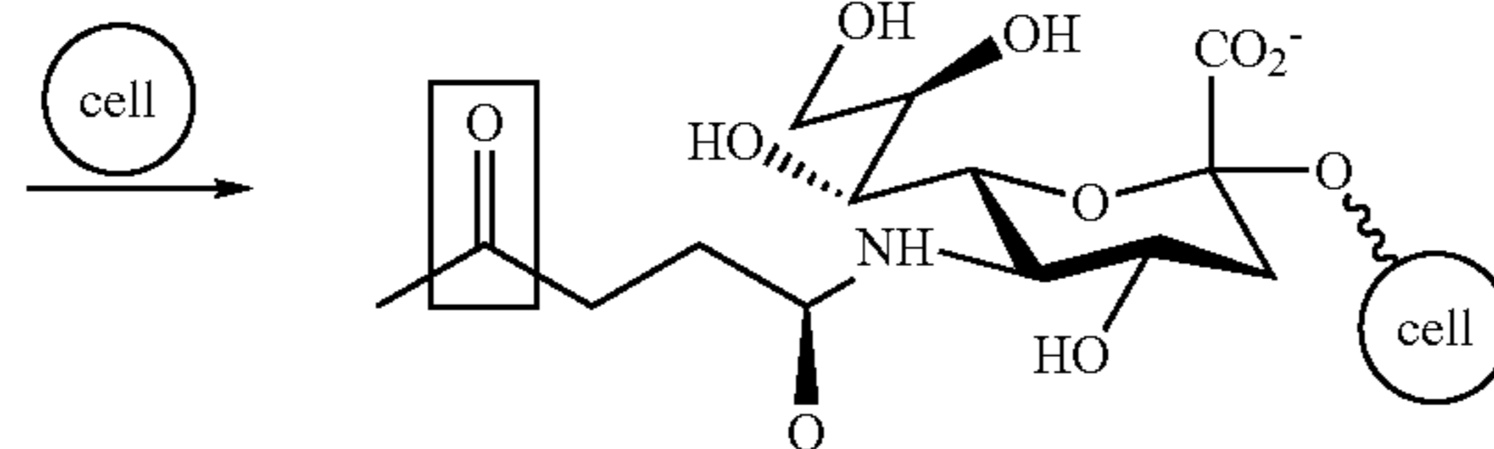
SiaLev 4
