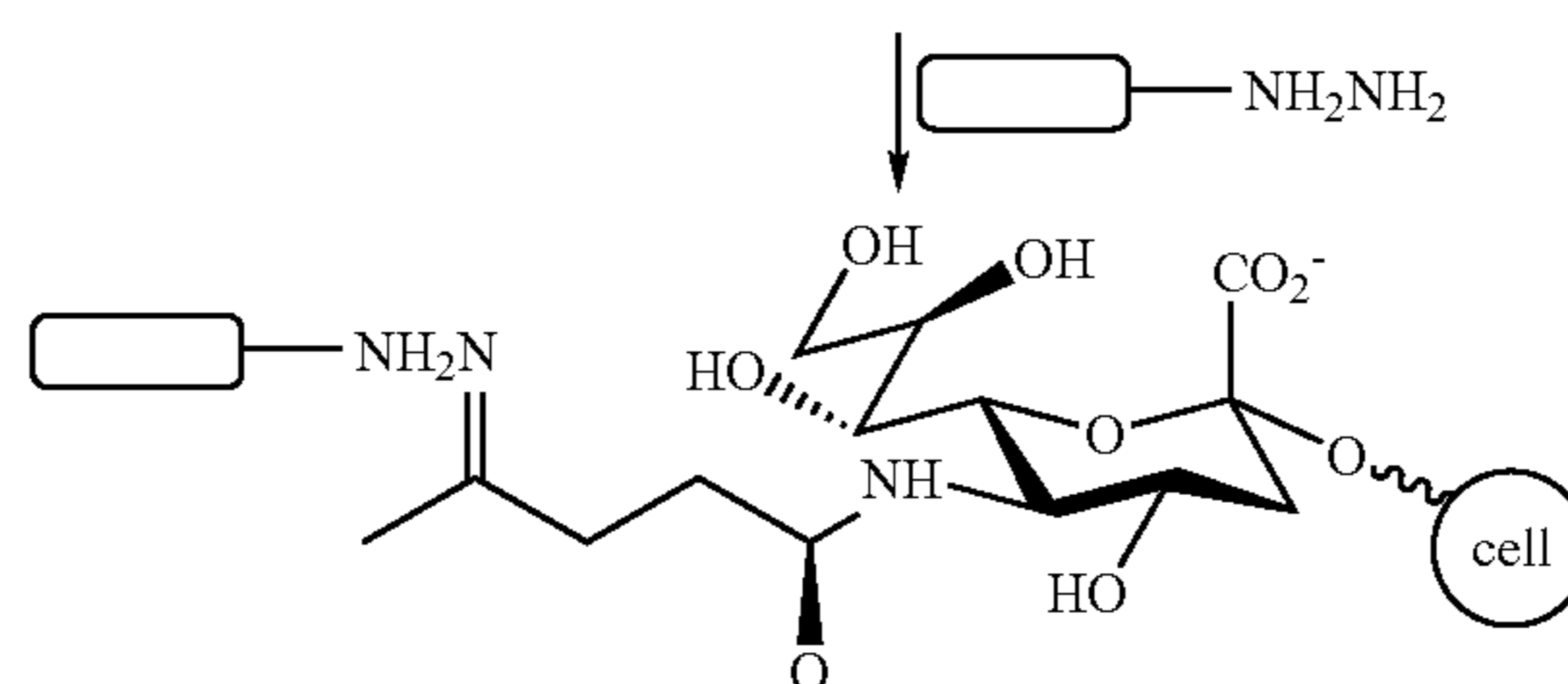
SiaLev 4
