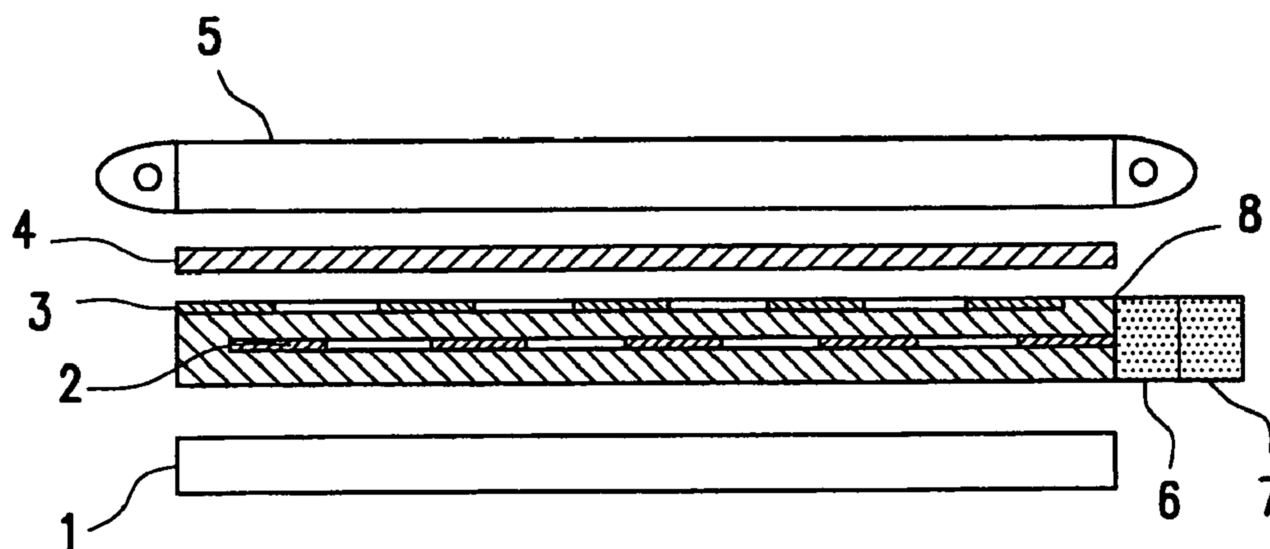
FIG. 3B(PRIOR ART)
