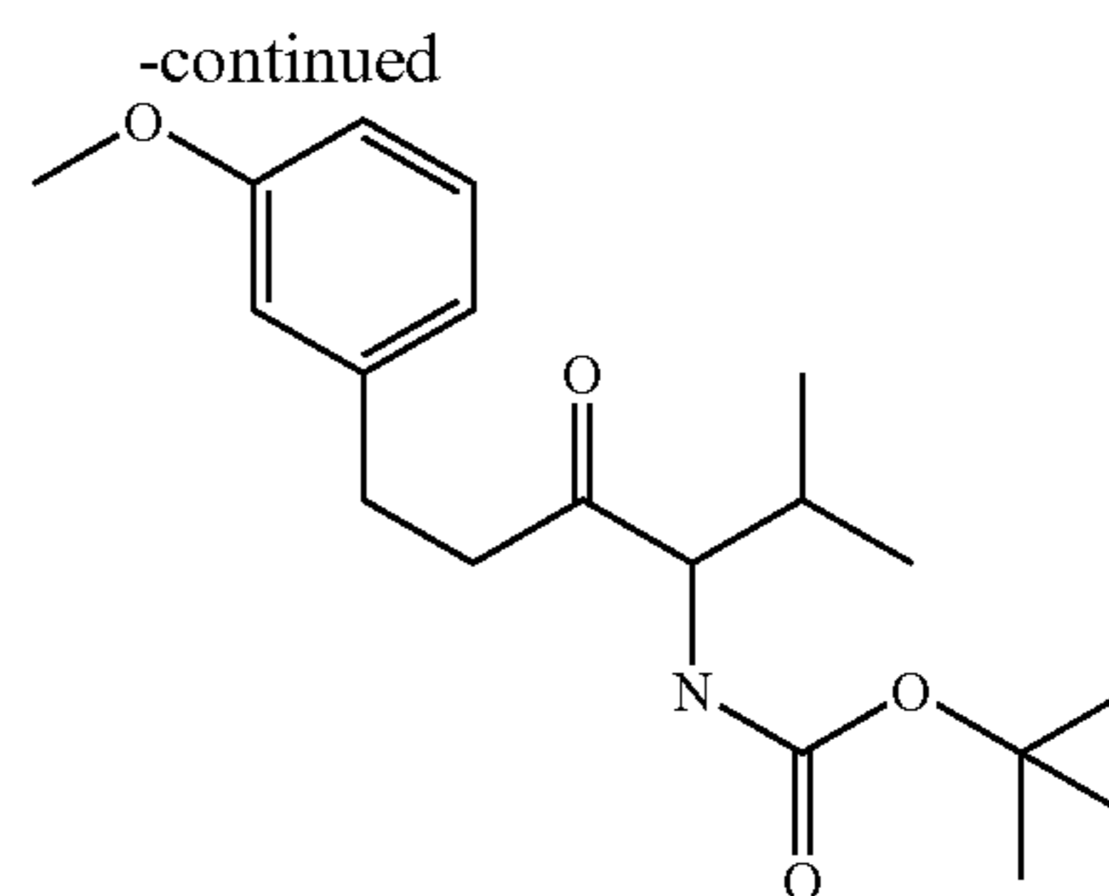
[(2)-(E)-1-Isopropyl-4-(3-methoxy-phenyl)-2-oxo-butyl]-carbamic acid tert-butyl ester
