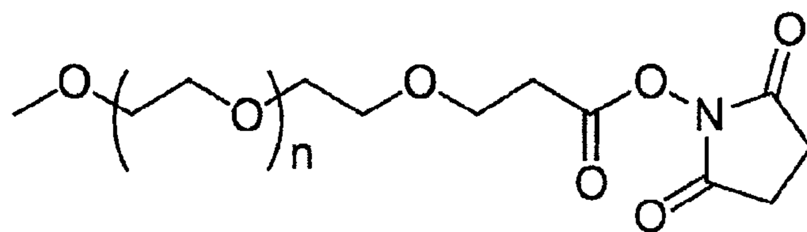
mPEG-SPA
