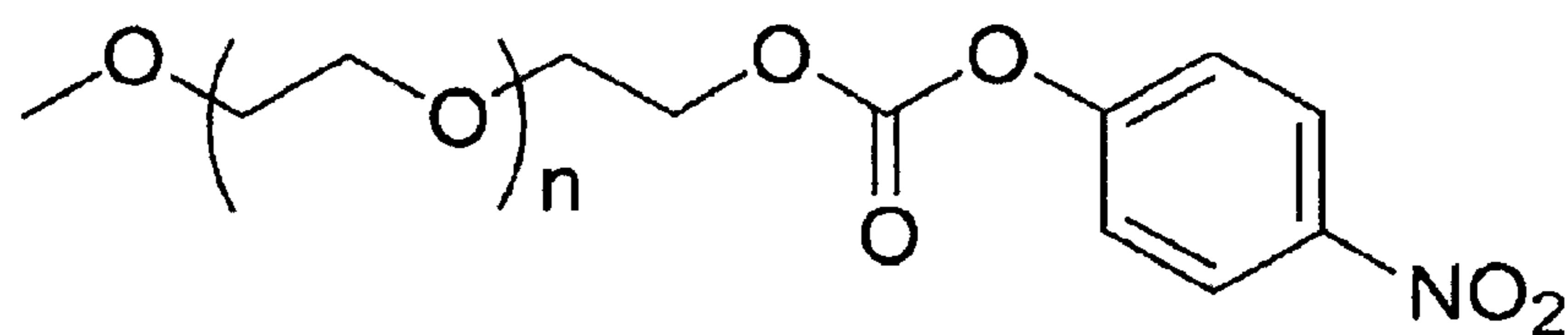
mPEG-NPC
