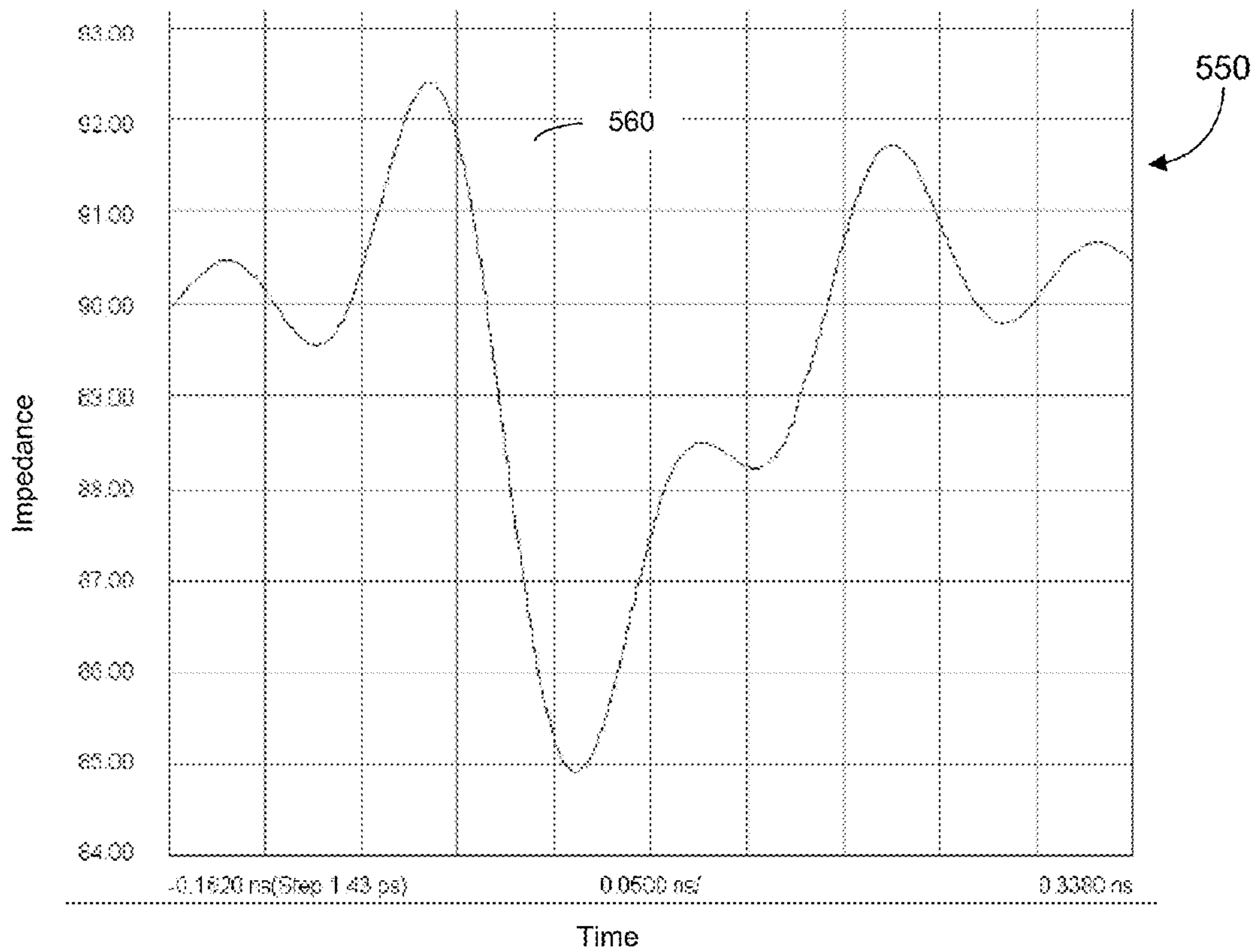
FIG. 5B
