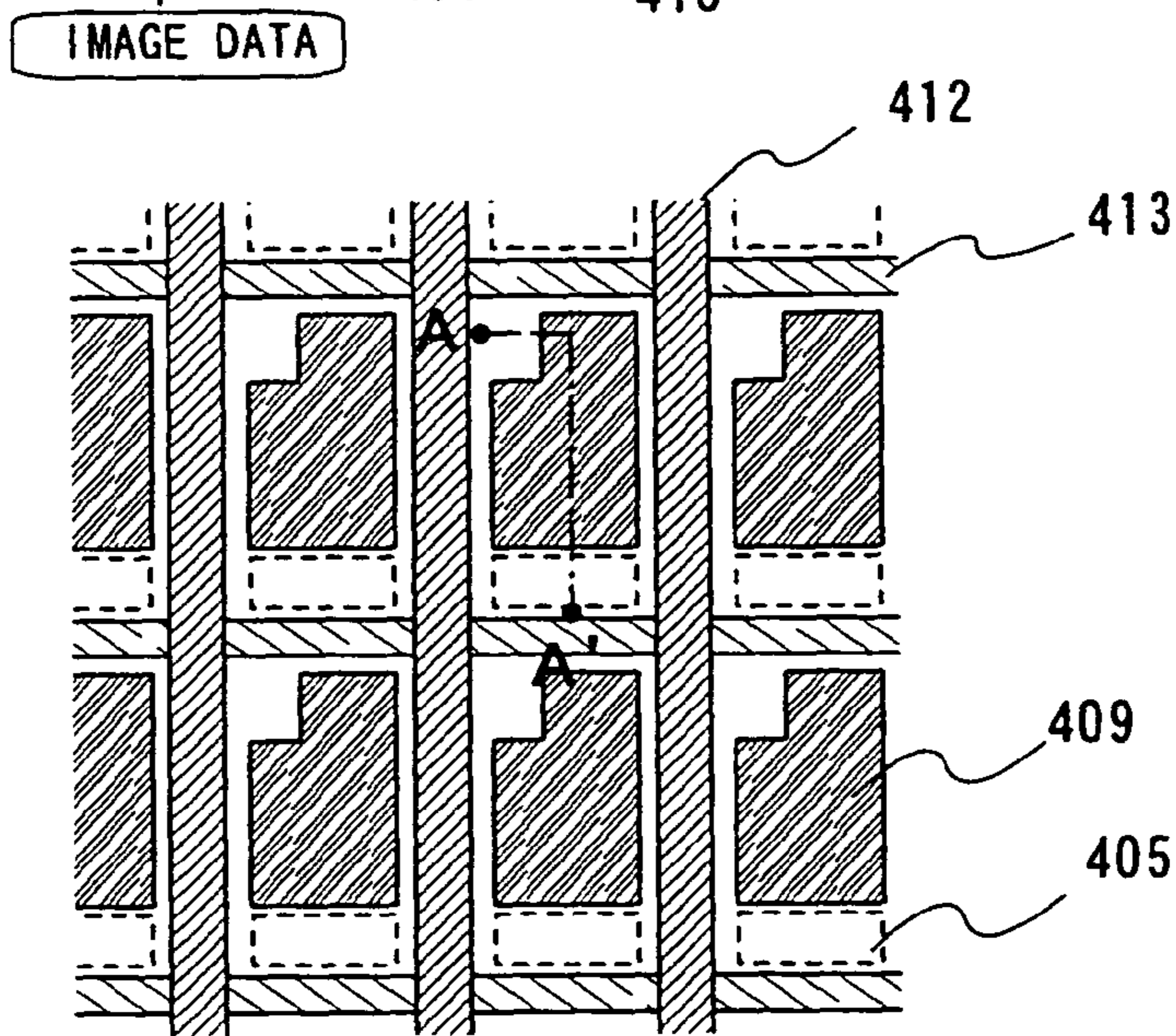
FIG. 11B
