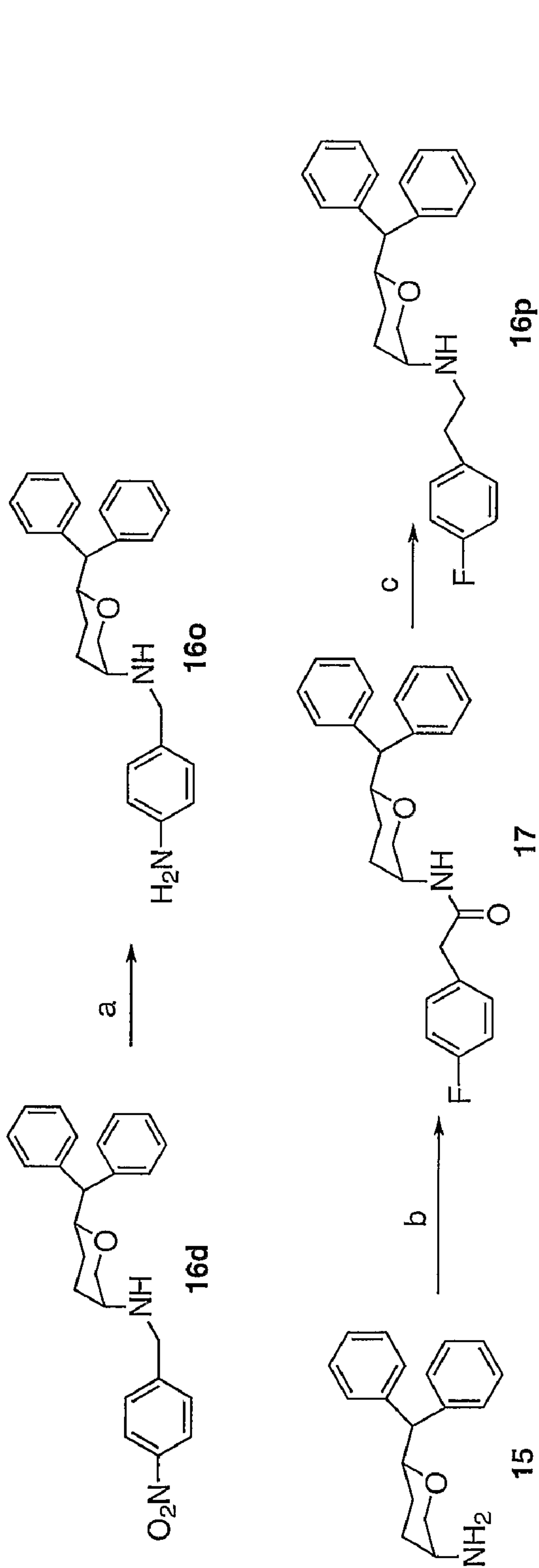
(a) \text{SnCl}_2 \cdot 2\text{H}_2\text{O} / \text{EtOH} / \text{EtOAc} (b) 4-fluorophenylacetyl chloride, \text{Et}_3\text{N} / \text{CH}_2\text{Cl}_2 (d) \text{NaBH}_4 , \text{BF}_3 \cdot \text{Et}_2\text{O} / \text{THF}
