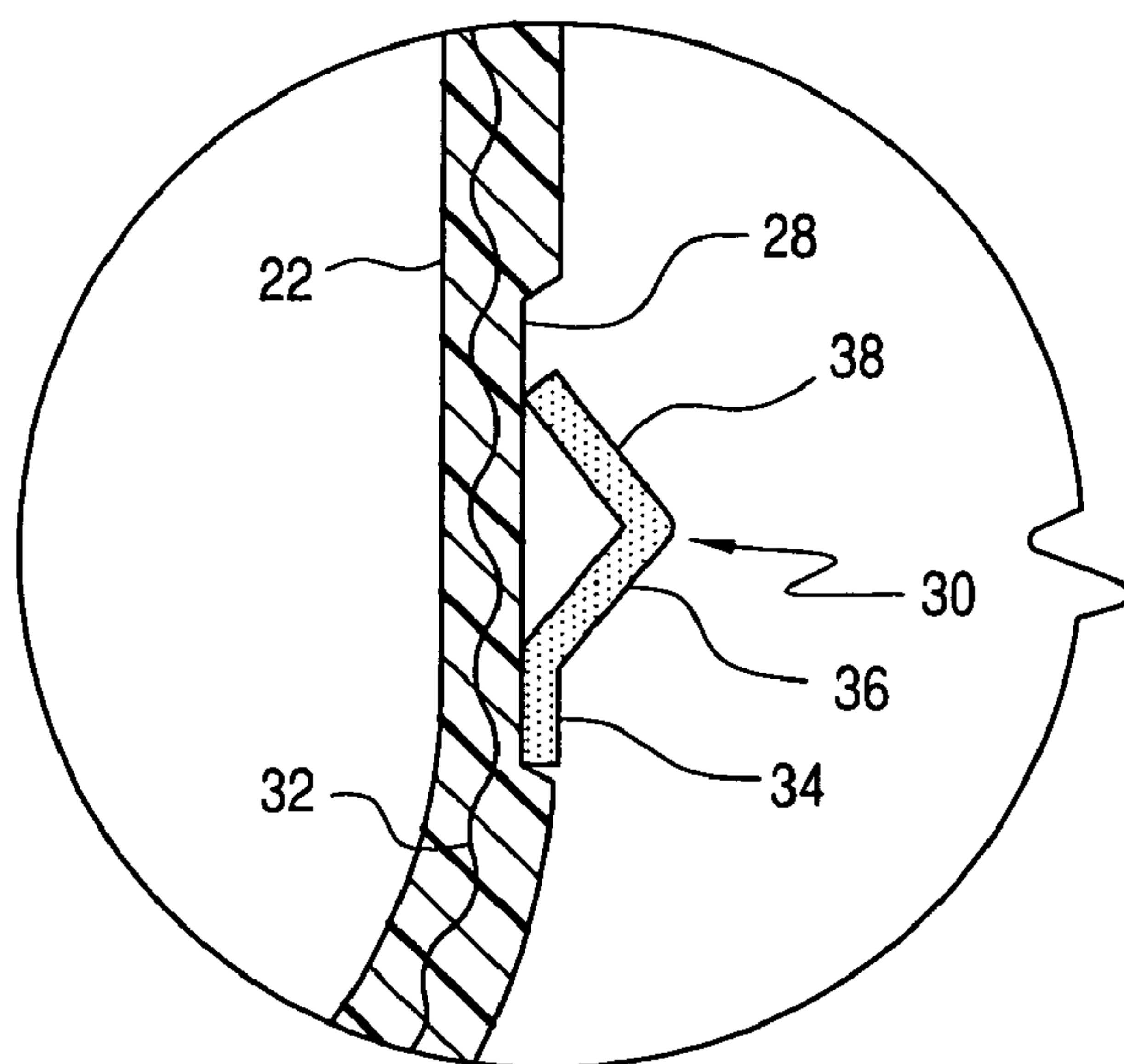
FIG. 18
