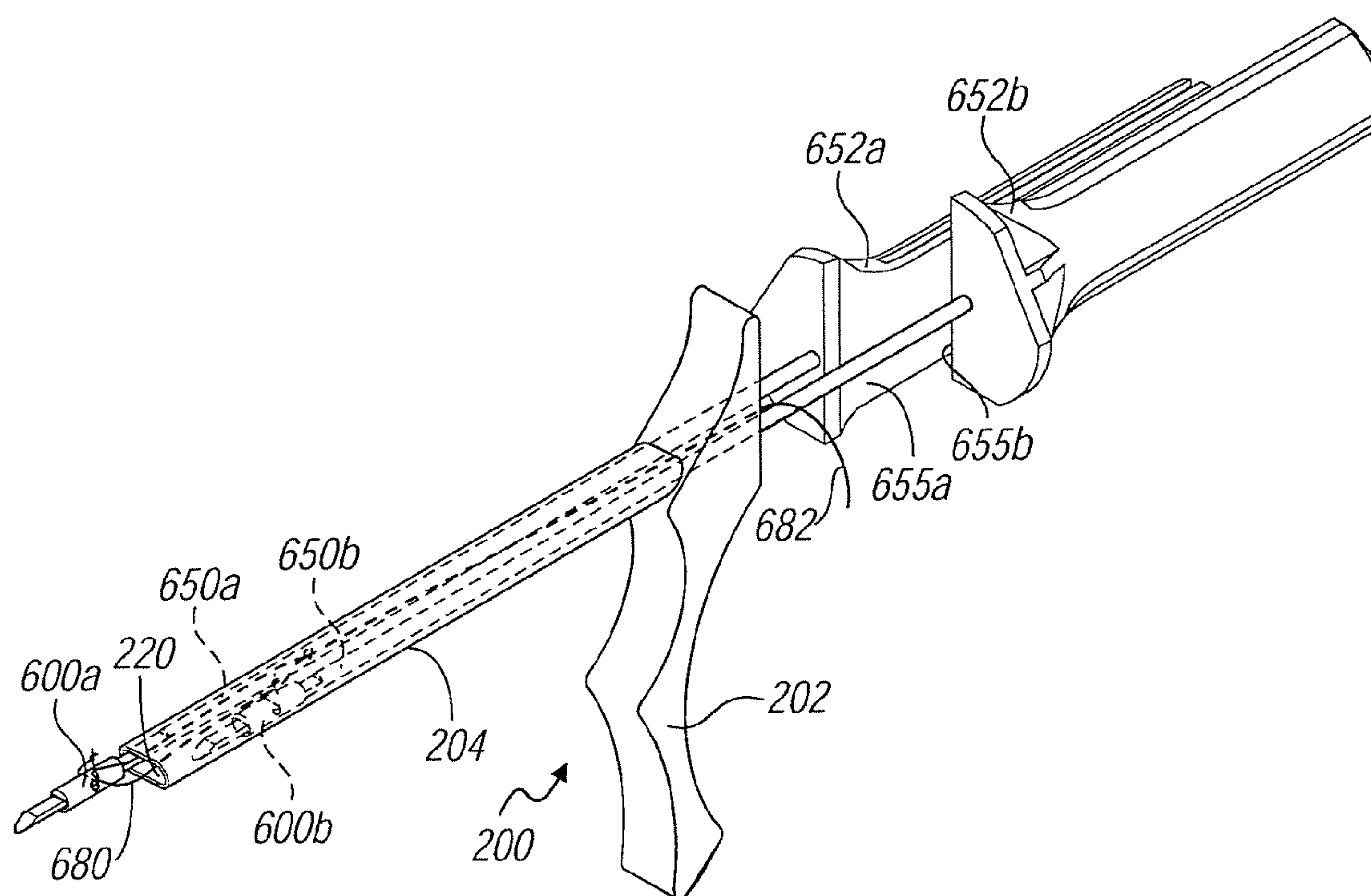
FIG. 26B
