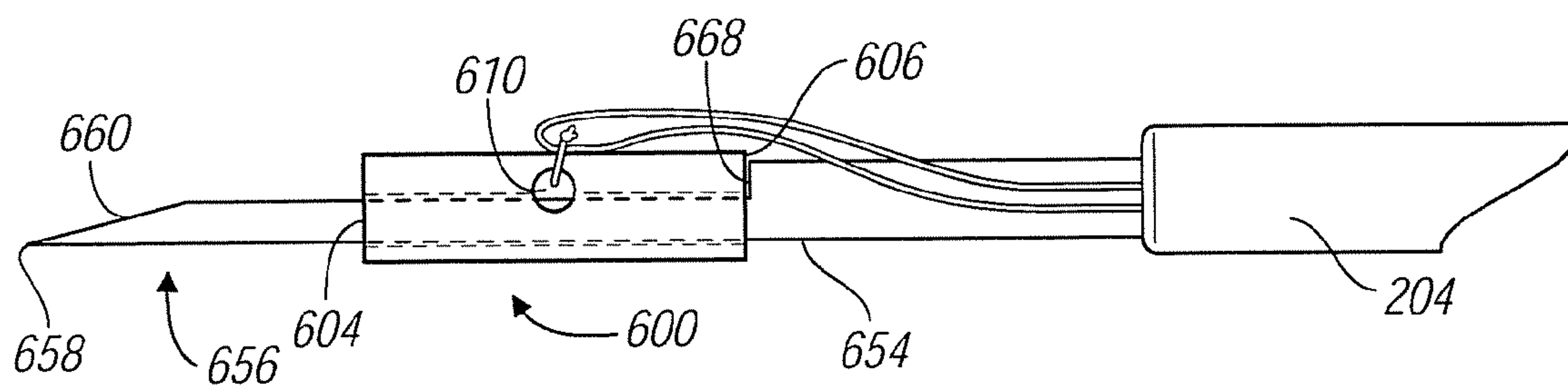
FIG. 18
