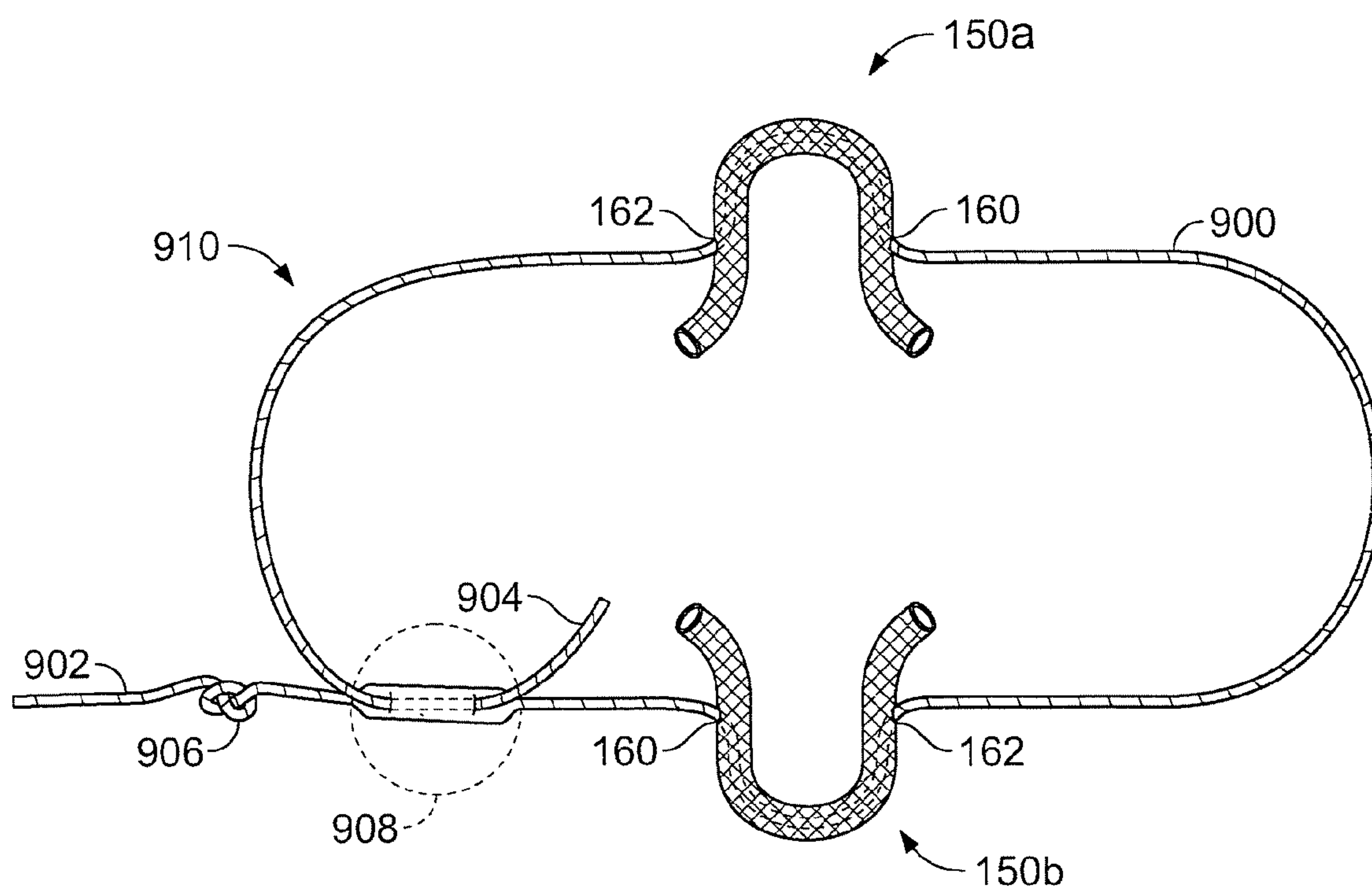
FIG. 35
