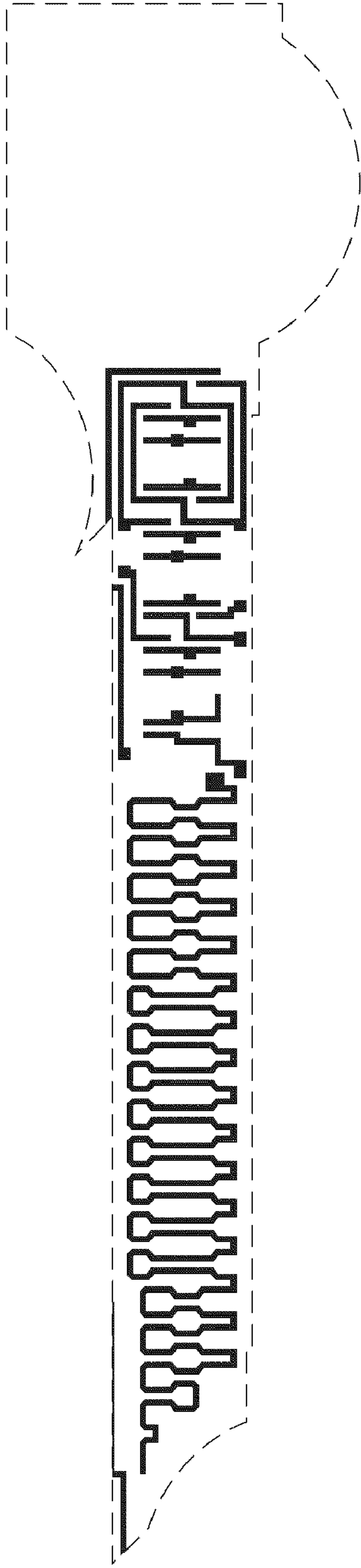
Poly mask
