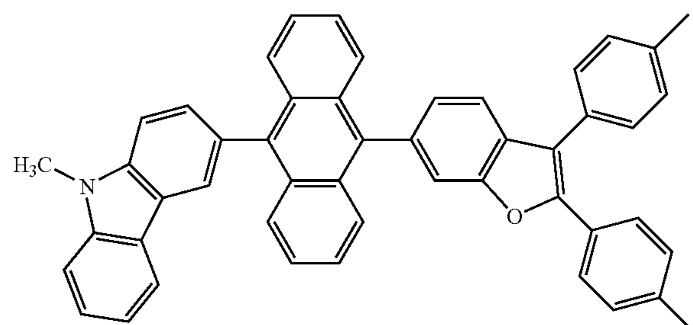
<Formula 47>
