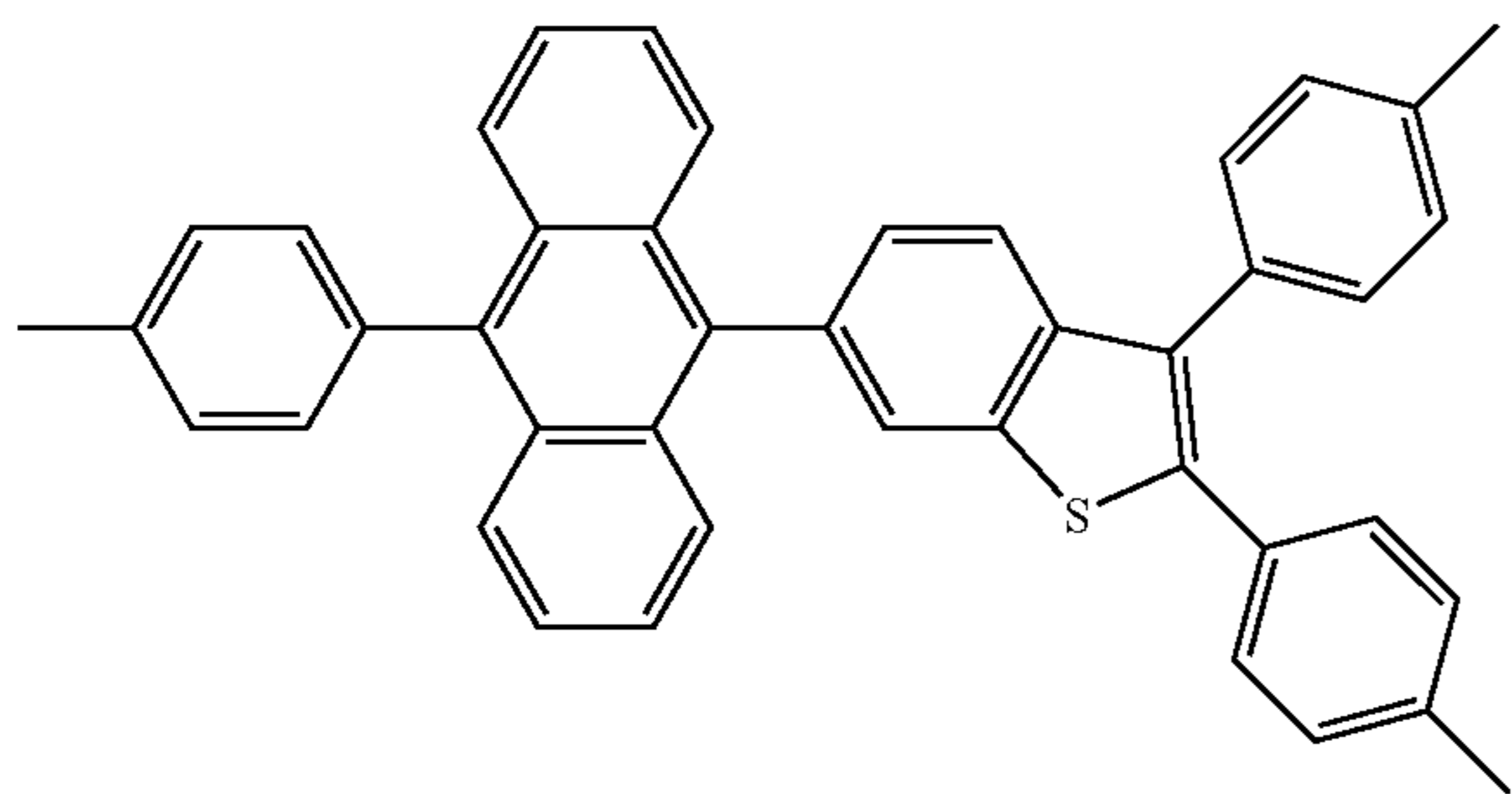
&lt;Formula 4&gt;
