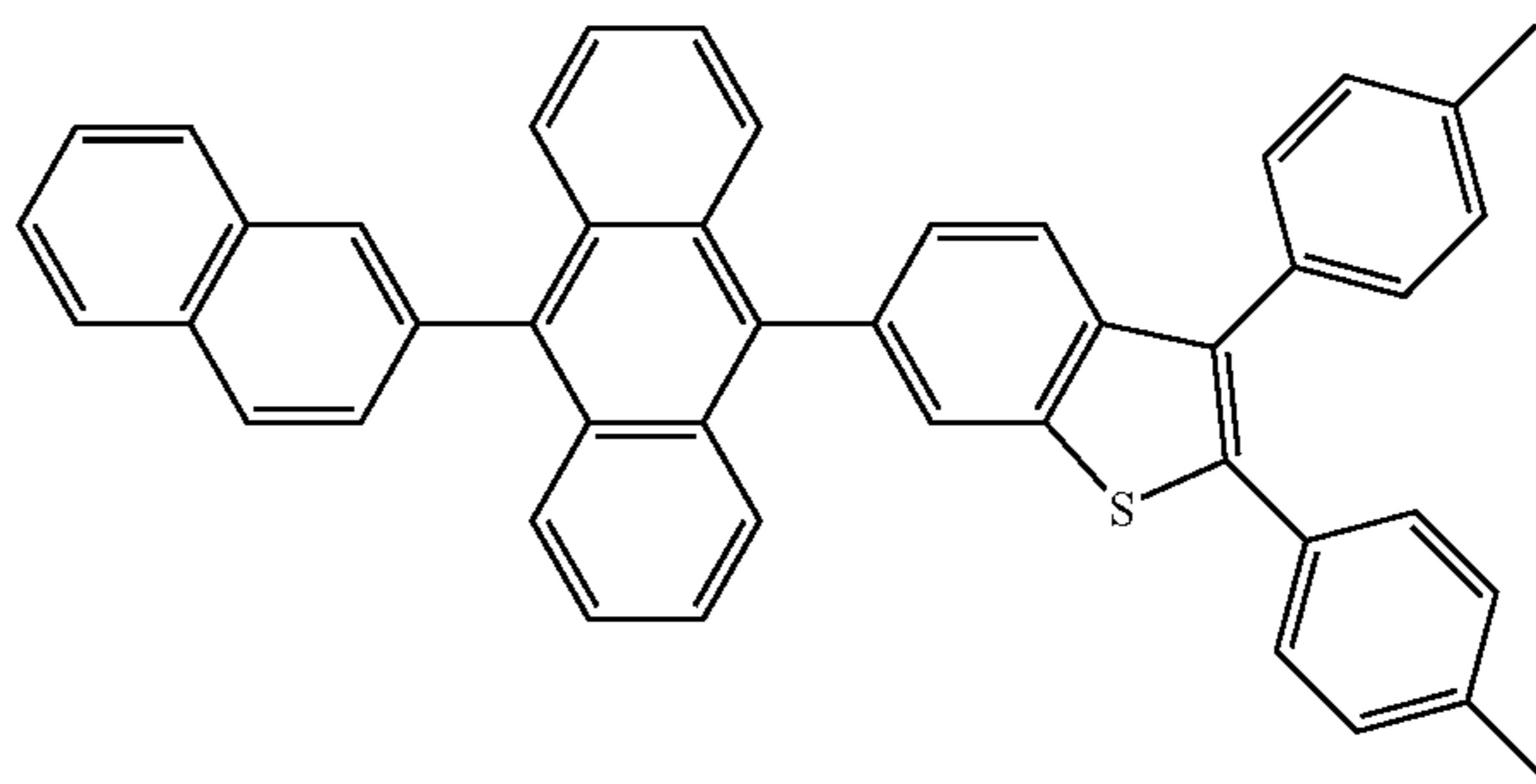
&lt;Formula 5&gt;
