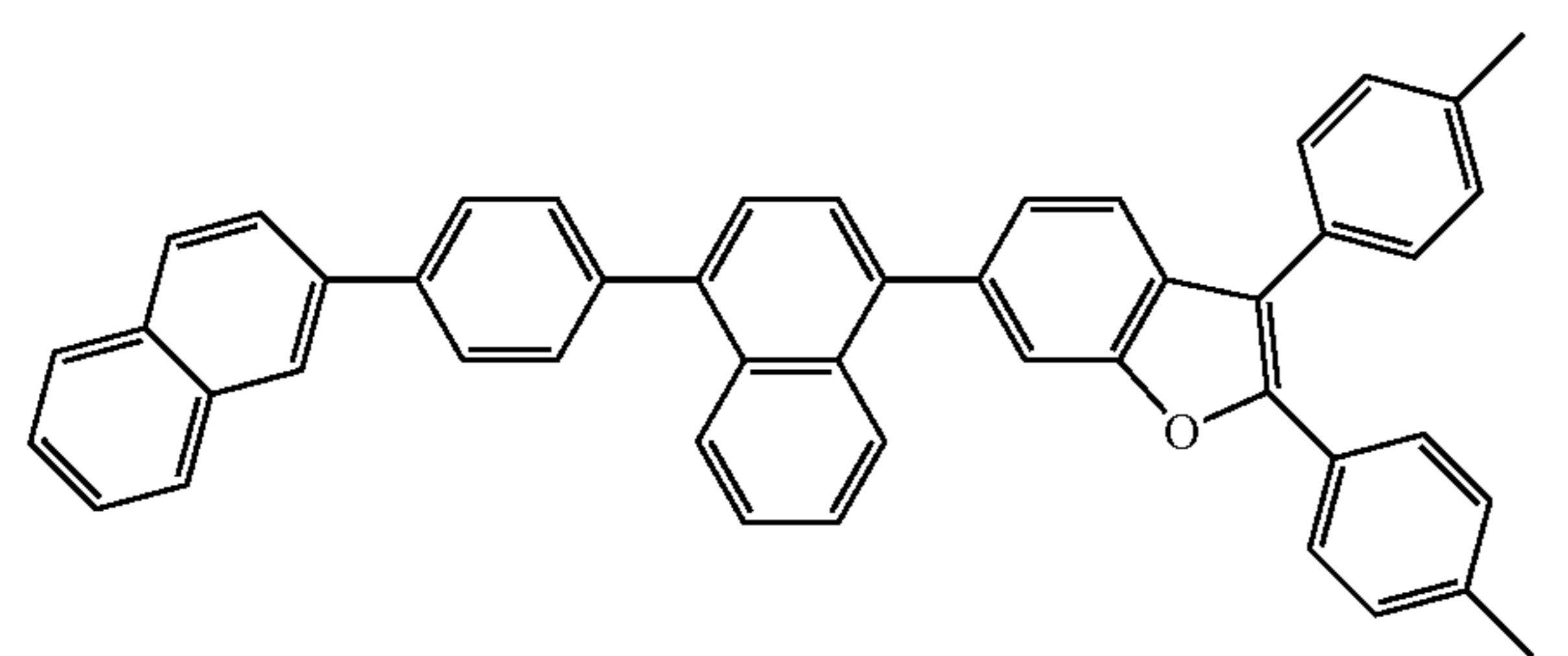
<Formula 53>
