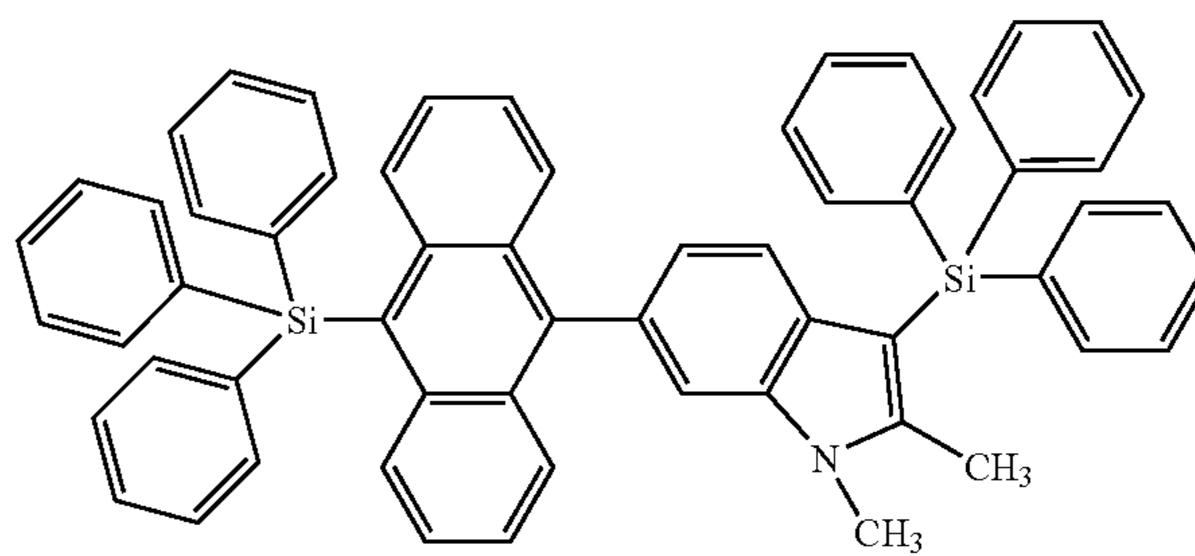
<Formula 66>
