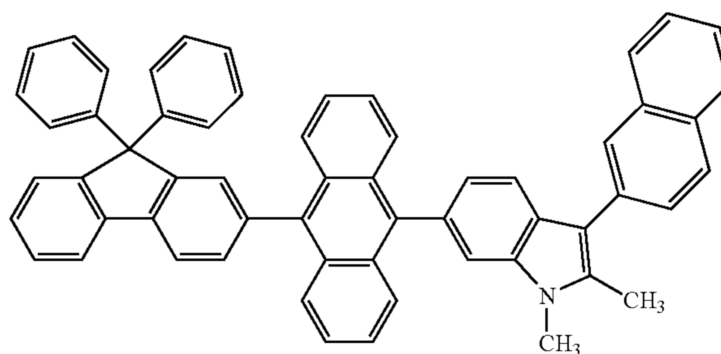
<Formula 71>
