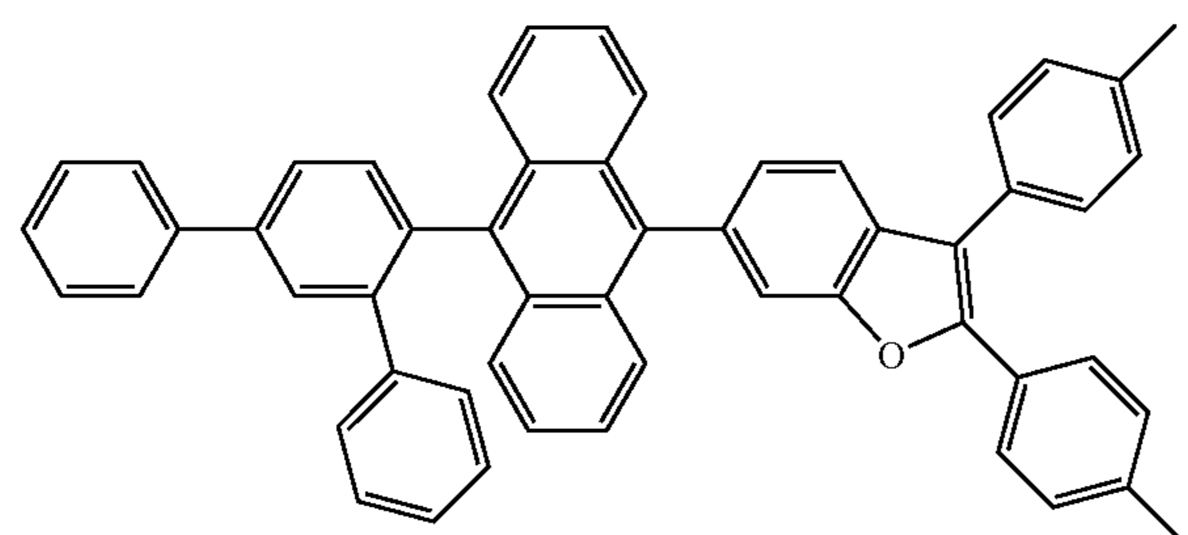
<Formula 49>
