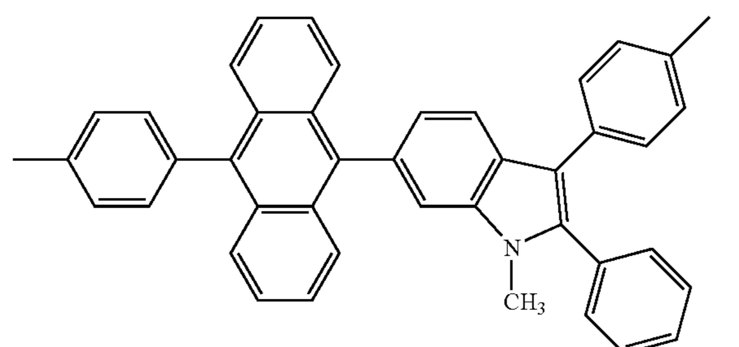
<Formula 55>
