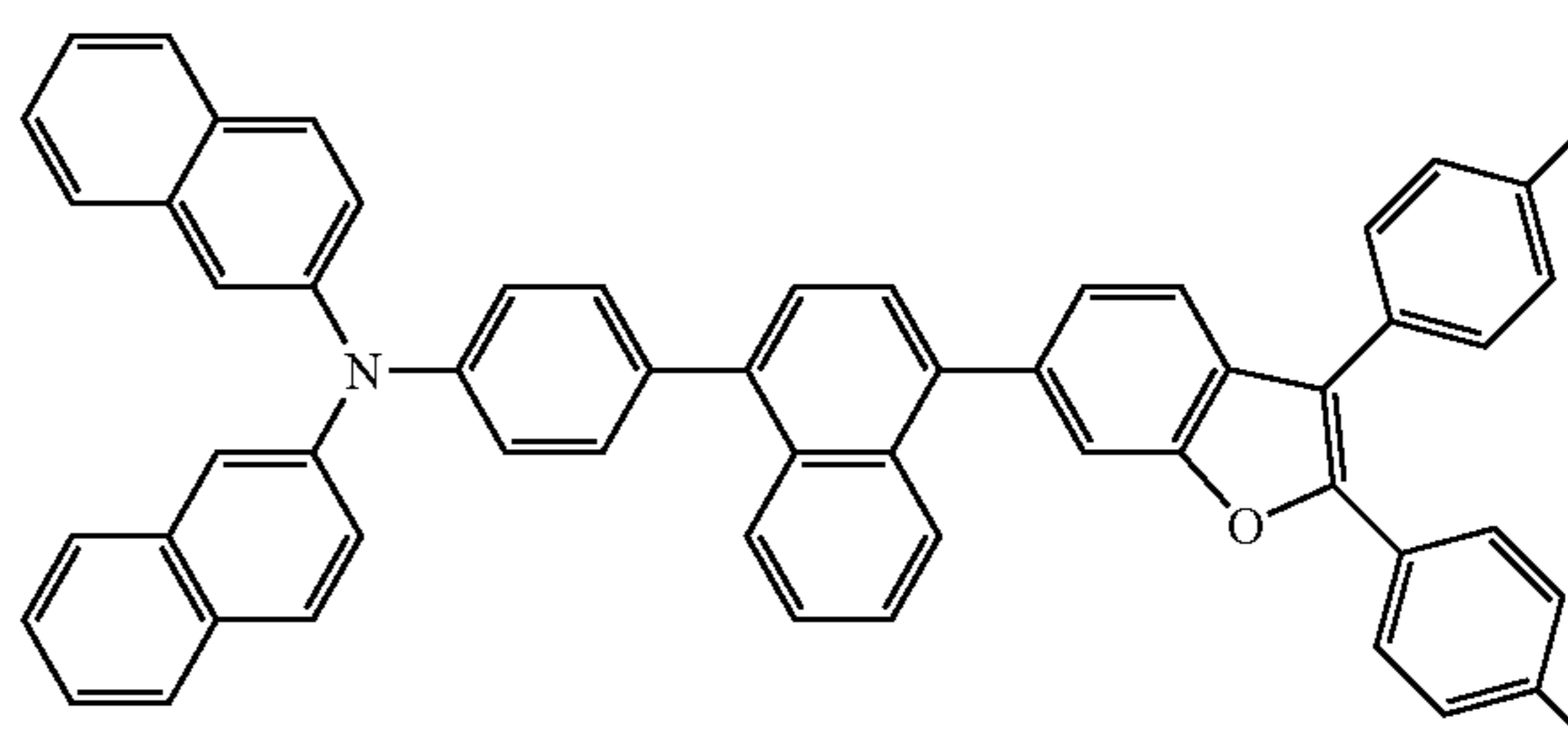
<Formula 54>
