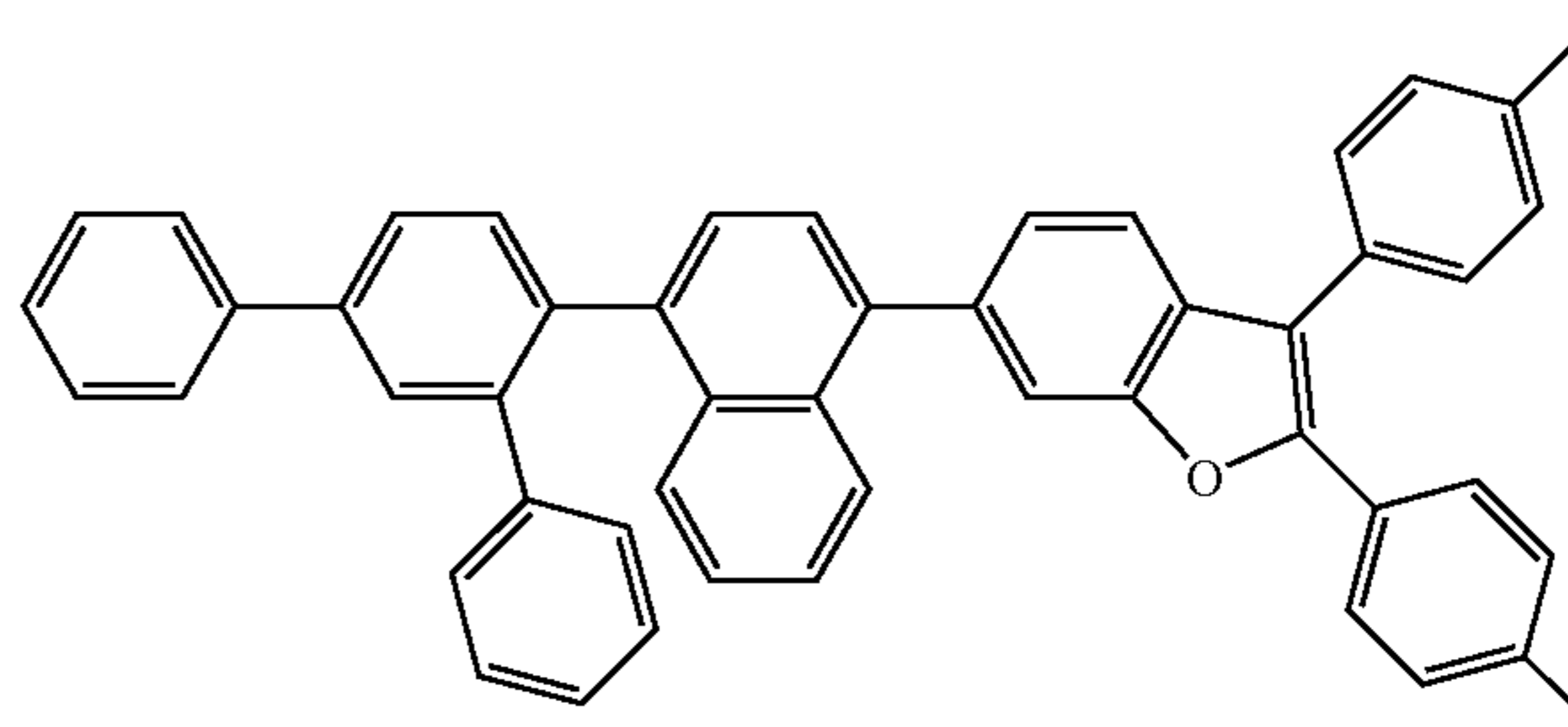
<Formula 52>
