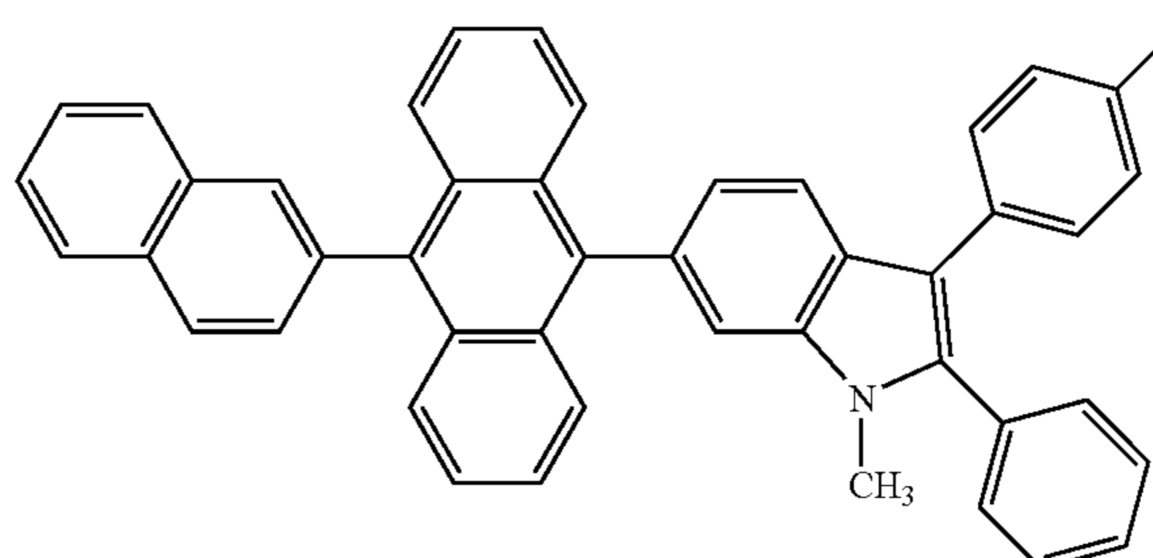
<Formula 56>
