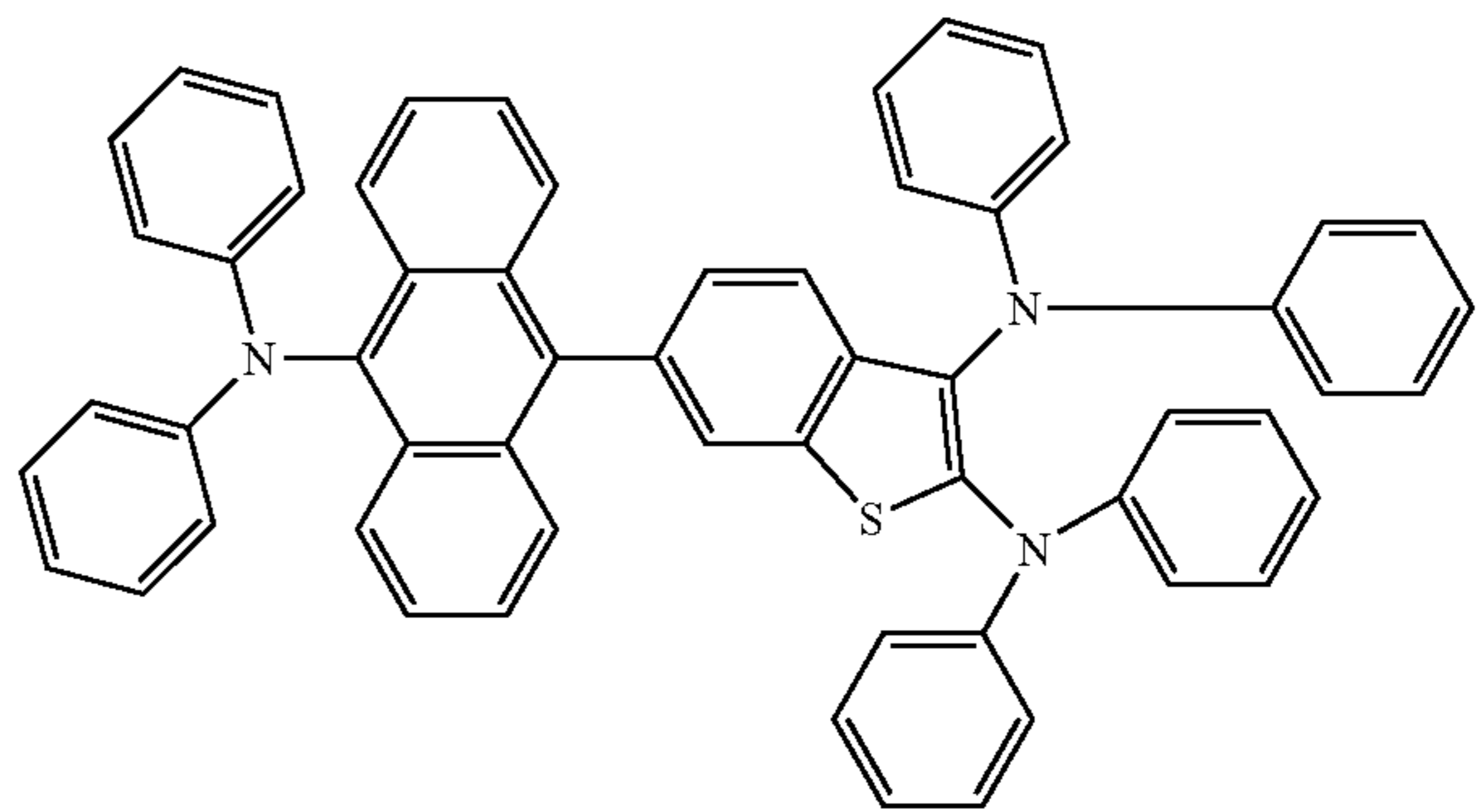
<Formula 12>
