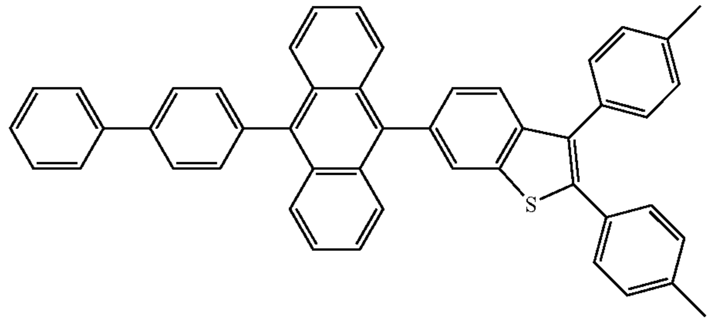
<Formula 9>
