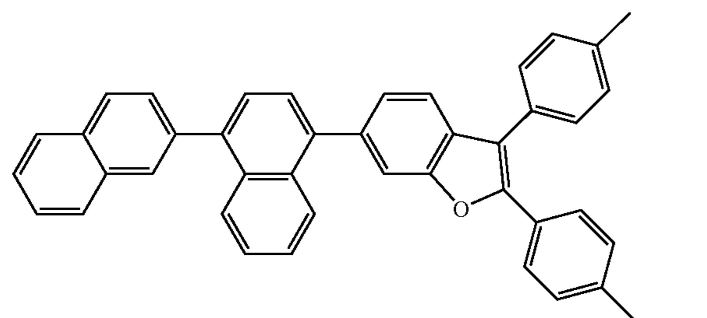
<Formula 51>
