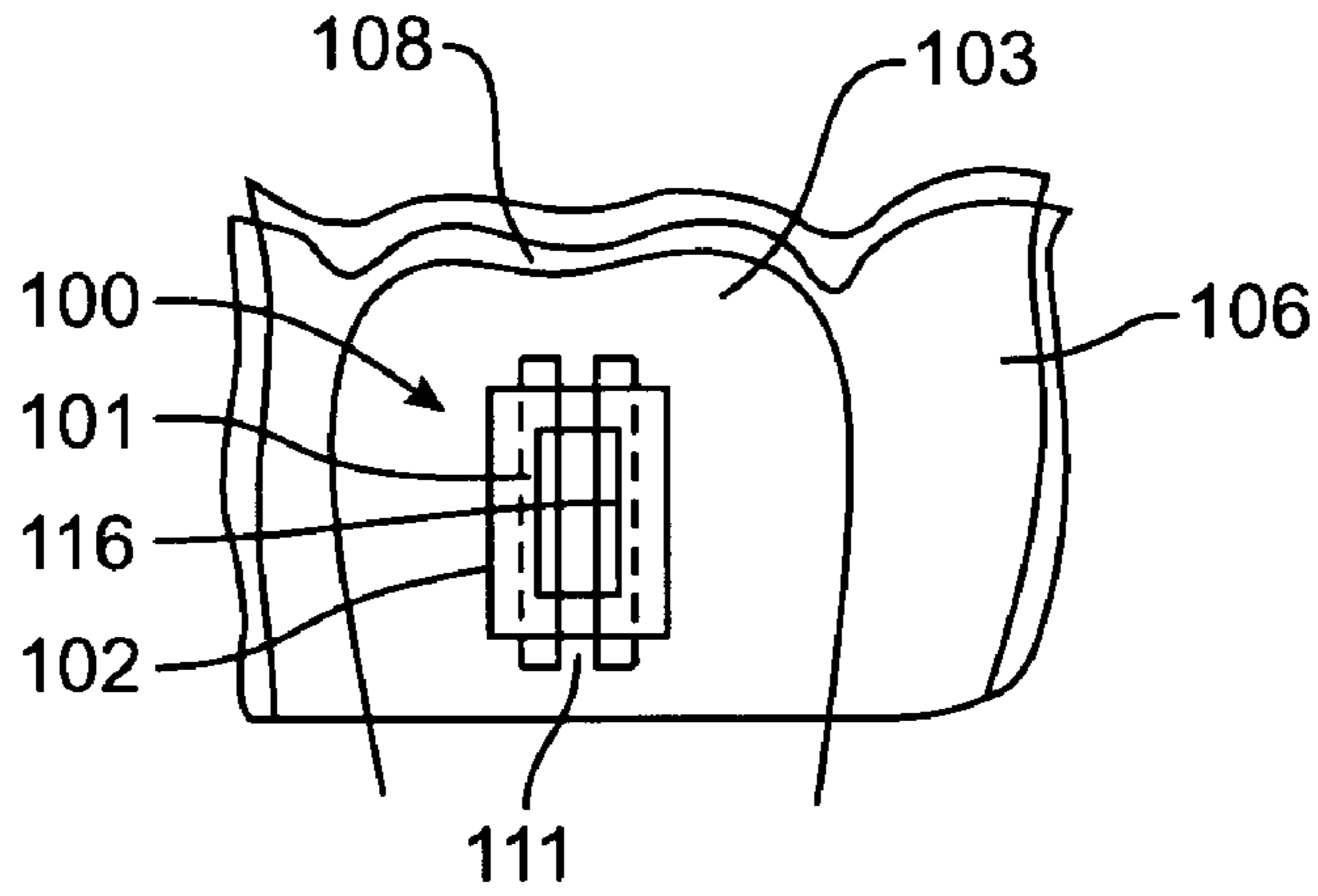
FIG. 4B
