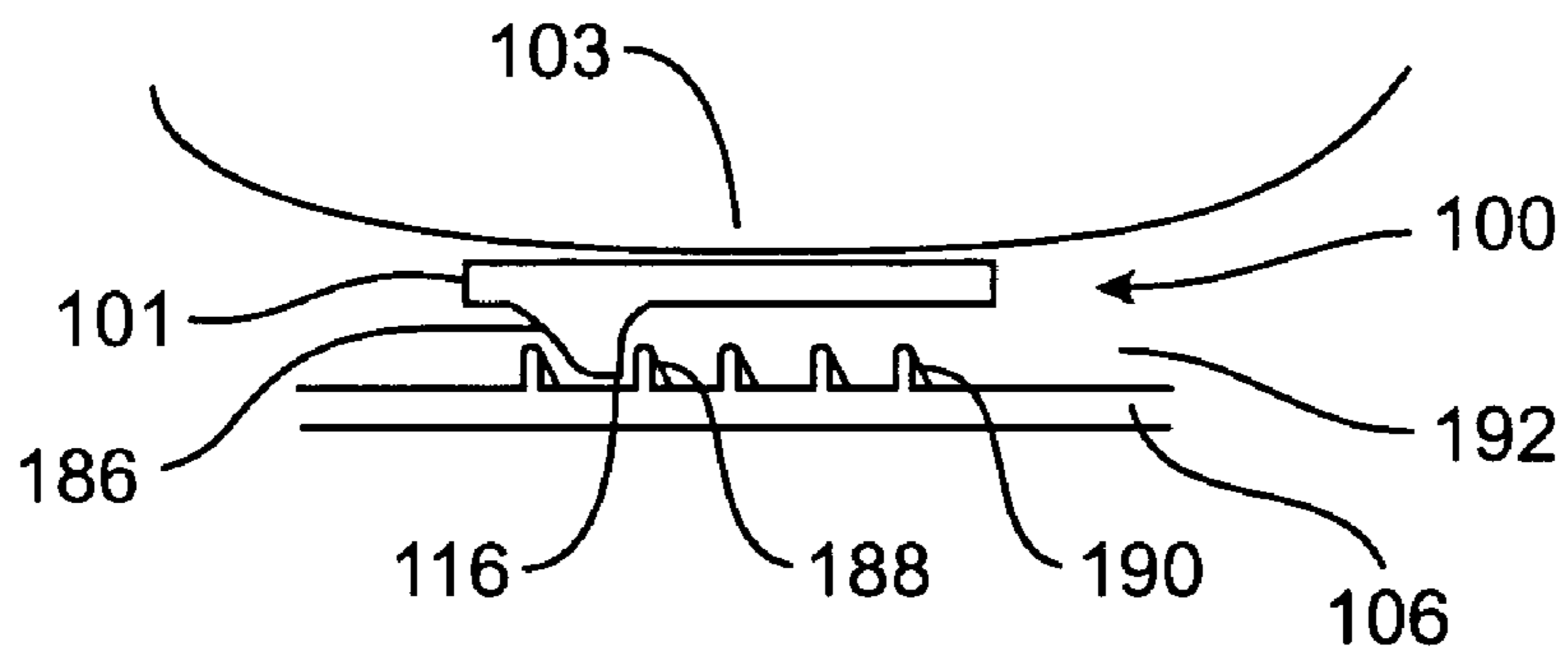
FIG. 15
