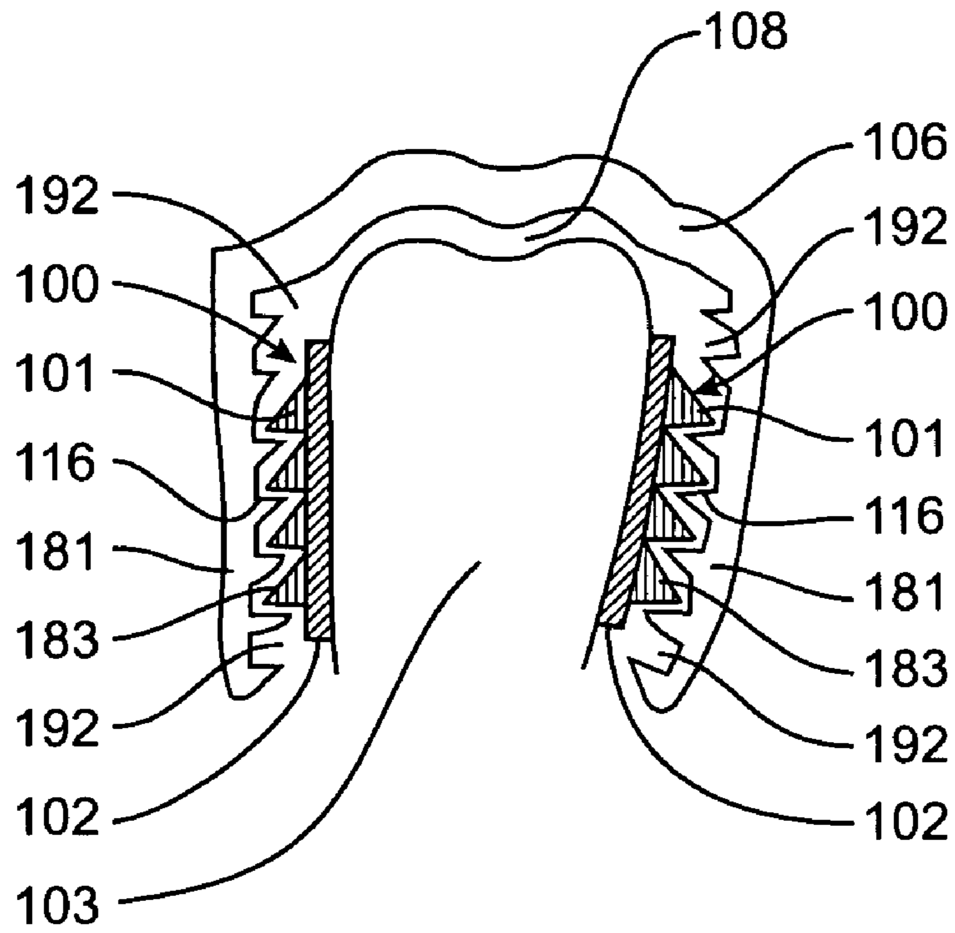
FIG. 13A
