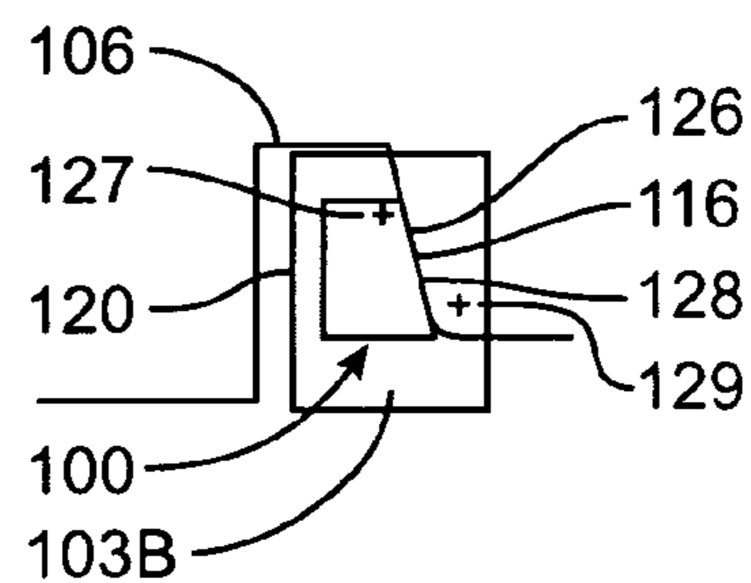
FIG. 6E
