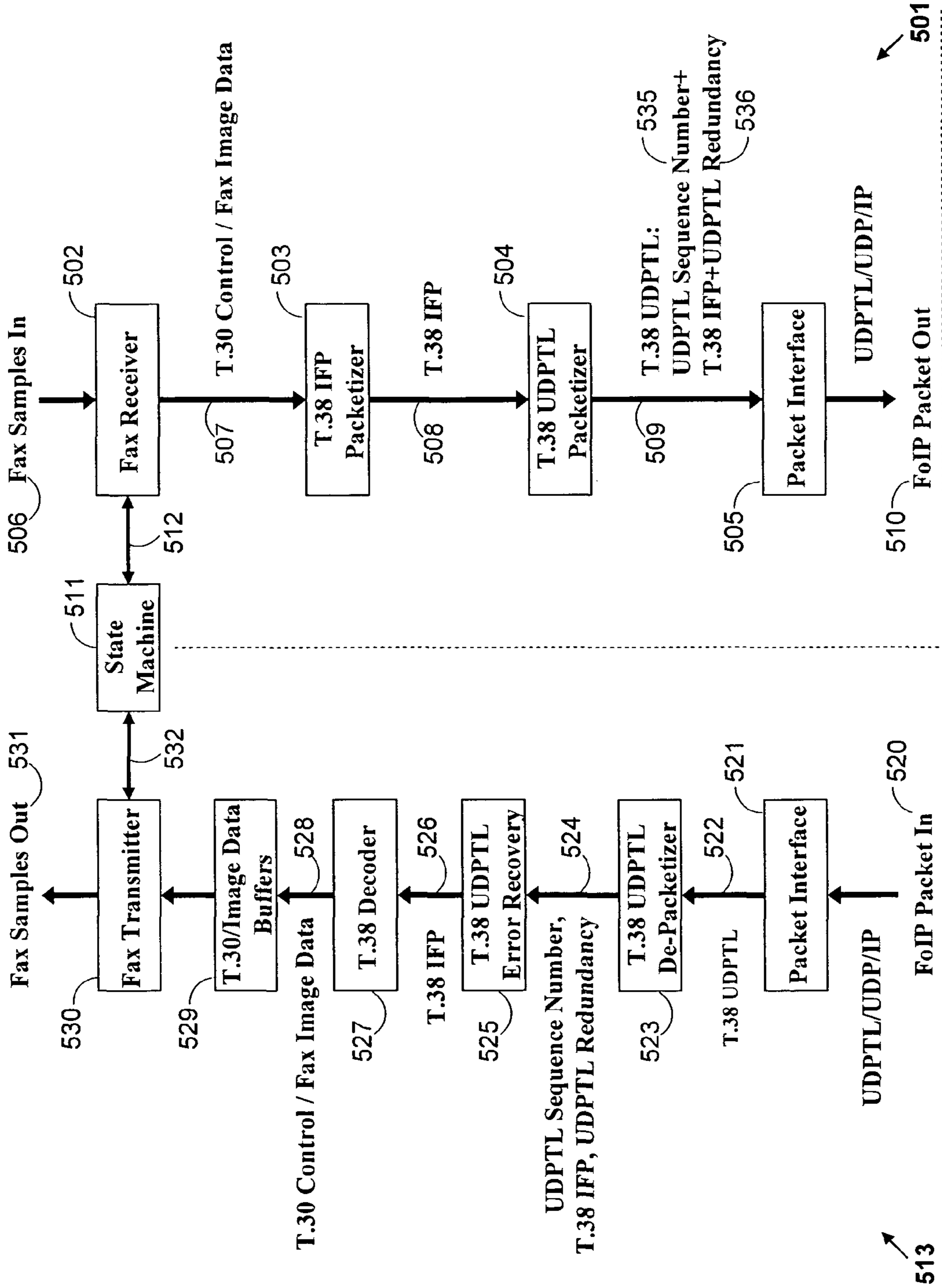
500 -- PRIOR ART -- Fig. 5a
