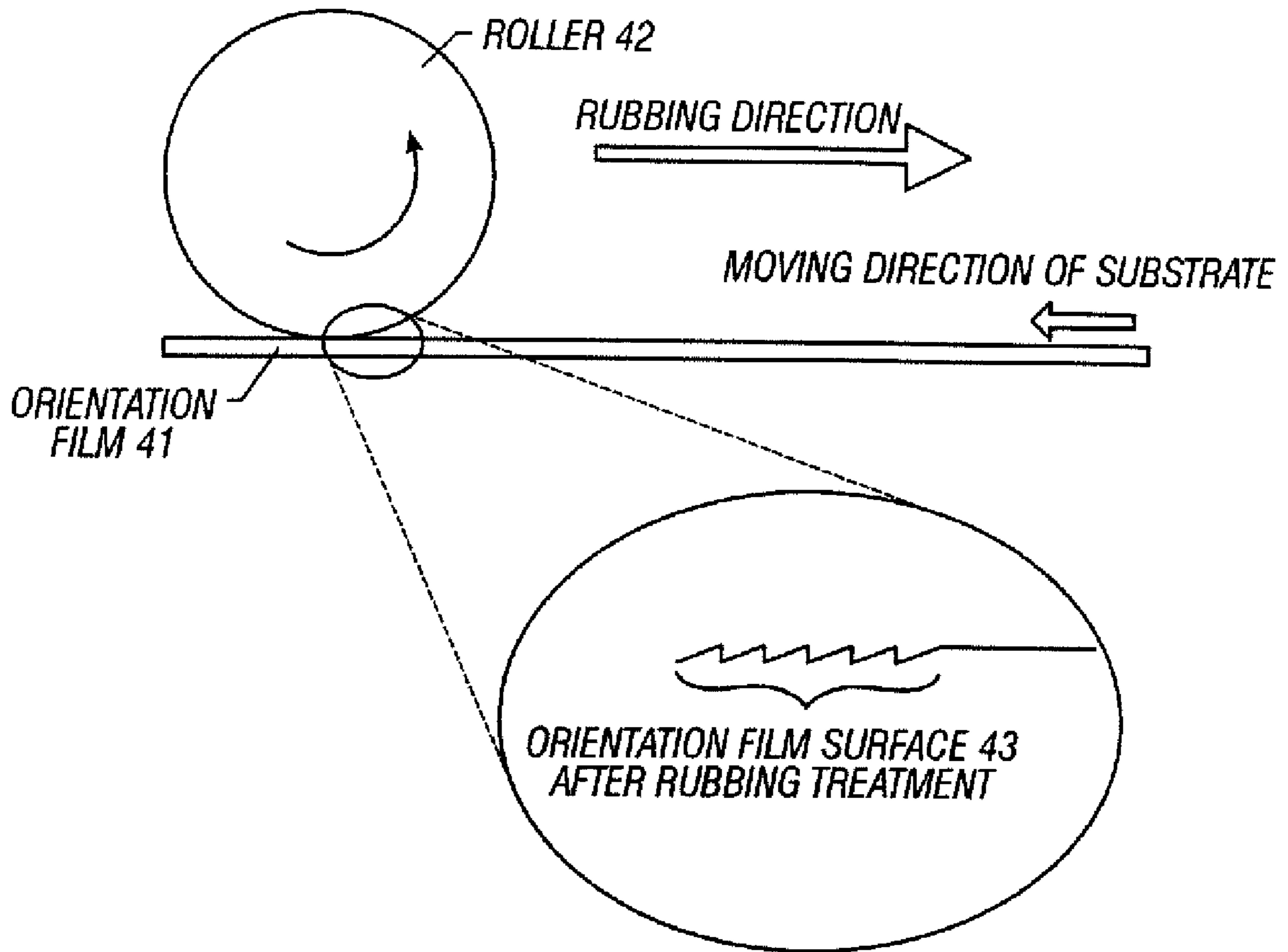
FIG. 10A
