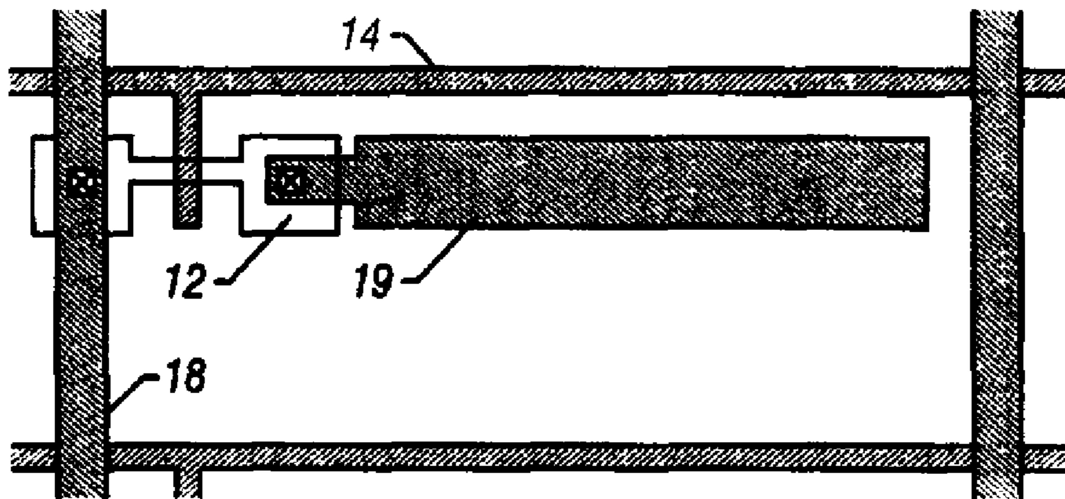
FIG. 2A
