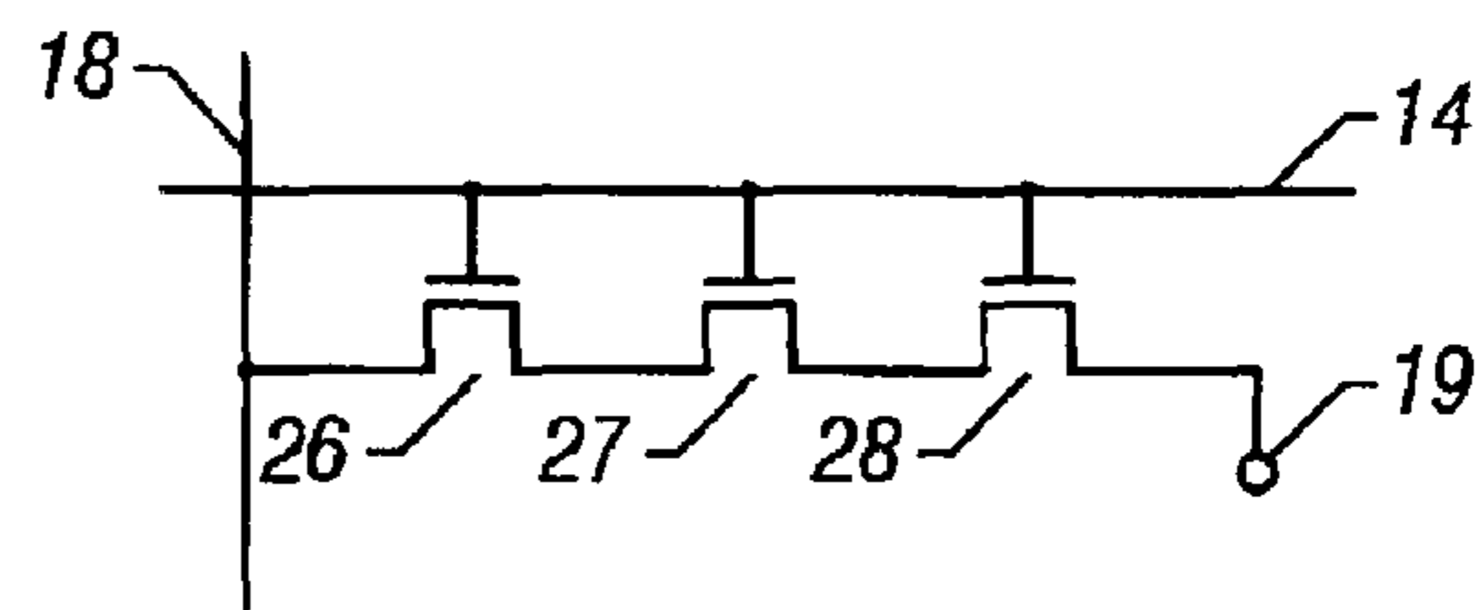
FIG. 7B
