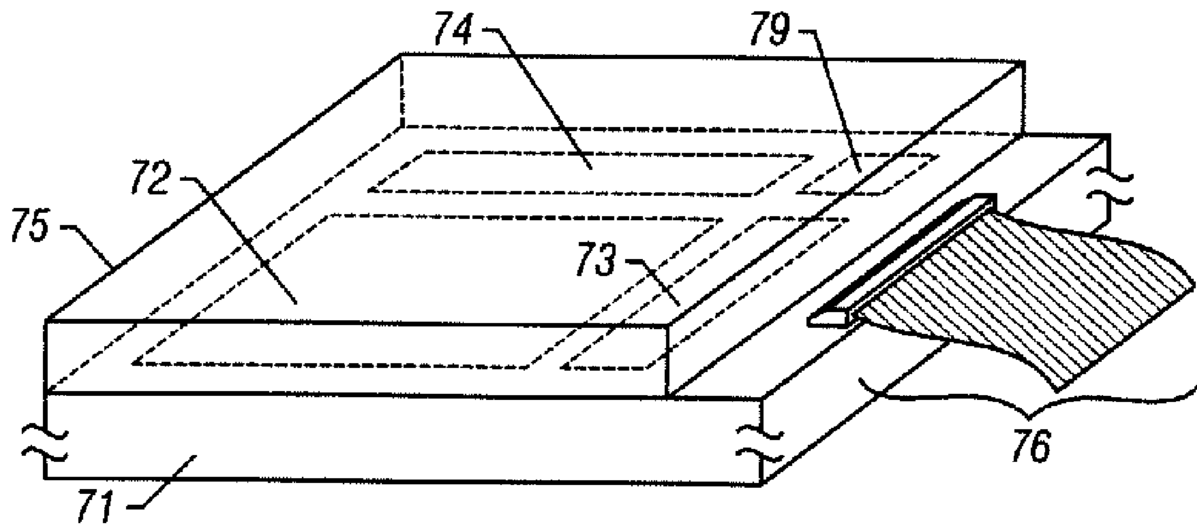
FIG. 12B
