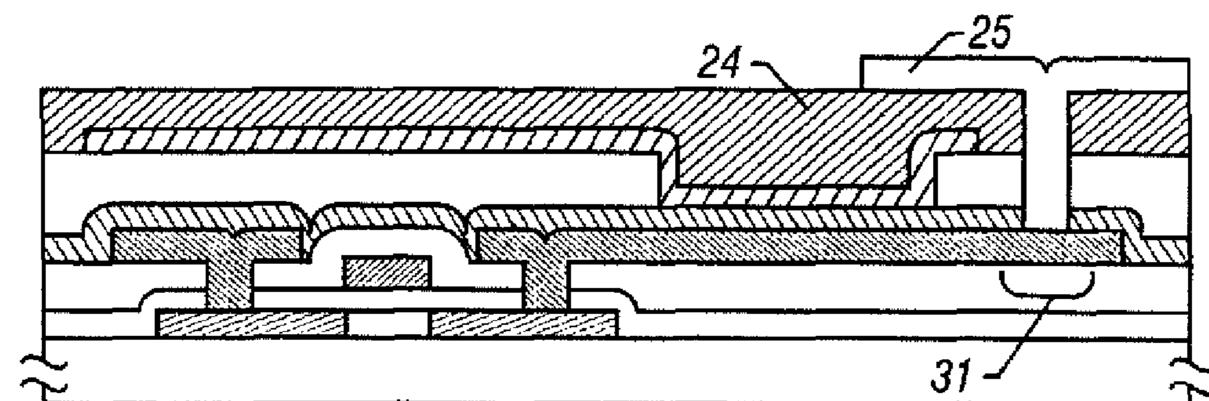
FIG. 3E
