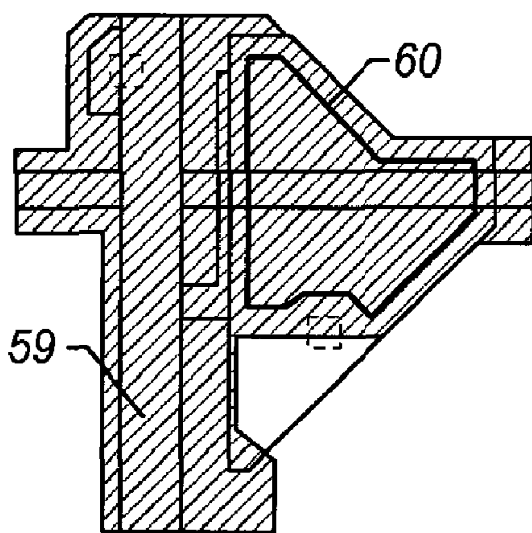
FIG. 11F
