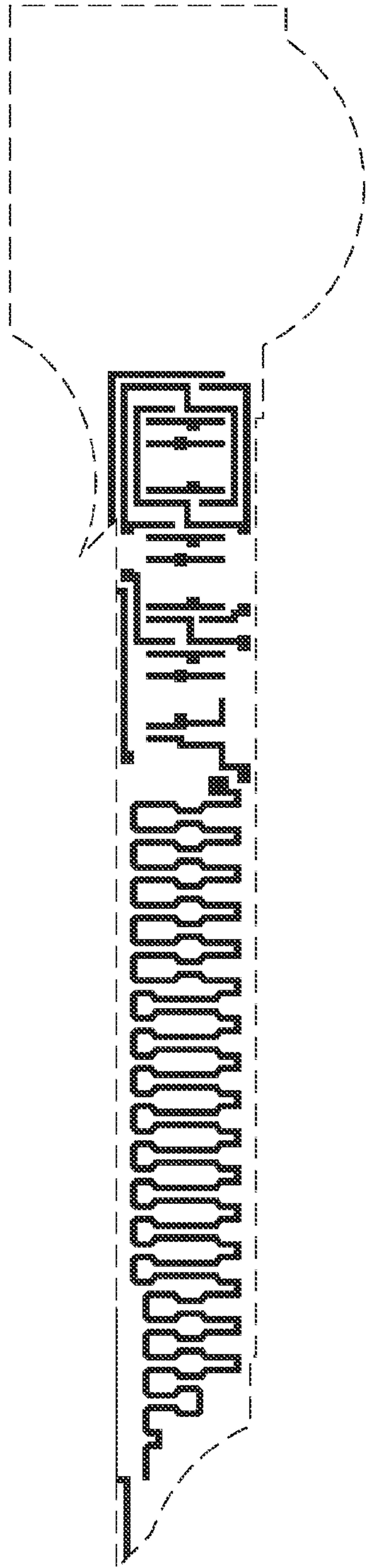
Poly mask
