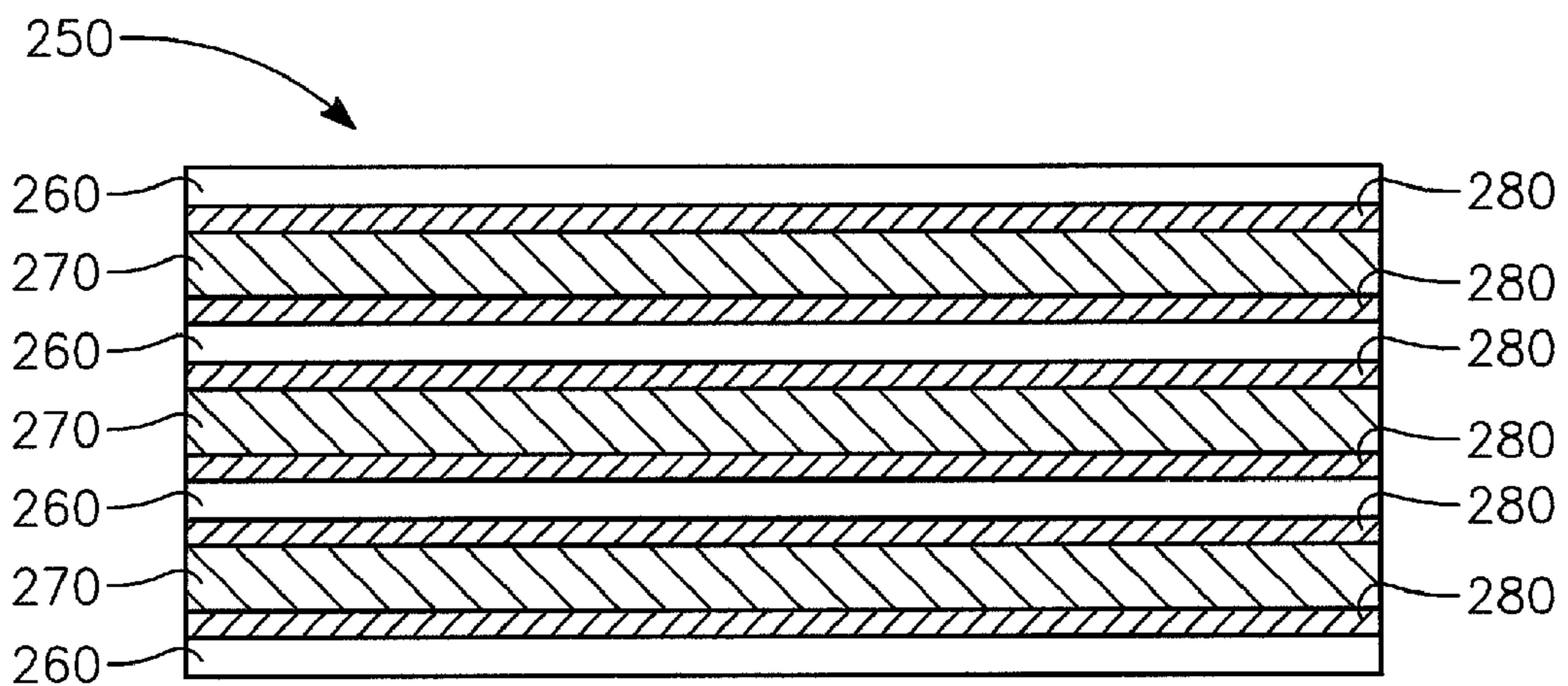
FIG. 2B
