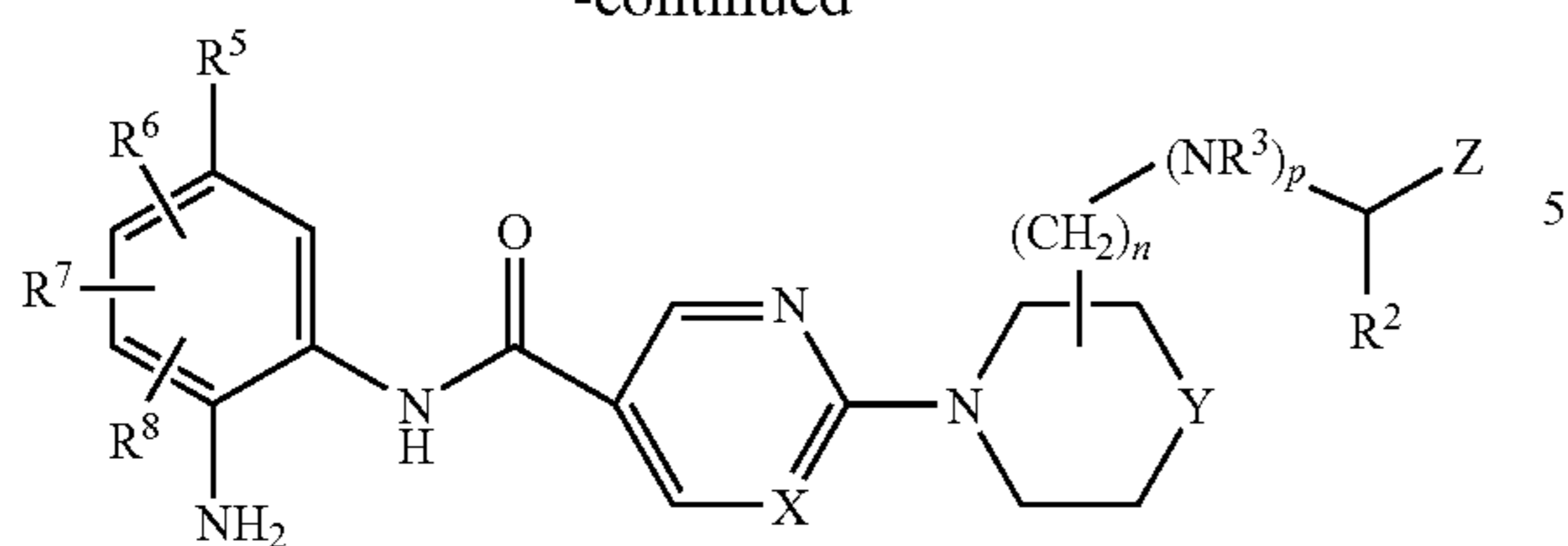
(I-b)
