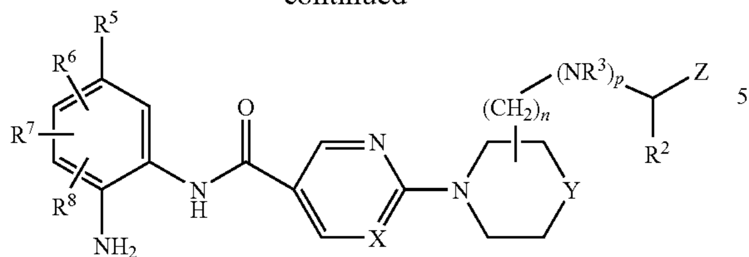
(I-b)
