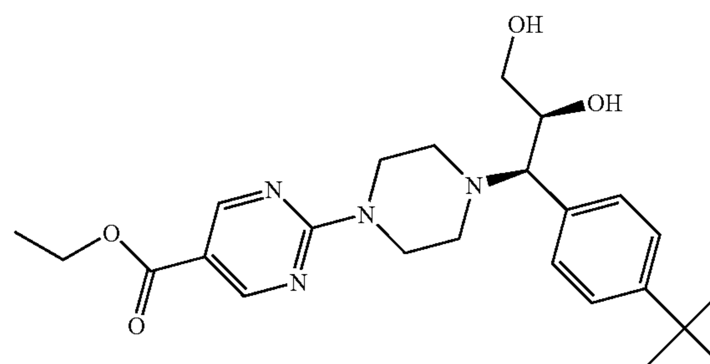
Enantiomer A
