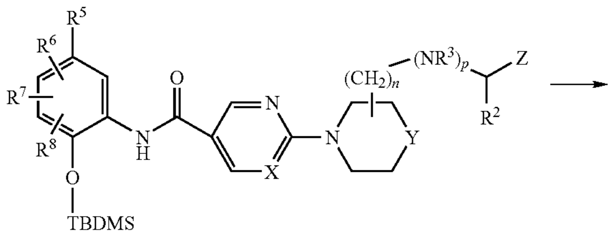
(V)
