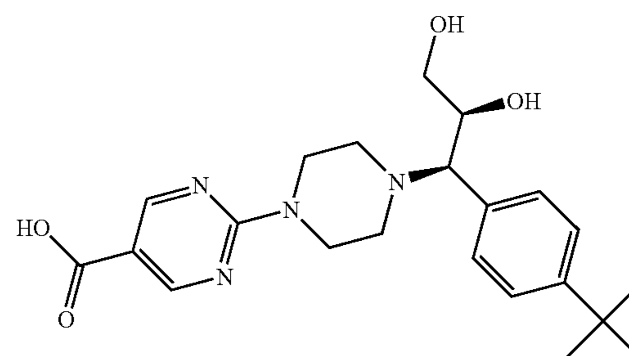
•2HCl•3Cl•3 Na
