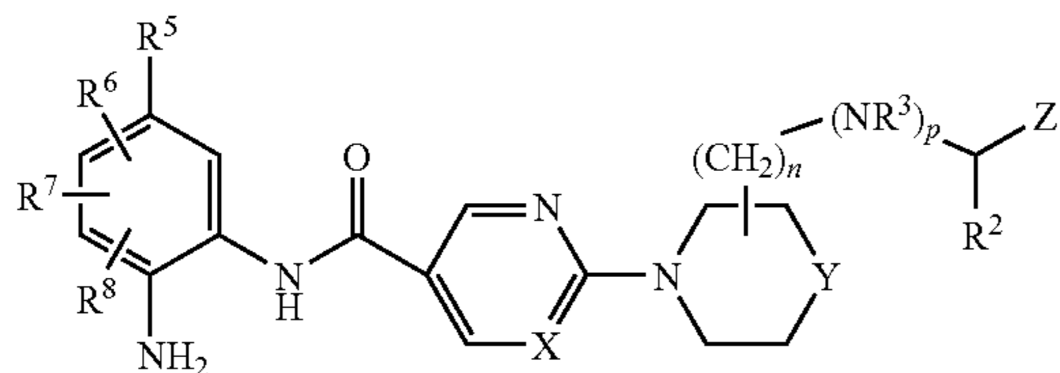
(I-b)
