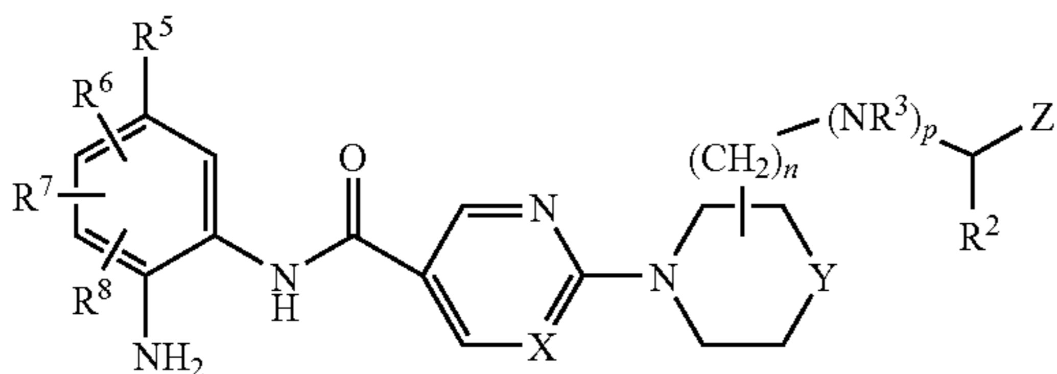
(I-b)
