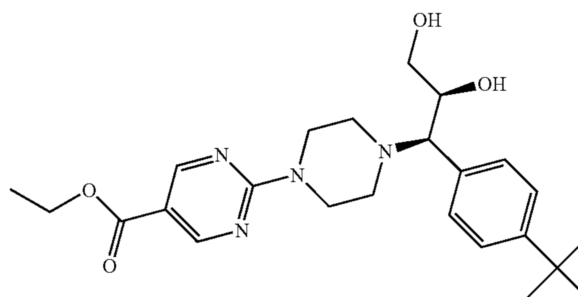
Enantiomer A
