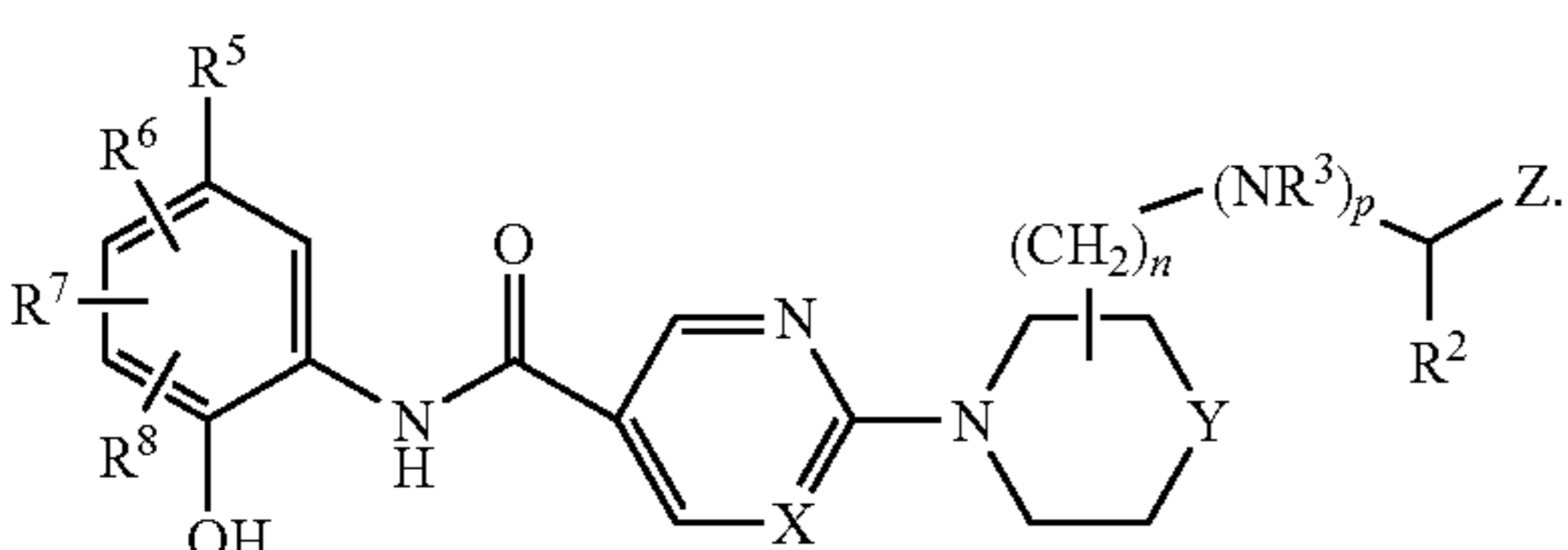
(I-c)
