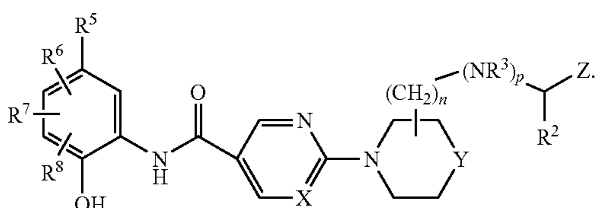
(I-c)
