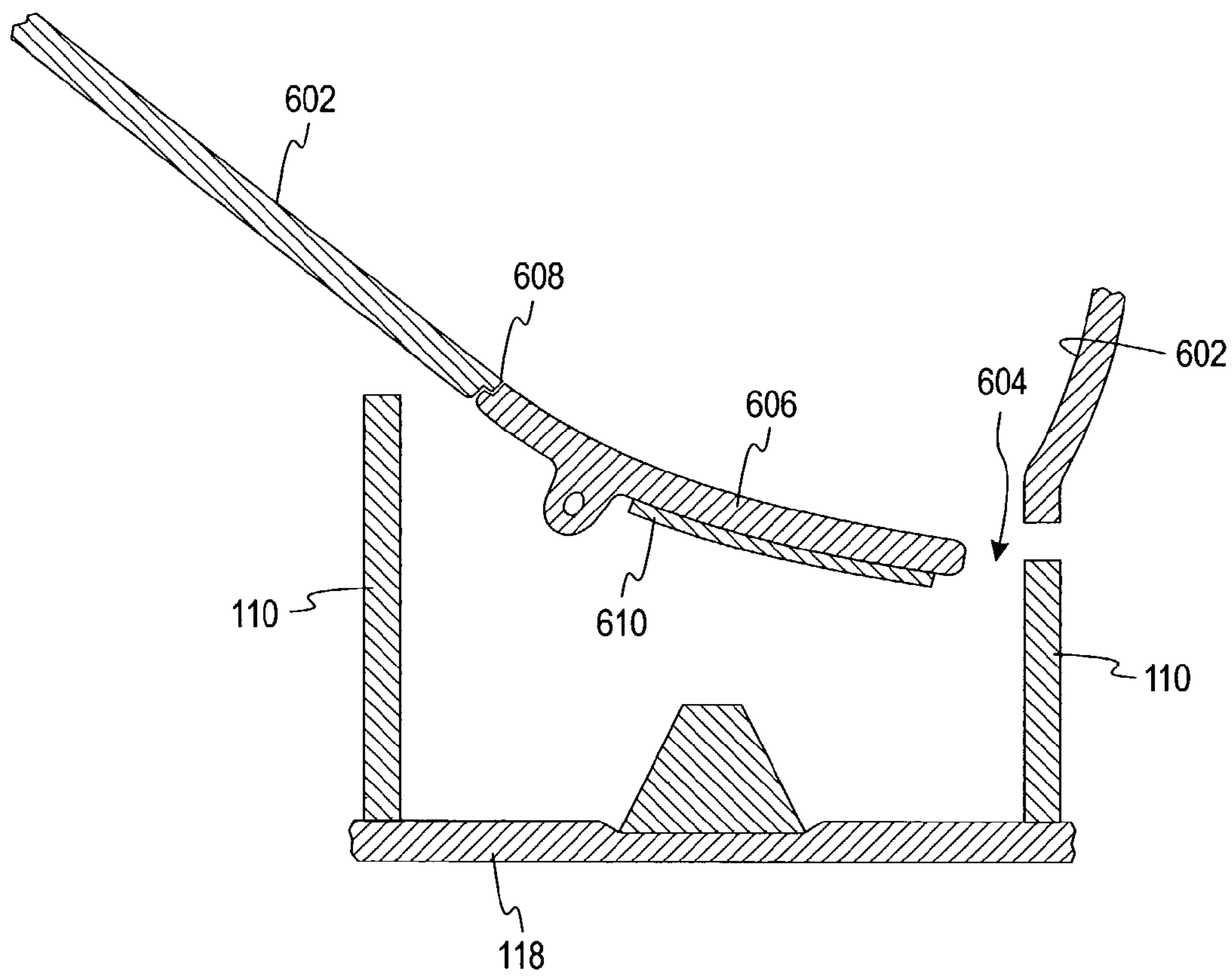
FIG. 13b
