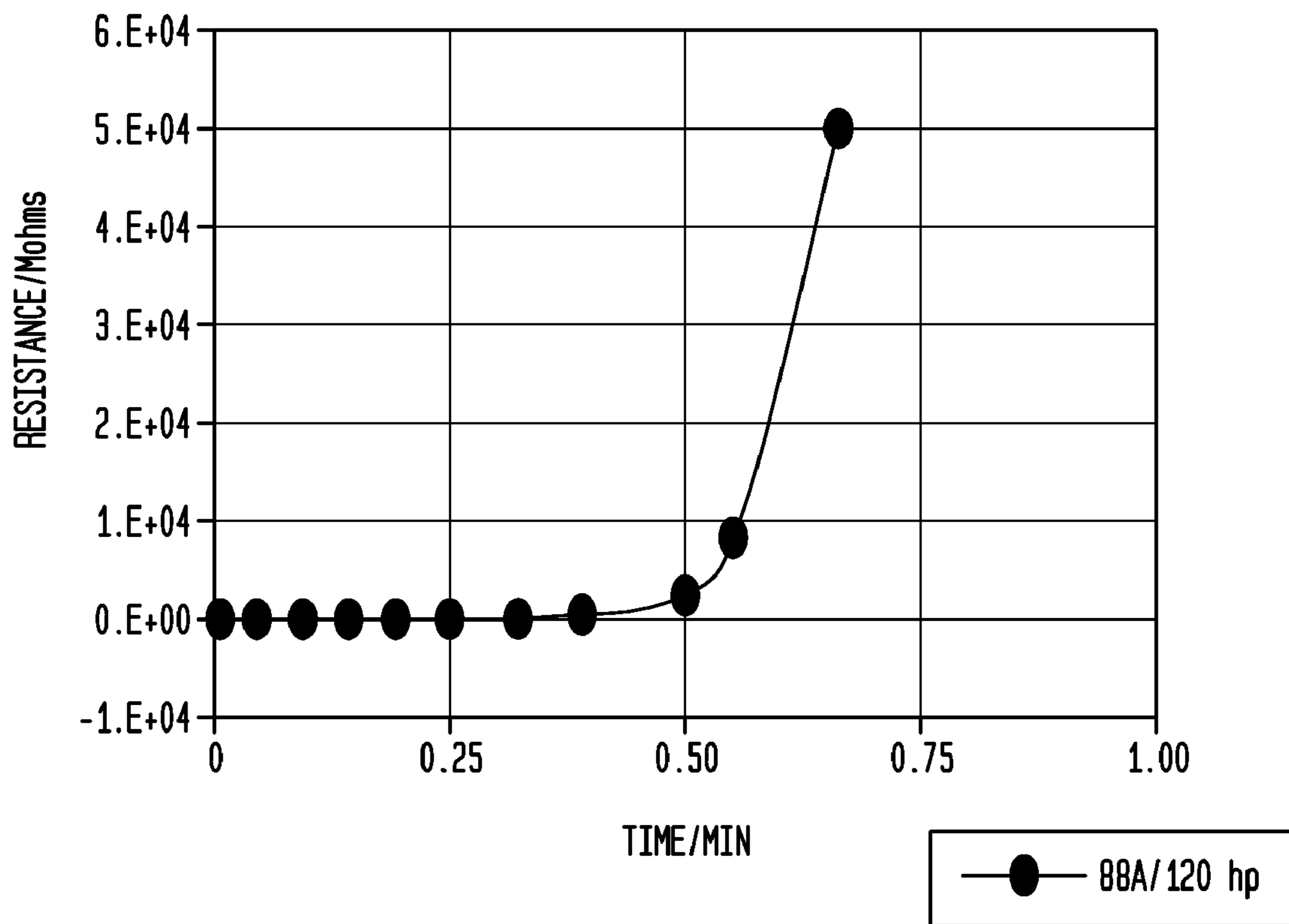
FIG. 14 W-b FLEXO INK - 88A - HANDPROOFER 1201pi
