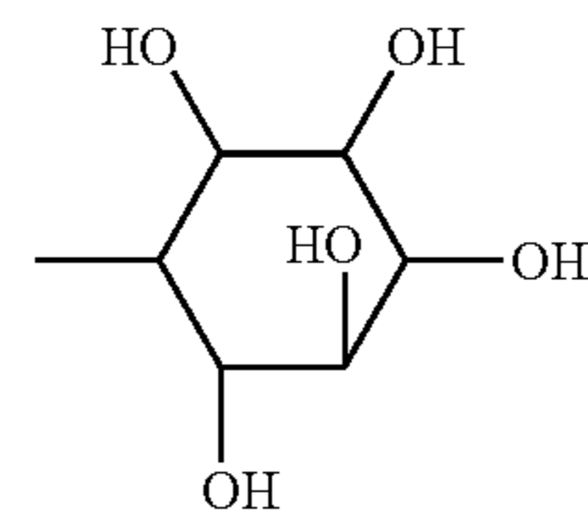
inositol
