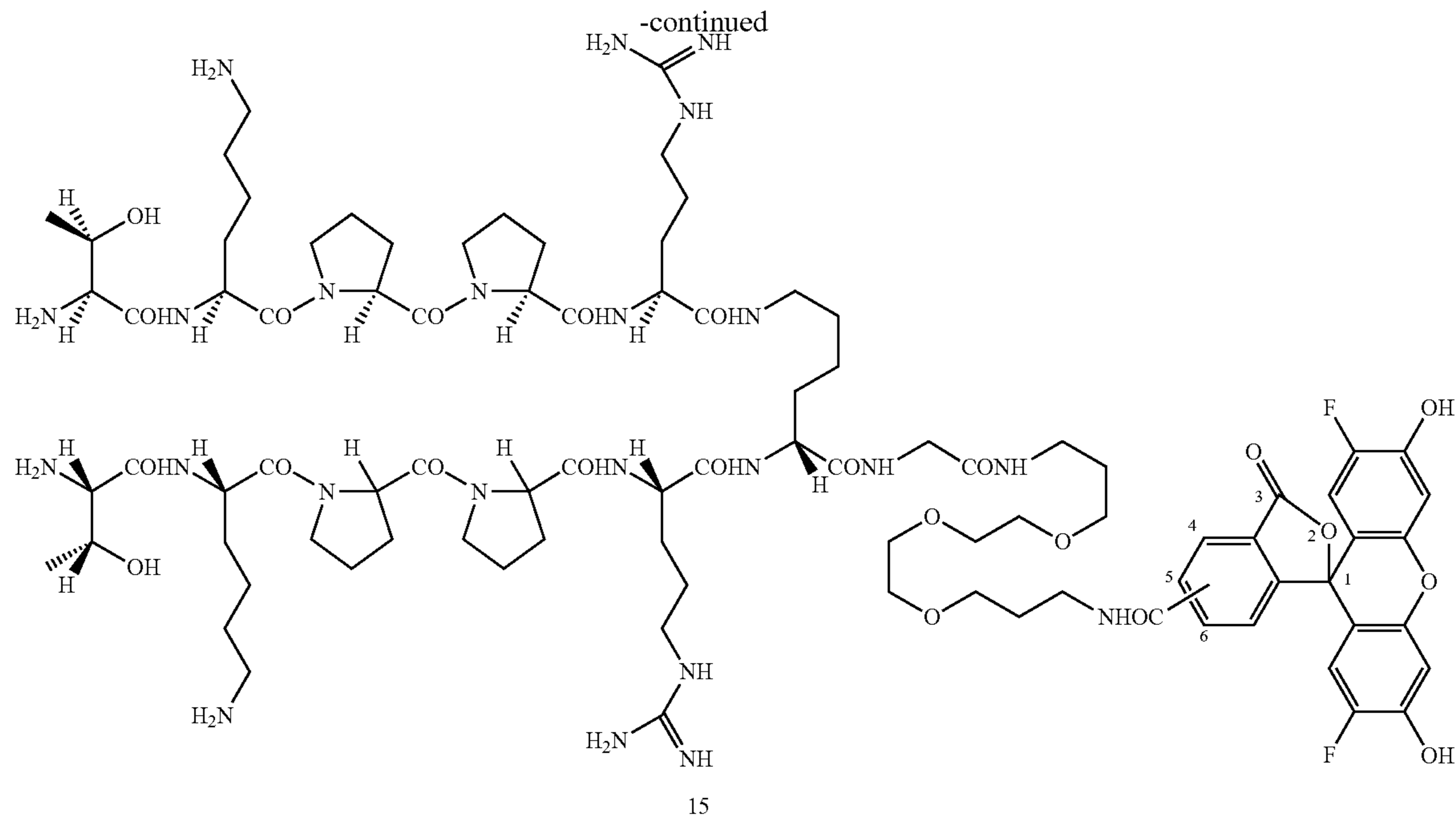
Thr-Lys-Pro-Pro-Arg-Lys(Arg-Pro-Pro-Lys-Thr)-Gly- TTDA-OG (SEQ ID NO:7) TTDA = 4,7,10-Trioxa-1,13-TridecaneDiame
