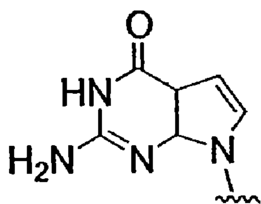
N9-(7-deaza-G)
