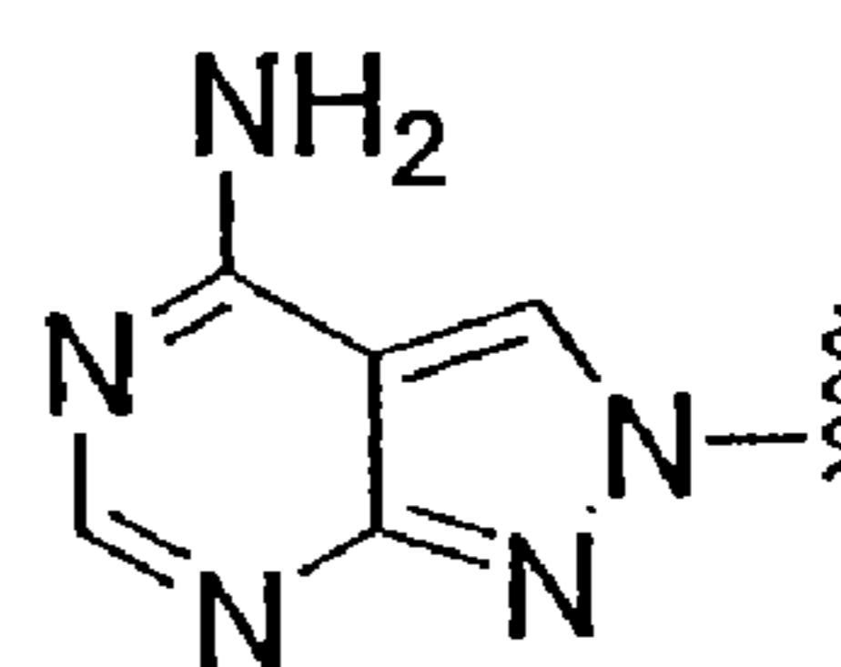
N8-(7-deaza-8-aza-A)
